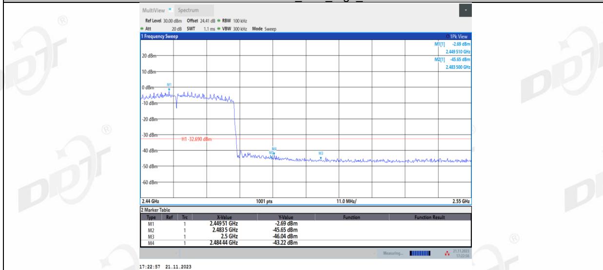
11AX40MIMO_Ant2_High_2452
