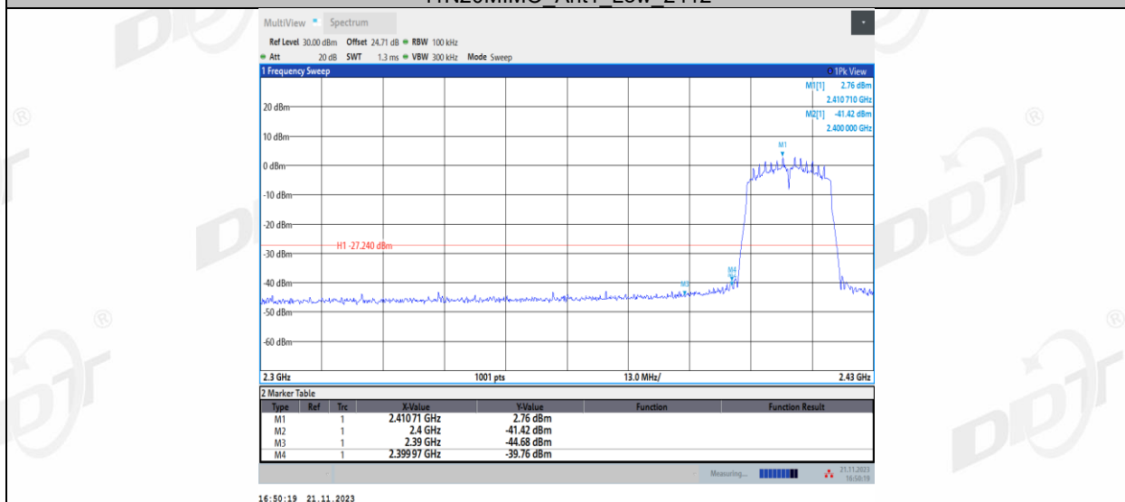
11N20MIMO_Ant2_Low_2412
