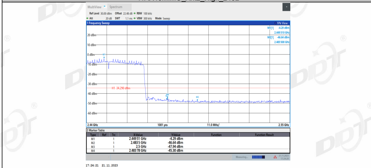
11AX40MIMO_Ant2_High_2452
