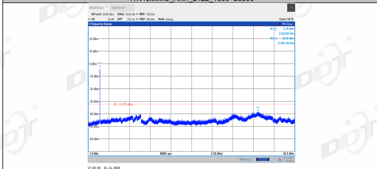
11N40MIMO_Ant2_2422_0~Reference
