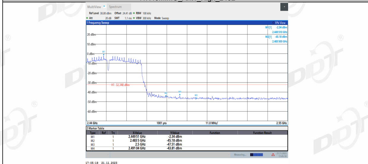
11N40MIMO_Ant2_High_2452
