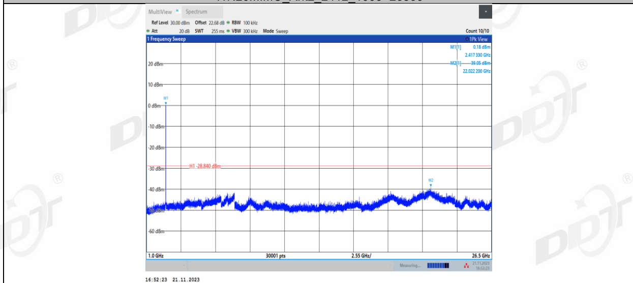
11N20MIMO_Ant1_2437_0~Reference
