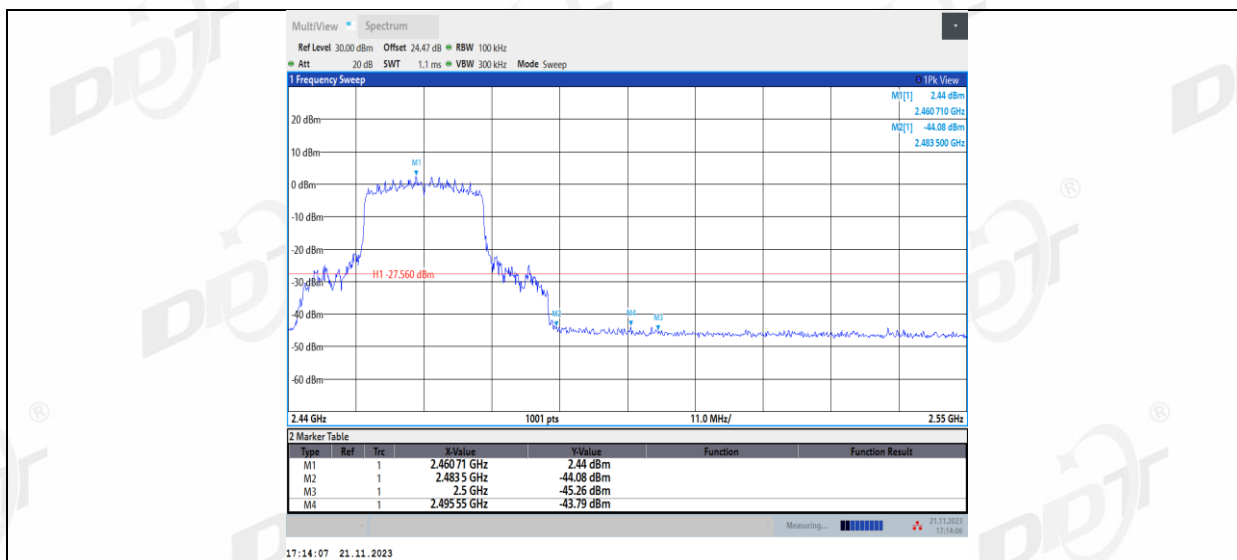
11AX20MIMO_Ant2_High_2462
