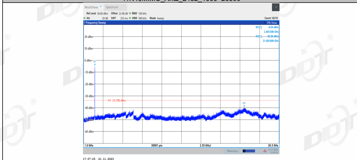
11AX20MIMO_Ant1_2412_0~Reference
