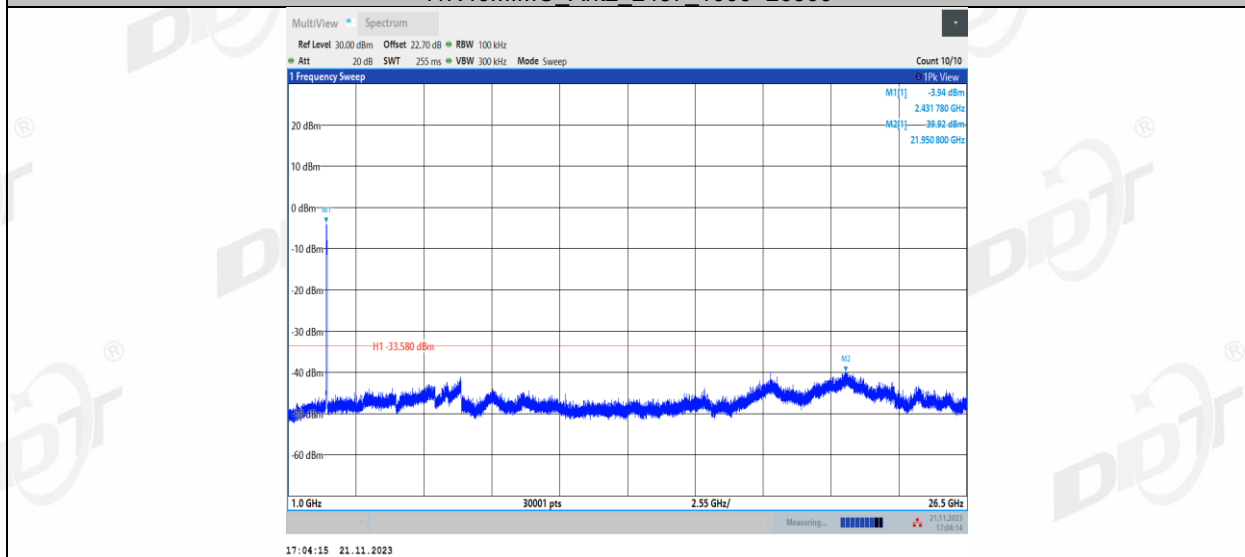
11N40MIMO_Ant1_2452_0~Reference
