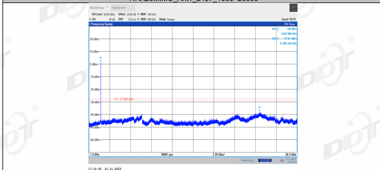
11AX20MIMO_Ant2_2437_0~Reference
