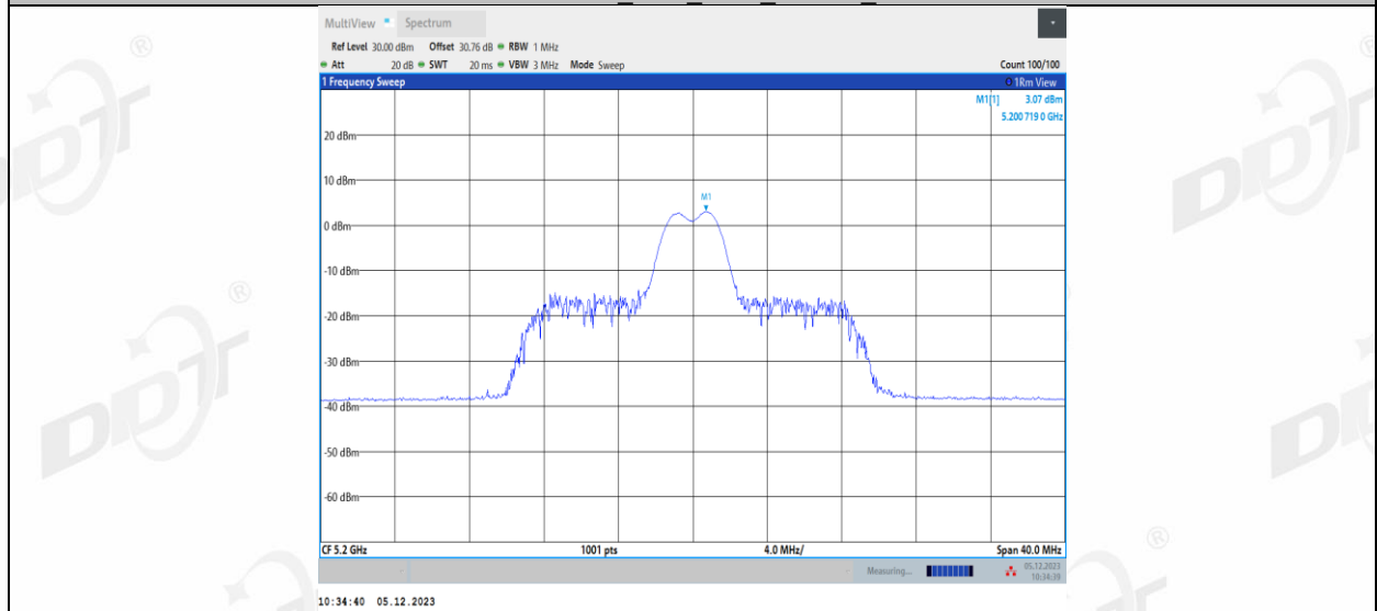
11AX20MIMO_Ant1_5200_26Tone_RU8
