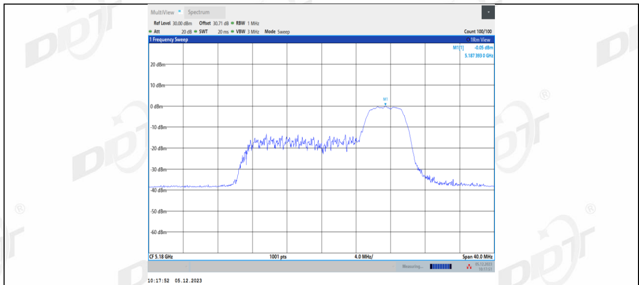
11AX20MIMO_Ant2_5180_106Tone_RU53
