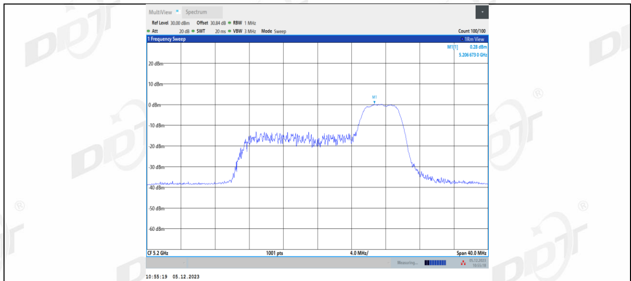
11AX20MIMO_Ant2_5200_106Tone_RU53
