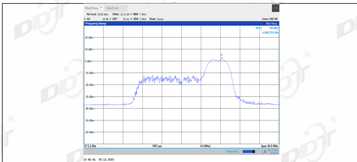
11AX20MIMO_Ant1_5200_106Tone_RU53
