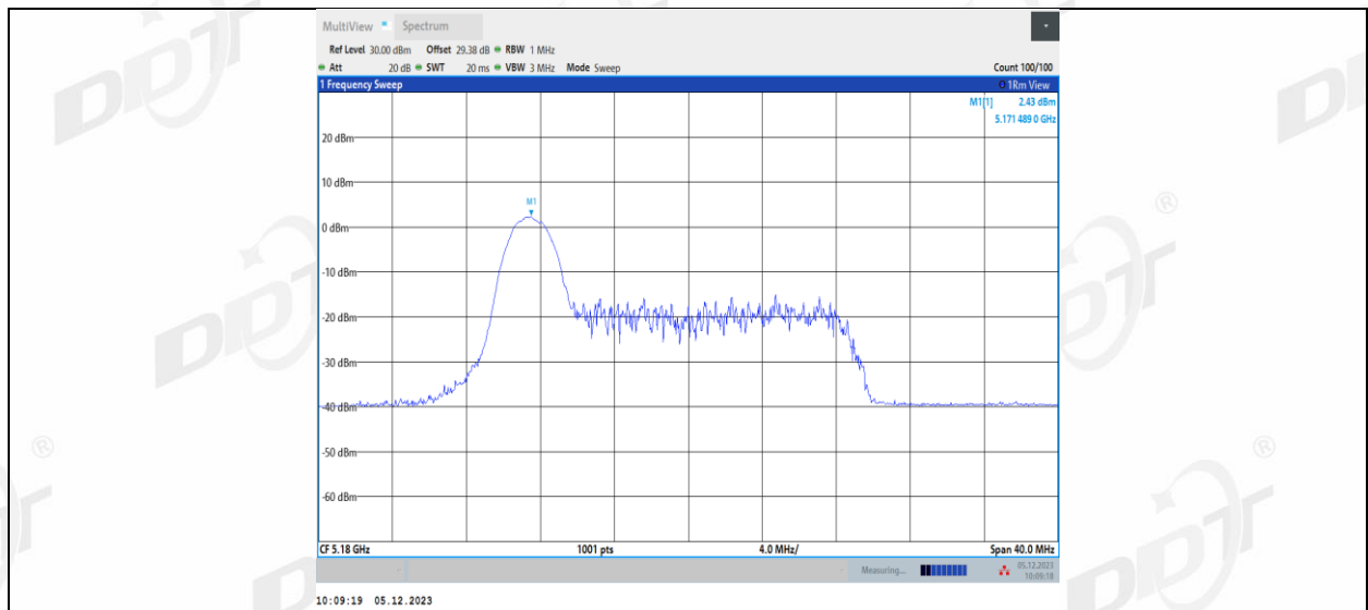
11AX20MIMO_Ant2_5180_26Tone_RU4
