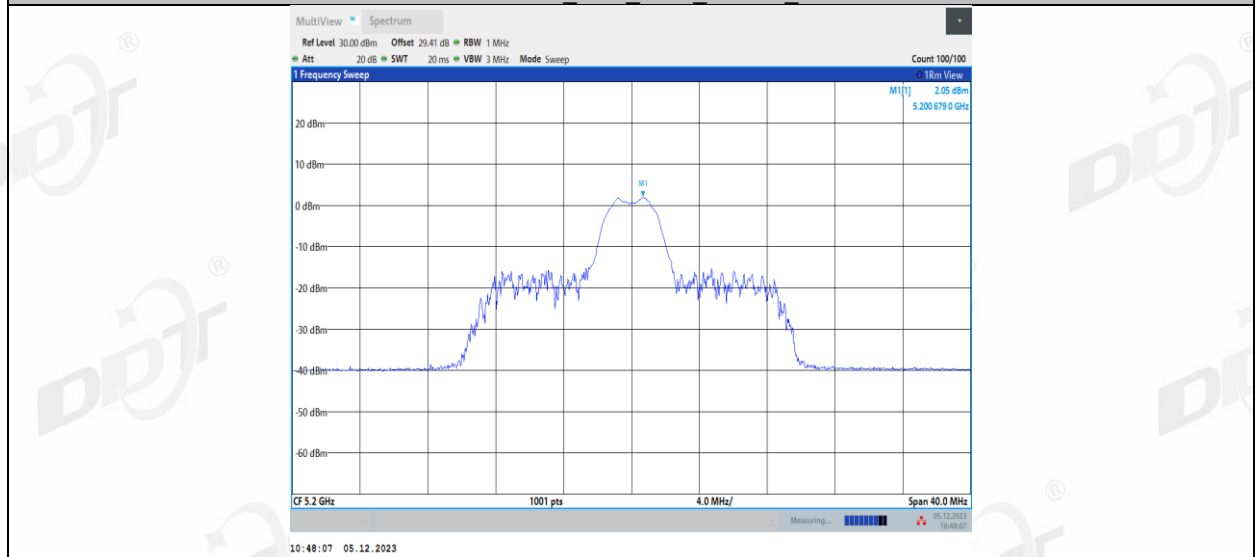
11AX20MIMO_Ant2_5200_26Tone_RU8
