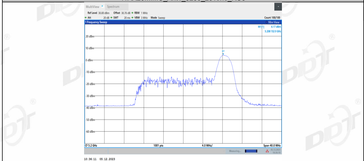
11AX20MIMO_Ant1_5200_52Tone_RU37
