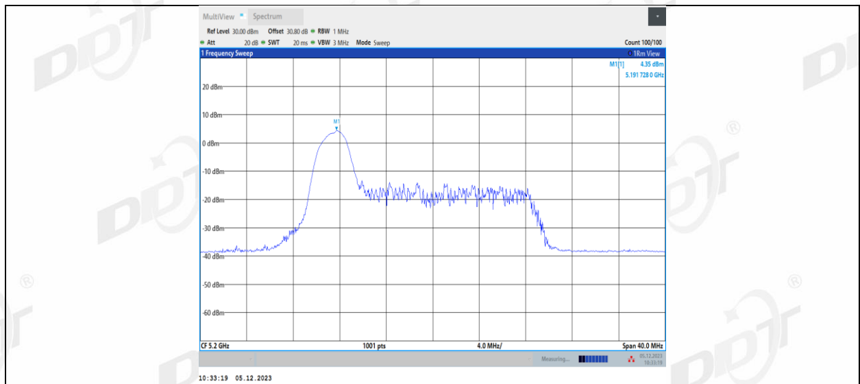
11AX20MIMO_Ant1_5200_26Tone_RU4
