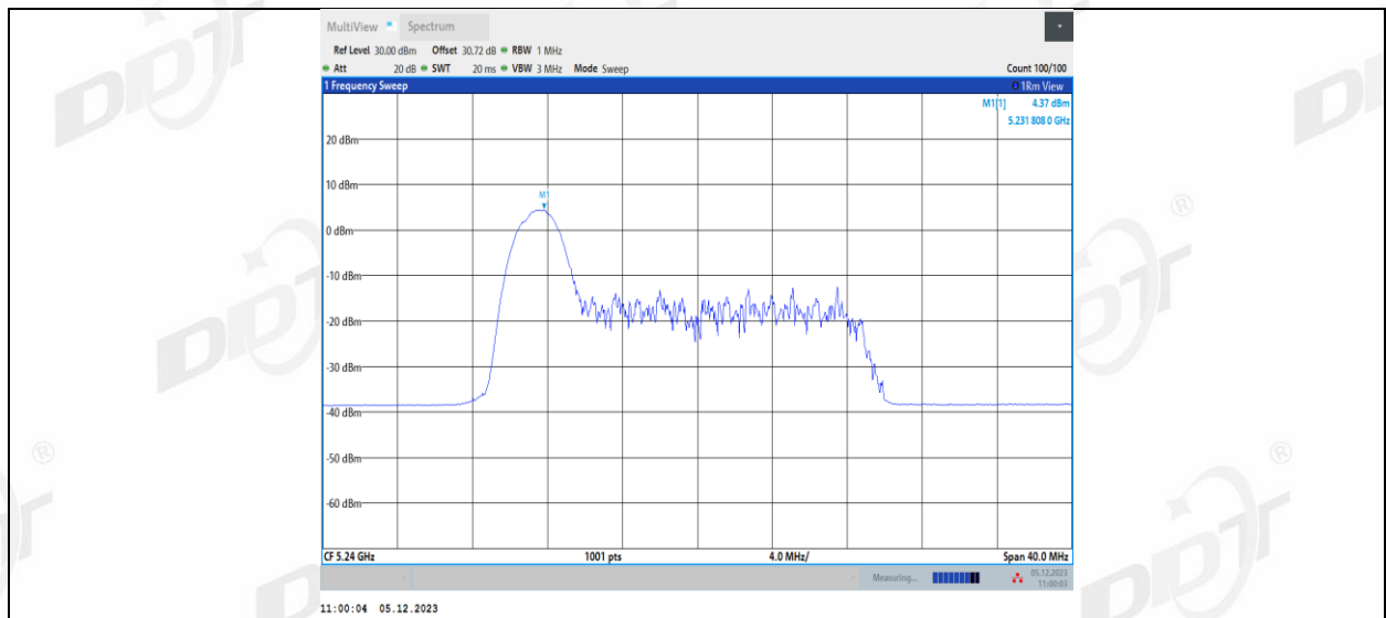
11AX20MIMO_Ant1_5240_26Tone_RU4
