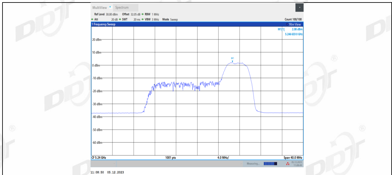
11AX20MIMO_Ant1_5240_106Tone_RU53
