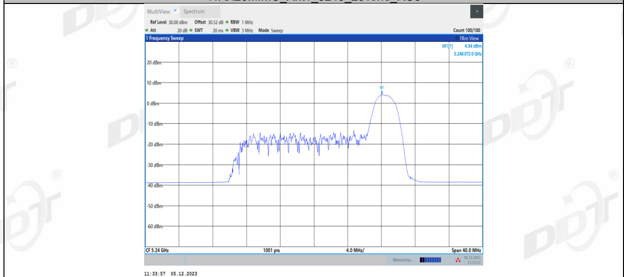
11AX20MIMO_Ant1_5240_52Tone_RU37
