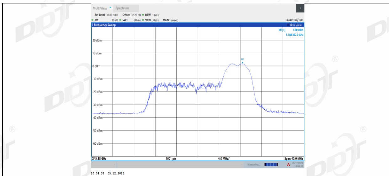
11AX20MIMO_Ant1_5180_106Tone_RU53
