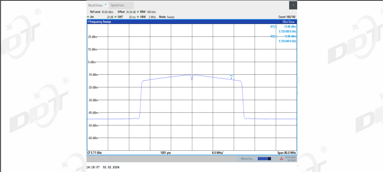
11AX40MIMO_Ant2_5710_UNII-3
