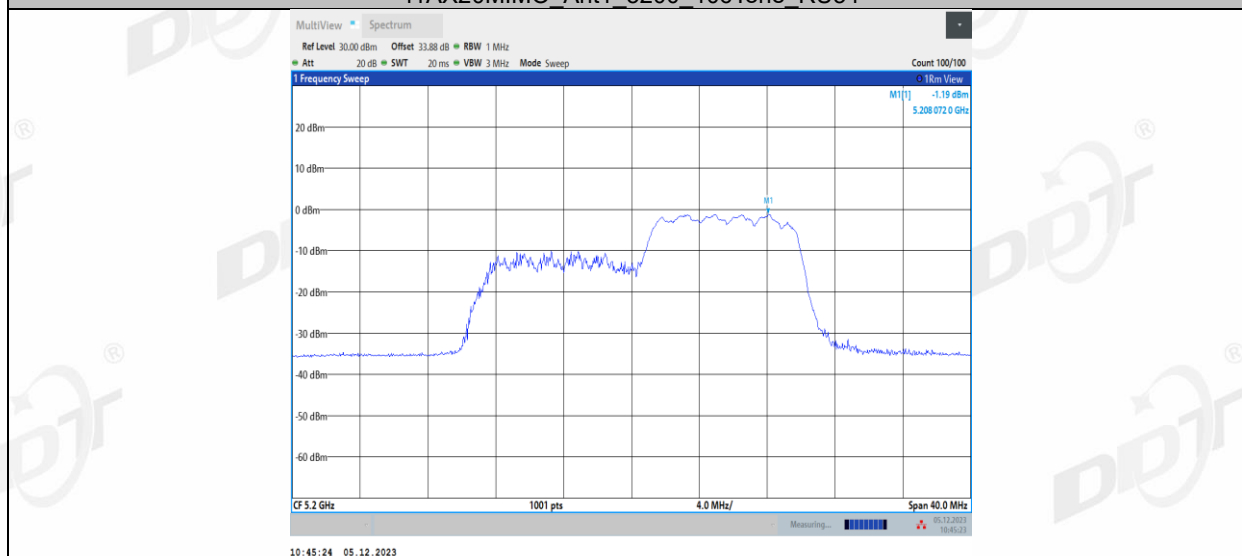
11AX20MIMO_Ant2_5200_26Tone_RU0
