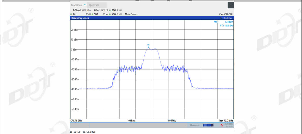
11AX20MIMO_Ant2_5180_26Tone_RU8
