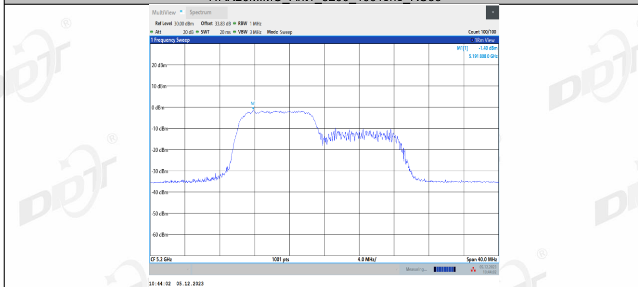
11AX20MIMO_Ant1_5200_106Tone_RU54
