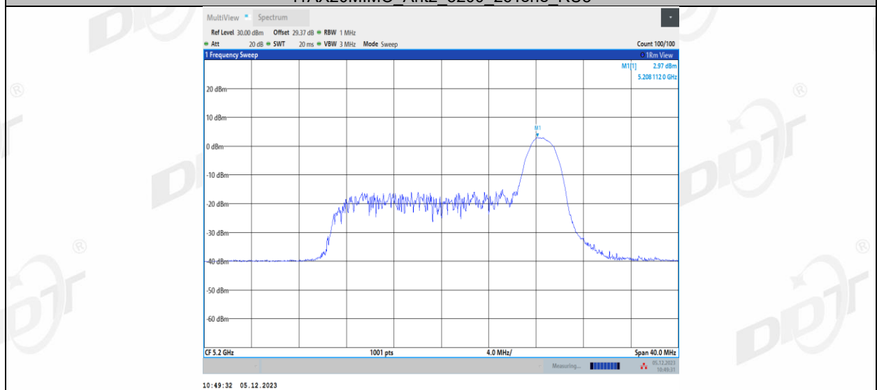
11AX20MIMO_Ant2_5200_52Tone_RU37
