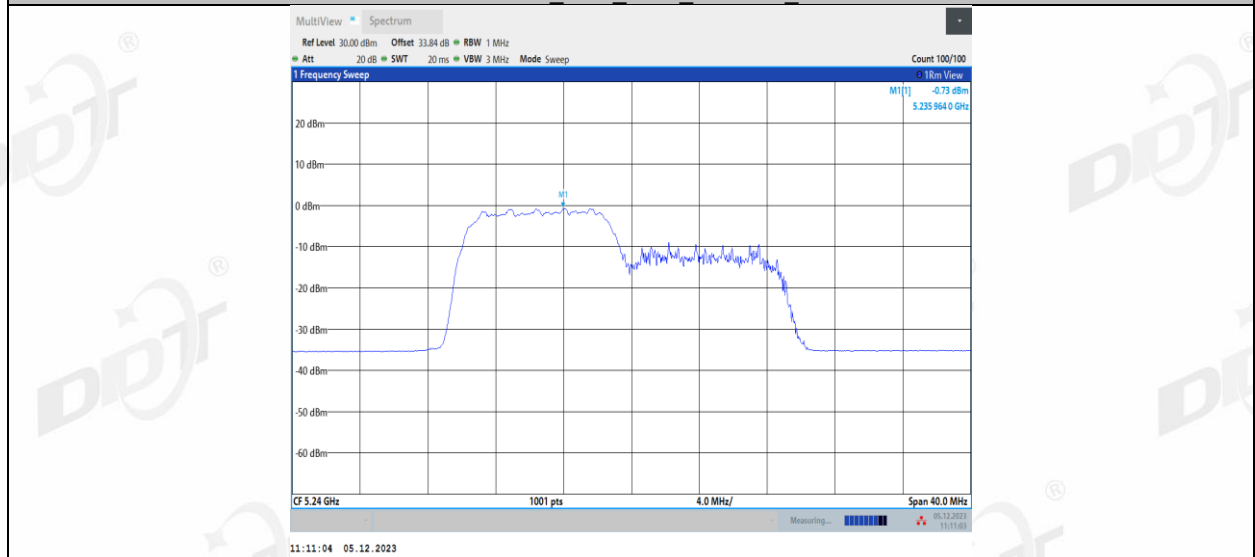
11AX20MIMO_Ant1_5240_106Tone_RU54
