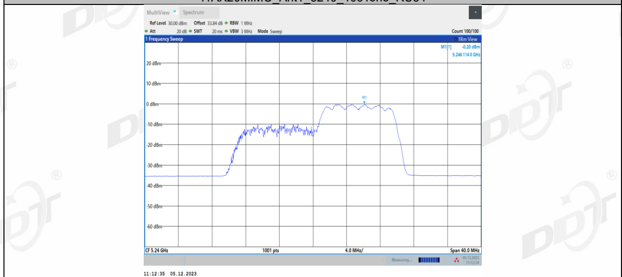
11AX20MIMO_Ant2_5240_26Tone_RU0
