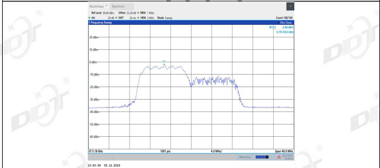
11AX20MIMO_Ant2_5180_106Tone_RU54
