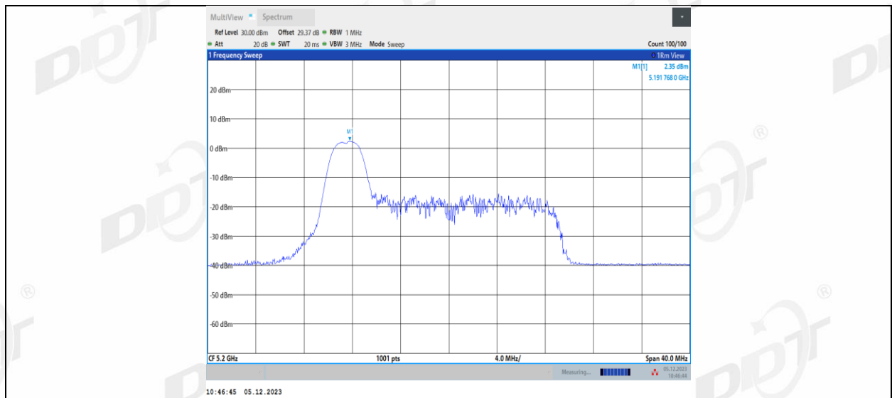
11AX20MIMO_Ant2_5200_26Tone_RU4
