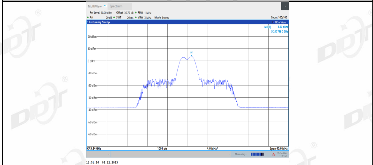
11AX20MIMO_Ant1_5240_26Tone_RU8
