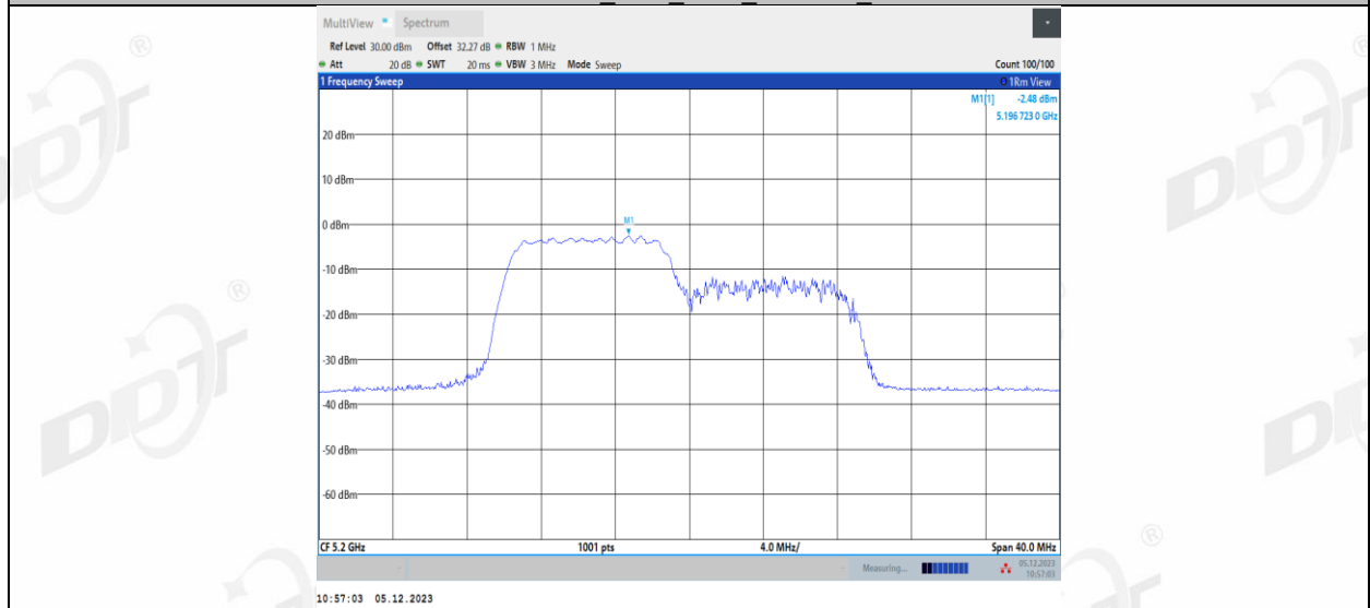
11AX20MIMO_Ant2_5200_106Tone_RU54
