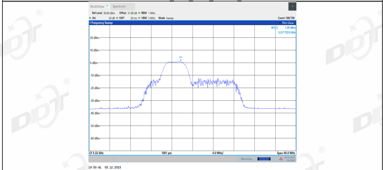
11AX20MIMO Ant1 5320_52Tone_RU39
