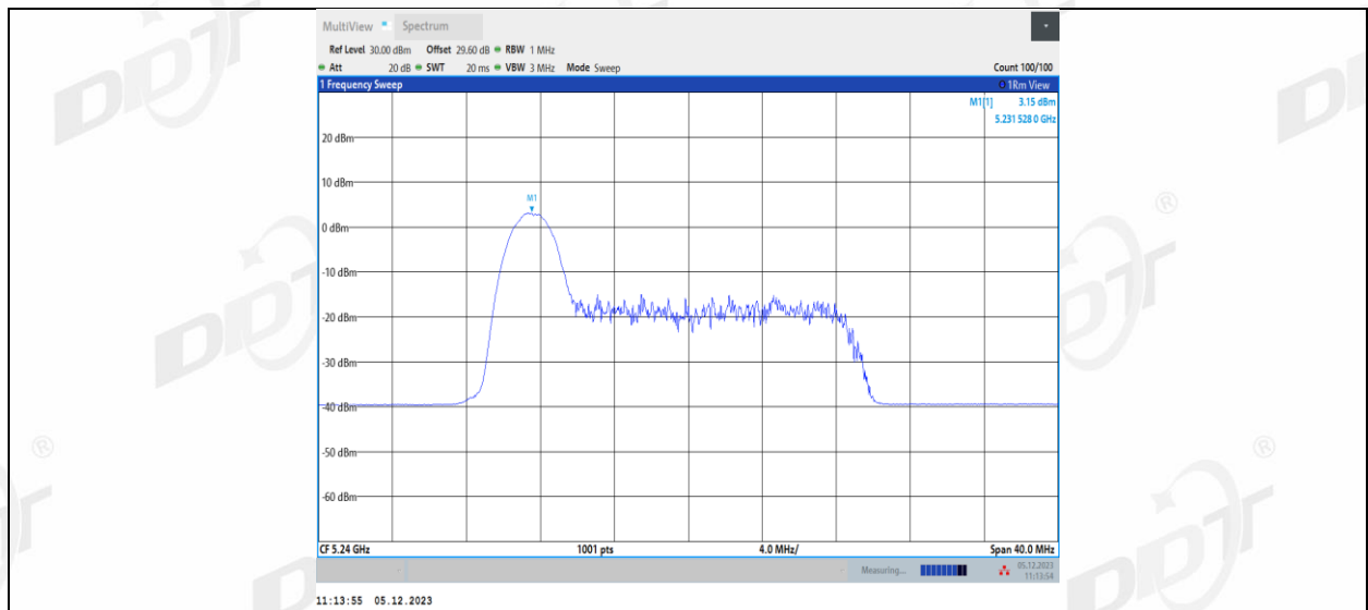
11AX20MIMO_Ant2_5240_26Tone_RU4
