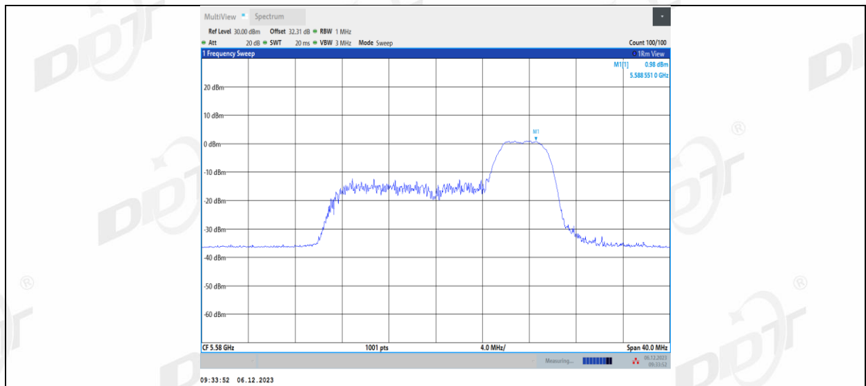
11AX20MIMO_Ant1_5580_106Tone_RU53
