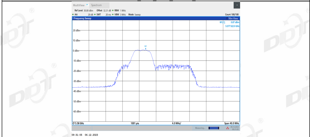
11AX20MIMO Ant1 5580_52Tone_RU39
