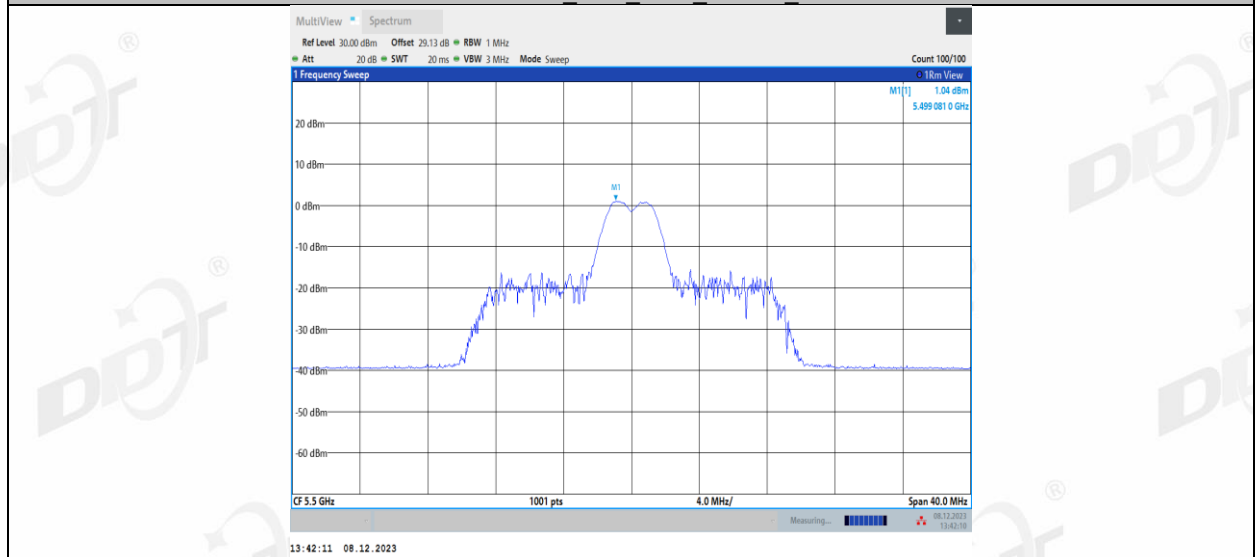
11AX20MIMO_Ant1_5500_26Tone_RU8
