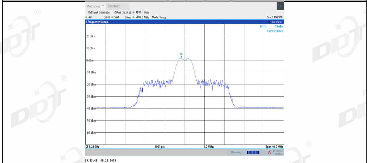
11AX20MIMO_Ant2_5280_26Tone_RU8
