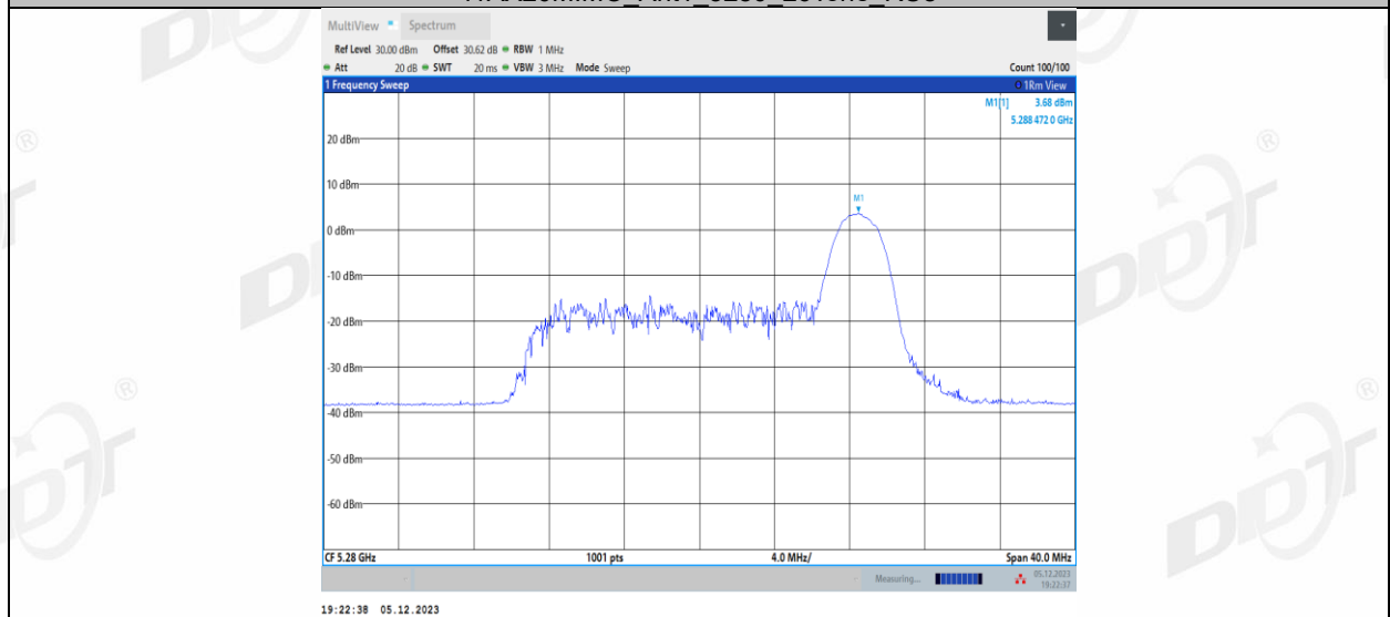
11AX20MIMO_Ant1_5280_52Tone_RU37
