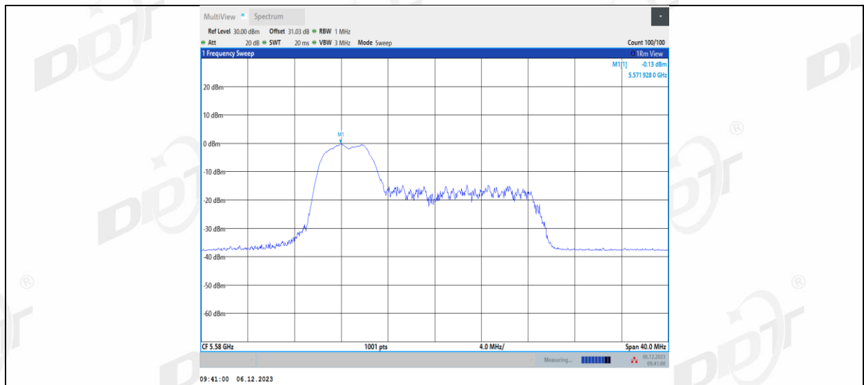
11AX20MIMO_Ant2_5580_52Tone_RU38
