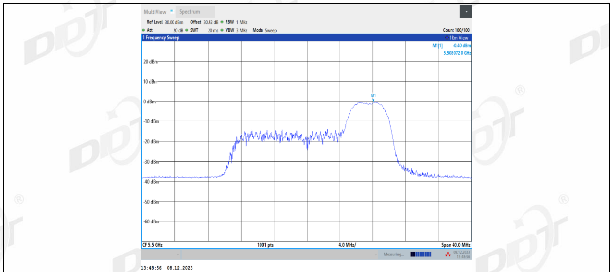
11AX20MIMO_Ant1_5500_106Tone_RU53
