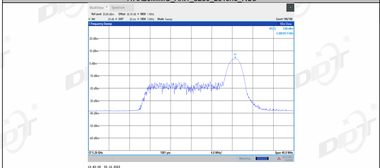
11AX20MIMO_Ant1_5260_52Tone_RU37
