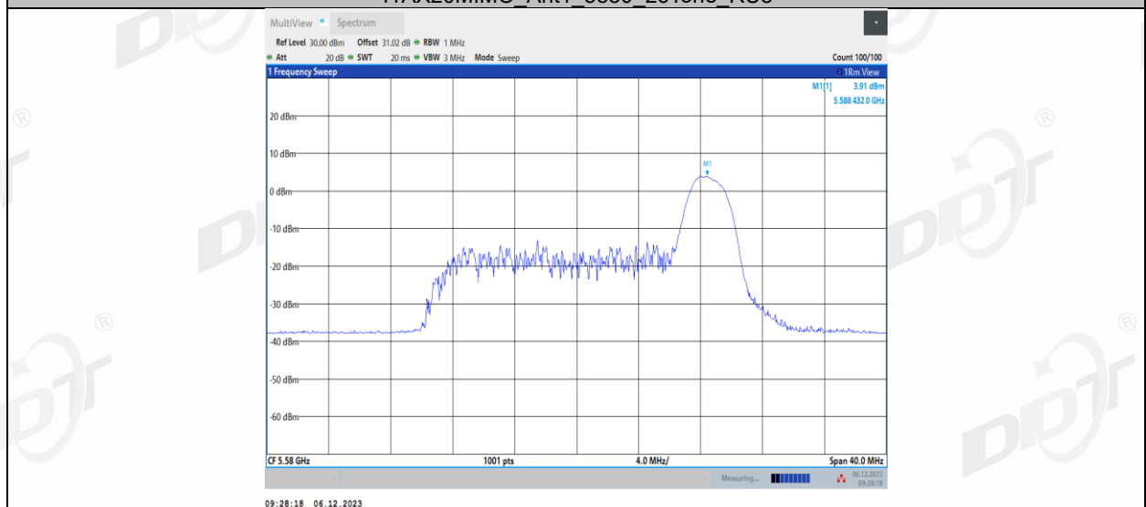
11AX20MIMO_Ant1_5580_52Tone_RU37
