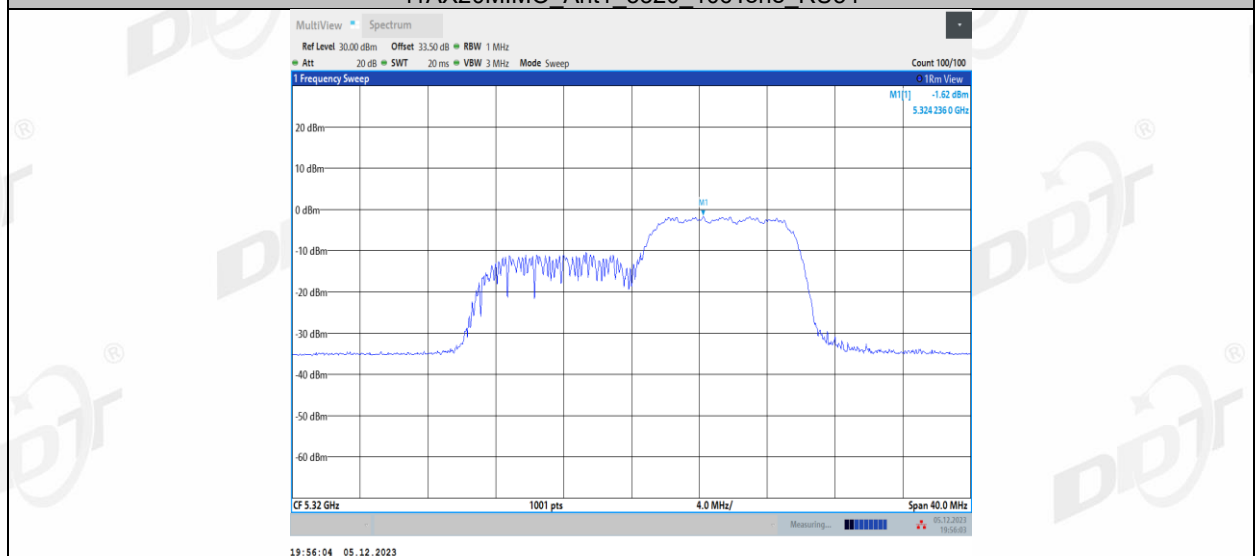
11AX20MIMO_Ant2_5320_26Tone_RU0
