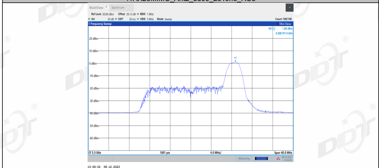
11AX20MIMO_Ant2_5500_52Tone_RU37
