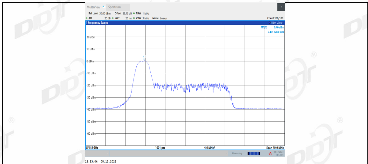
11AX20MIMO_Ant2_5500_26Tone_RU4
