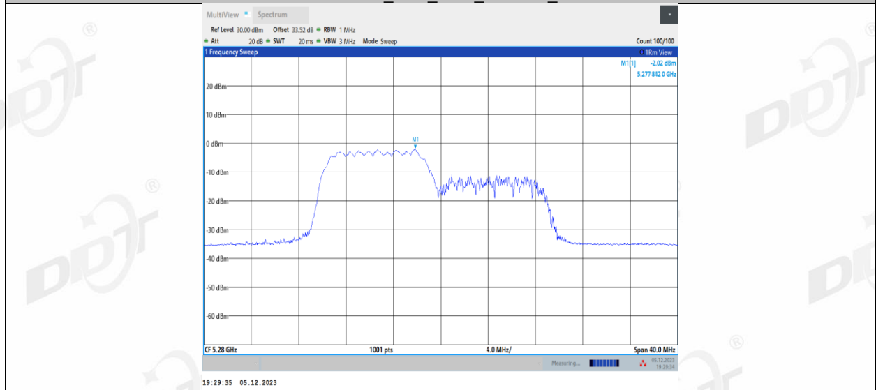
11AX20MIMO_Ant1_5280_106Tone_RU54
