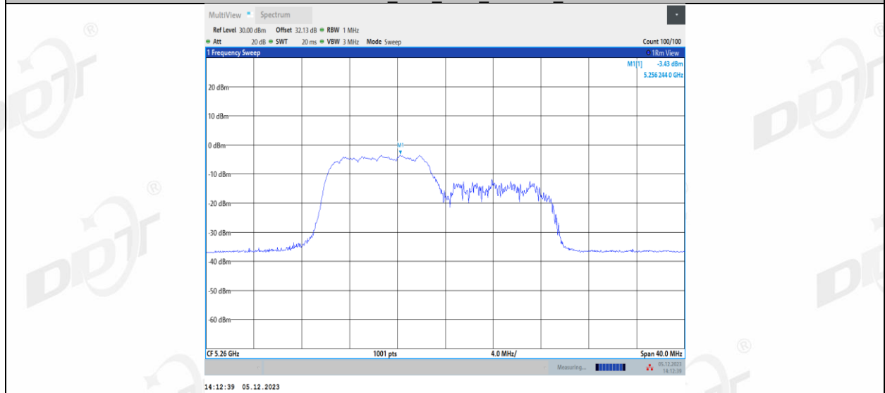
11AX20MIMO_Ant2_5260_106Tone_RU54
