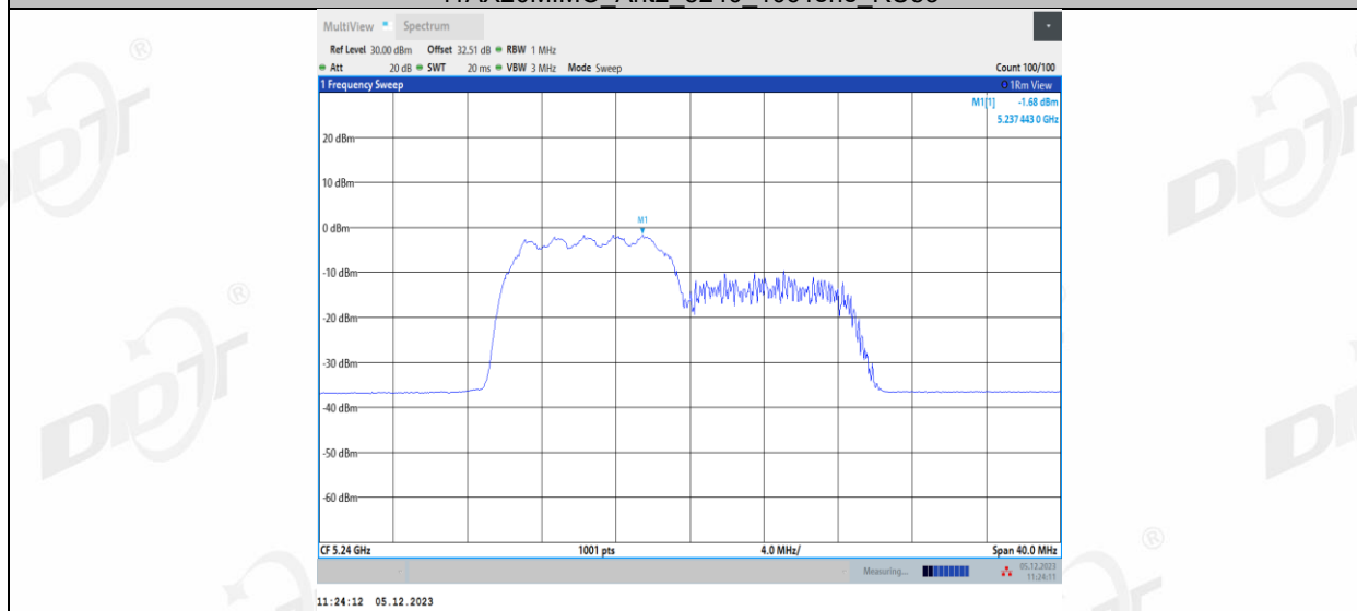
11AX20MIMO_Ant2_5240_106Tone_RU54
