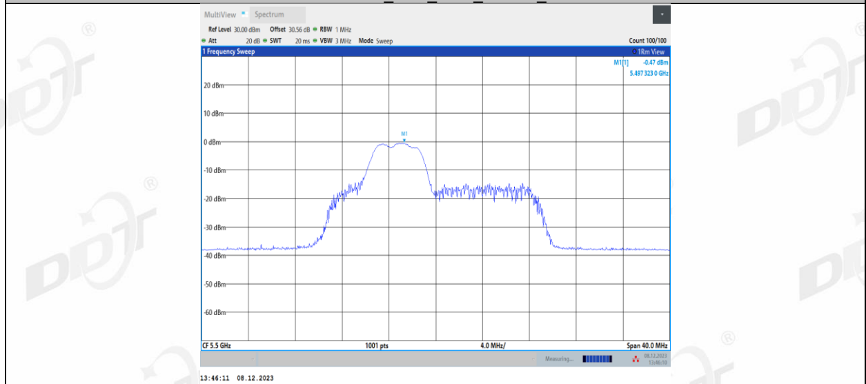
11AX20MIMO_Ant1_5500_52Tone_RU39
