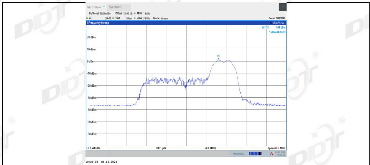
11AX20MIMO_Ant1_5280_106Tone_RU53
