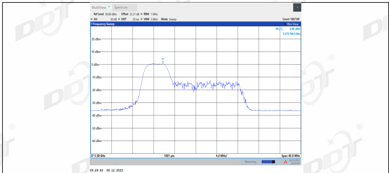
11AX20MIMO Ant1 5580_52Tone_RU38
