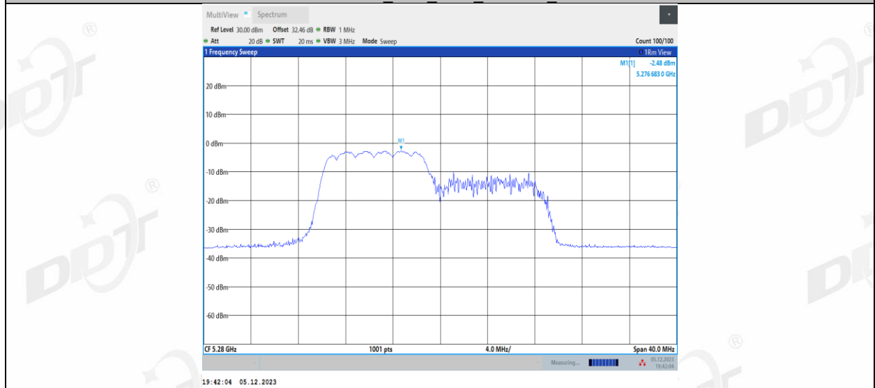
11AX20MIMO_Ant2_5280_106Tone_RU54
