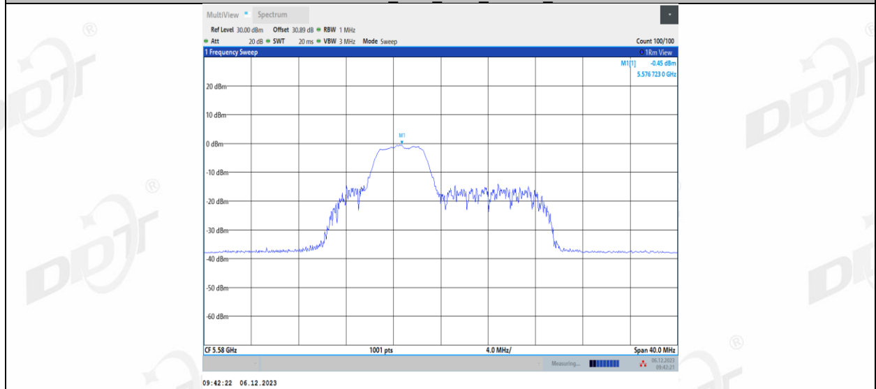
11AX20MIMO_Ant2_5580_52Tone_RU39
