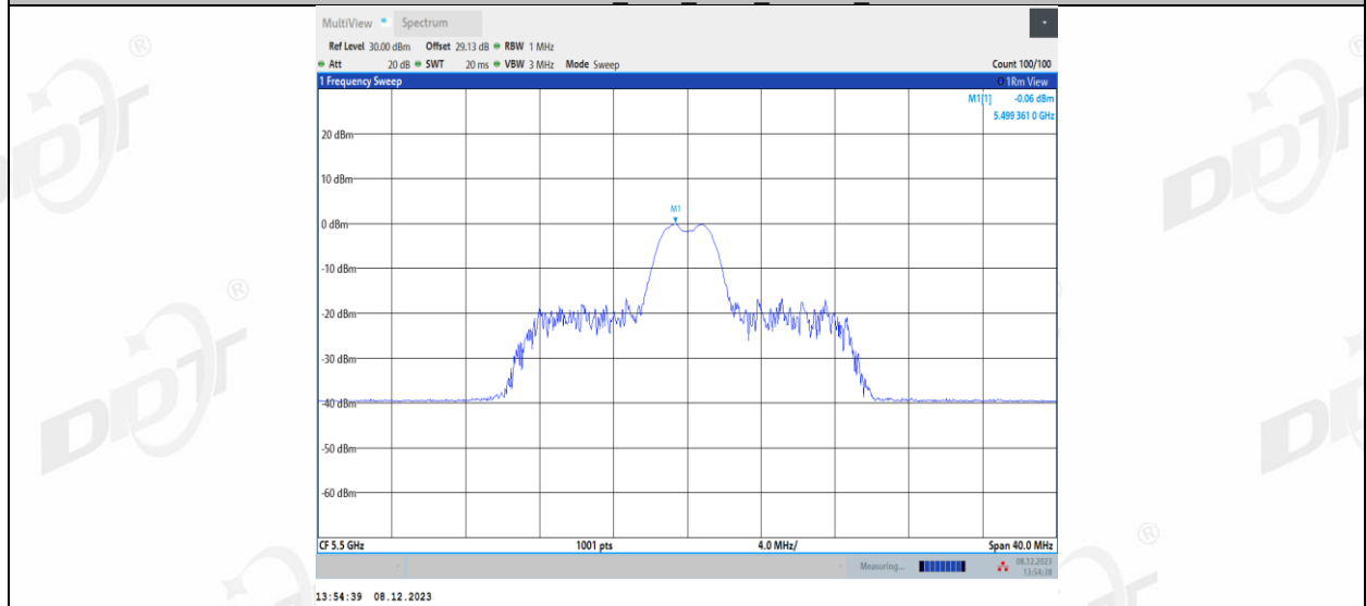
11AX20MIMO_Ant2_5500_26Tone_RU8
