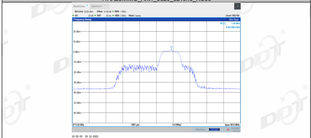
11AX20MIMO Ant1 5320_52Tone_RU40
