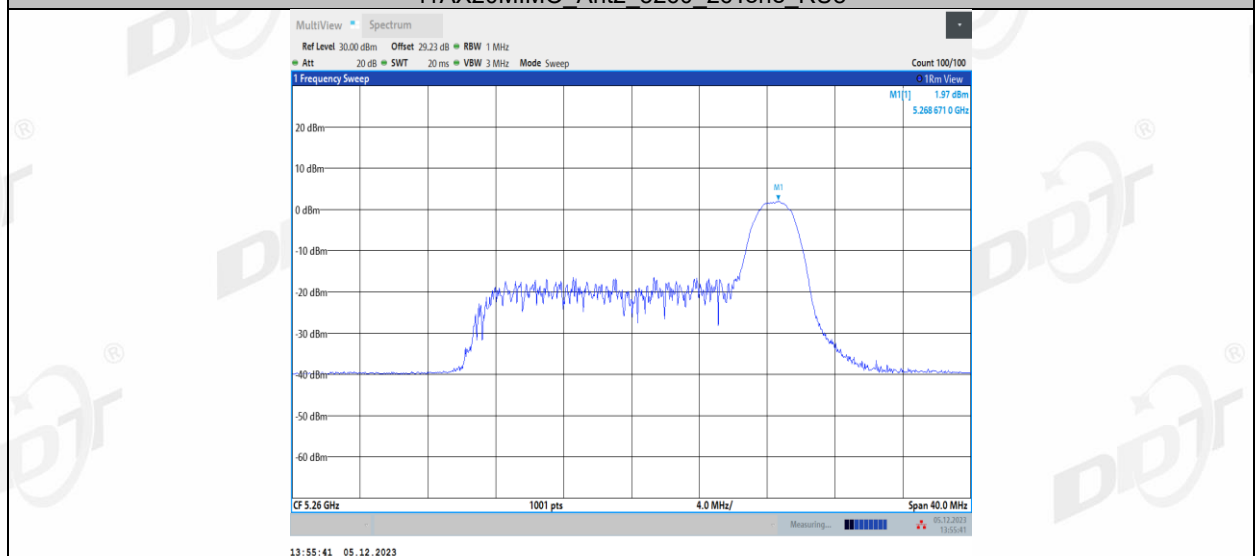
11AX20MIMO_Ant2_5260_52Tone_RU37
