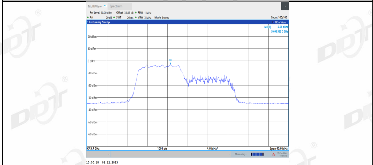
11AX20MIMO_Ant1_5700_106Tone_RU54
