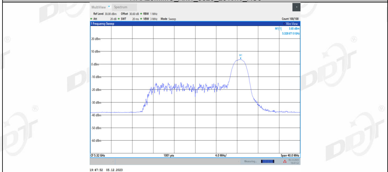
11AX20MIMO_Ant1_5320_52Tone_RU37
