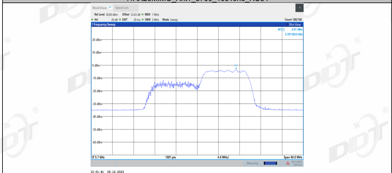
11AX20MIMO_Ant2_5700_26Tone_RU0
