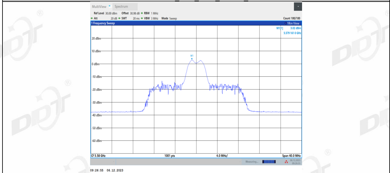
11AX20MIMO_Ant1_5580_26Tone_RU8
