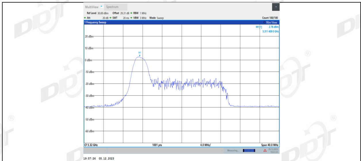
11AX20MIMO_Ant2_5320_26Tone_RU4
