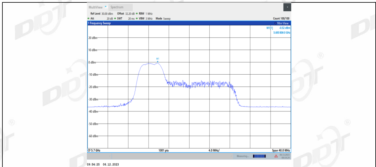
11AX20MIMO Ant1 5700_52Tone_RU38
