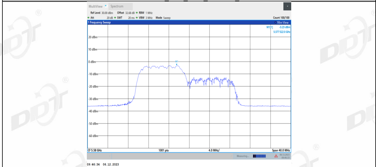
11AX20MIMO_Ant2_5580_106Tone_RU54
