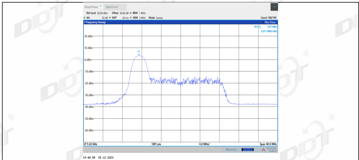
11AX20MIMO_Ant1_5320_26Tone_RU4
