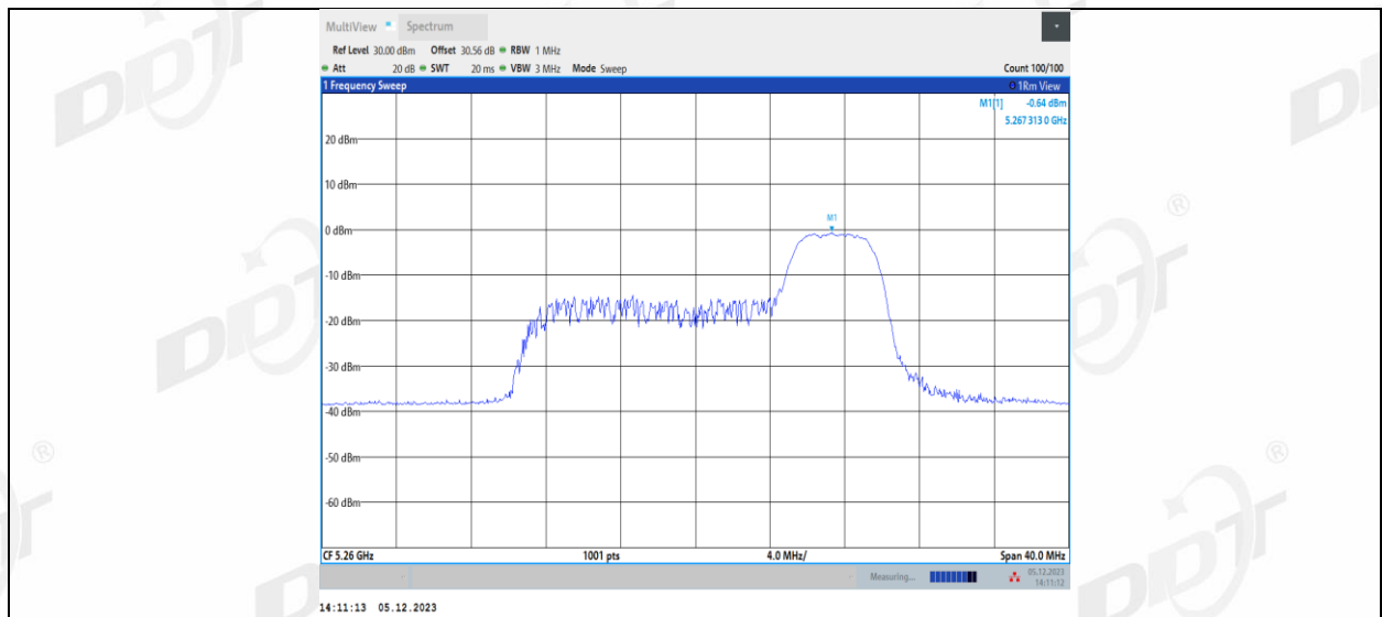
11AX20MIMO_Ant2_5260_106Tone_RU53
