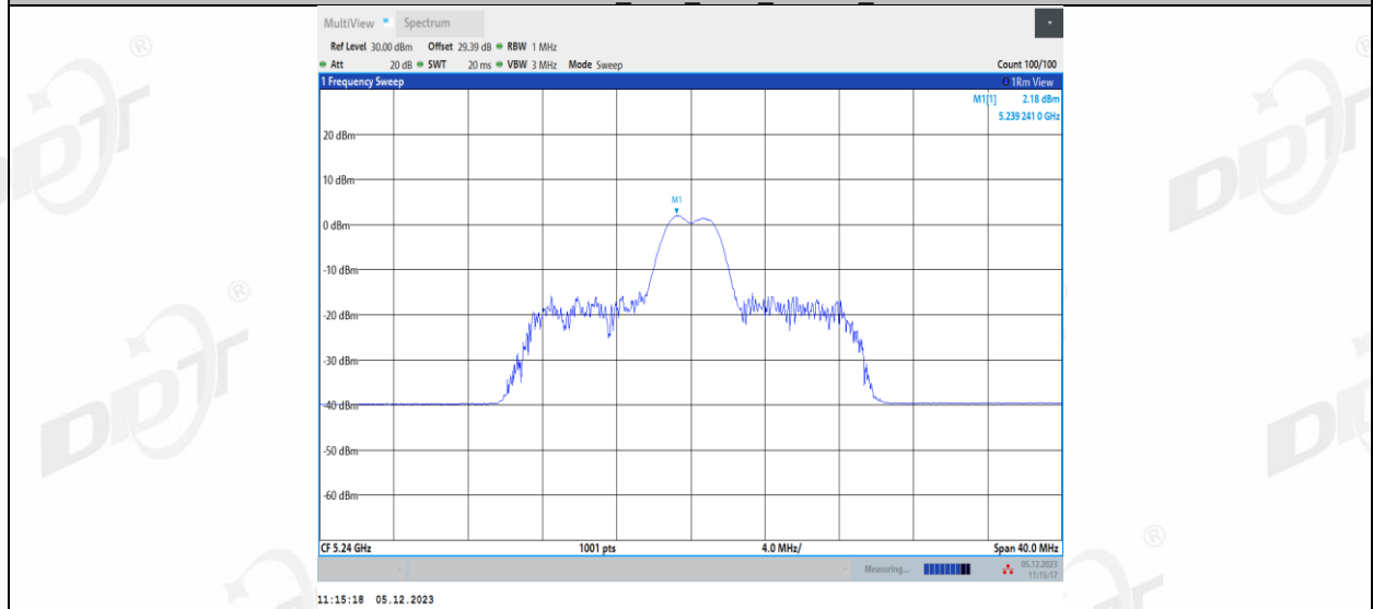
11AX20MIMO_Ant2_5240_26Tone_RU8
