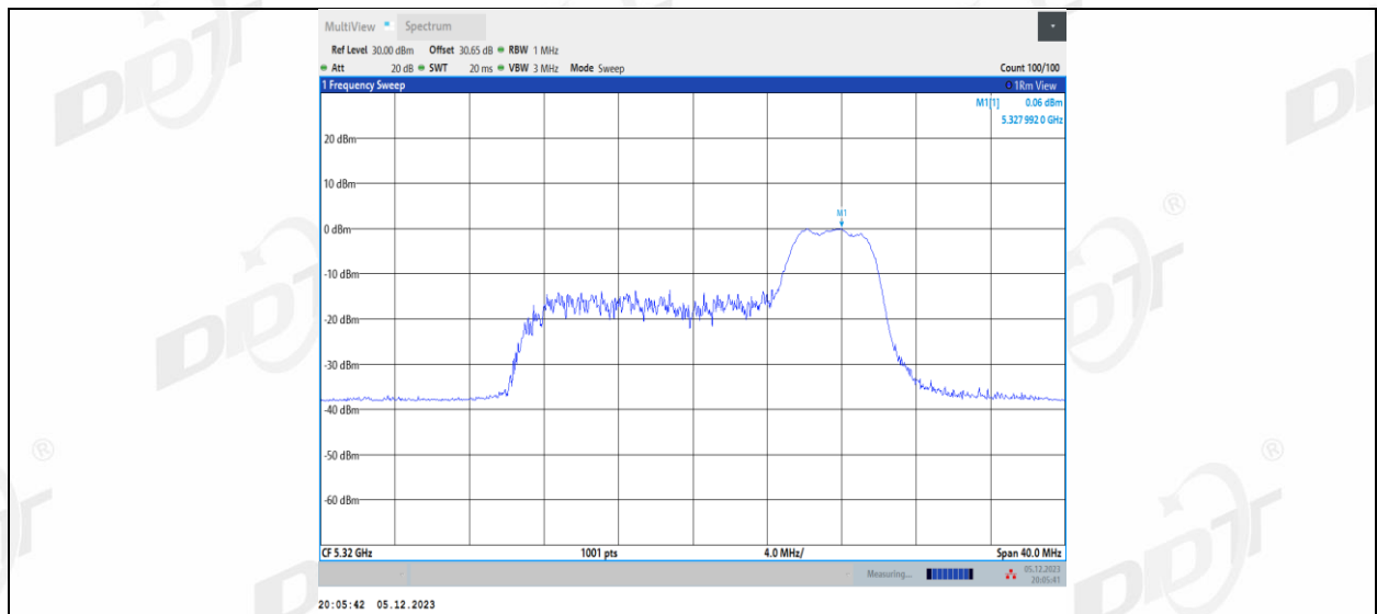
11AX20MIMO_Ant2_5320_106Tone_RU53
