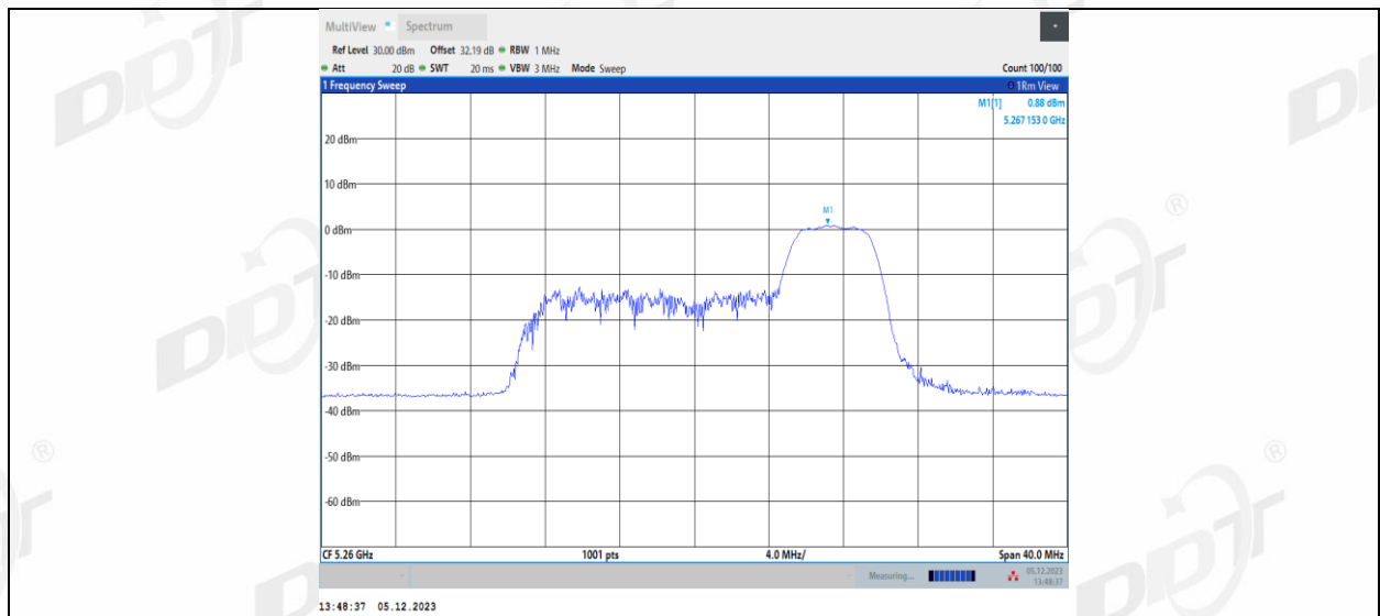
11AX20MIMO_Ant1_5260_106Tone_RU53
