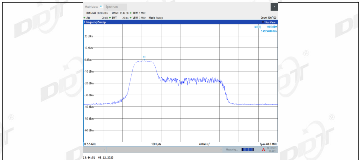
11AX20MIMO_Ant1_5500_52Tone_RU38
