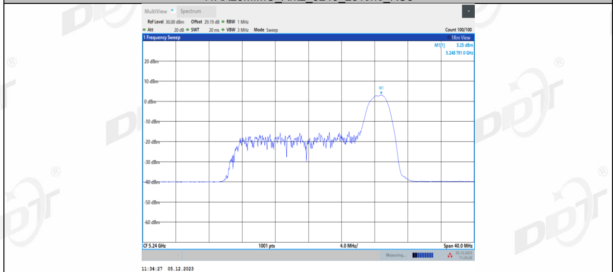
11AX20MIMO_Ant2_5240_52Tone_RU37
