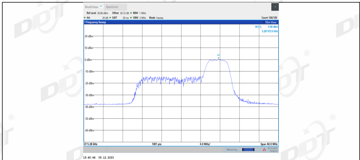
11AX20MIMO_Ant2_5280_106Tone_RU53
