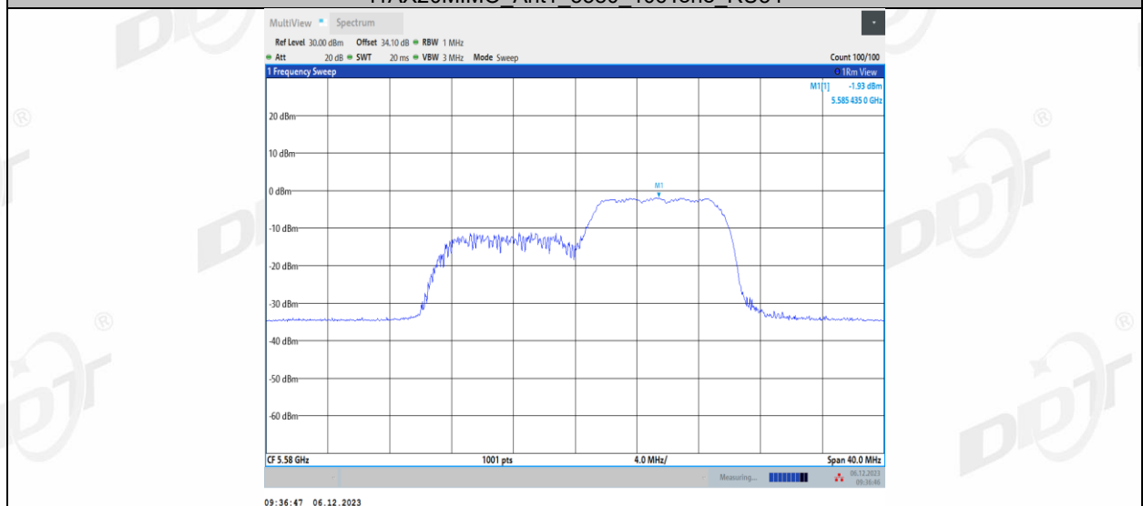
11AX20MIMO_Ant2_5580_26Tone_RU0
