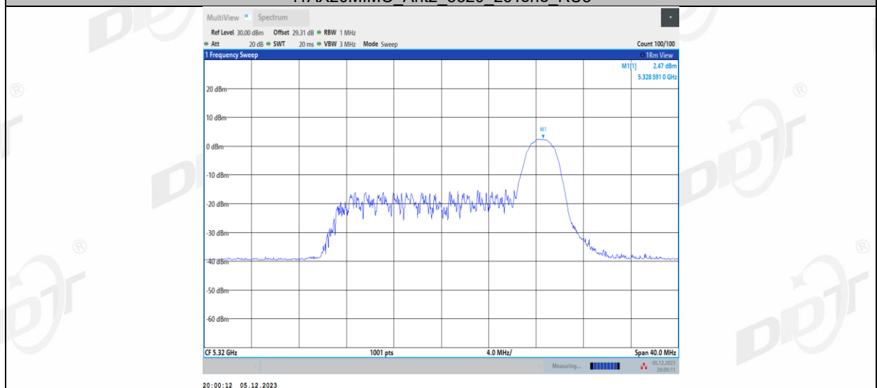
11AX20MIMO_Ant2_5320_52Tone_RU37
