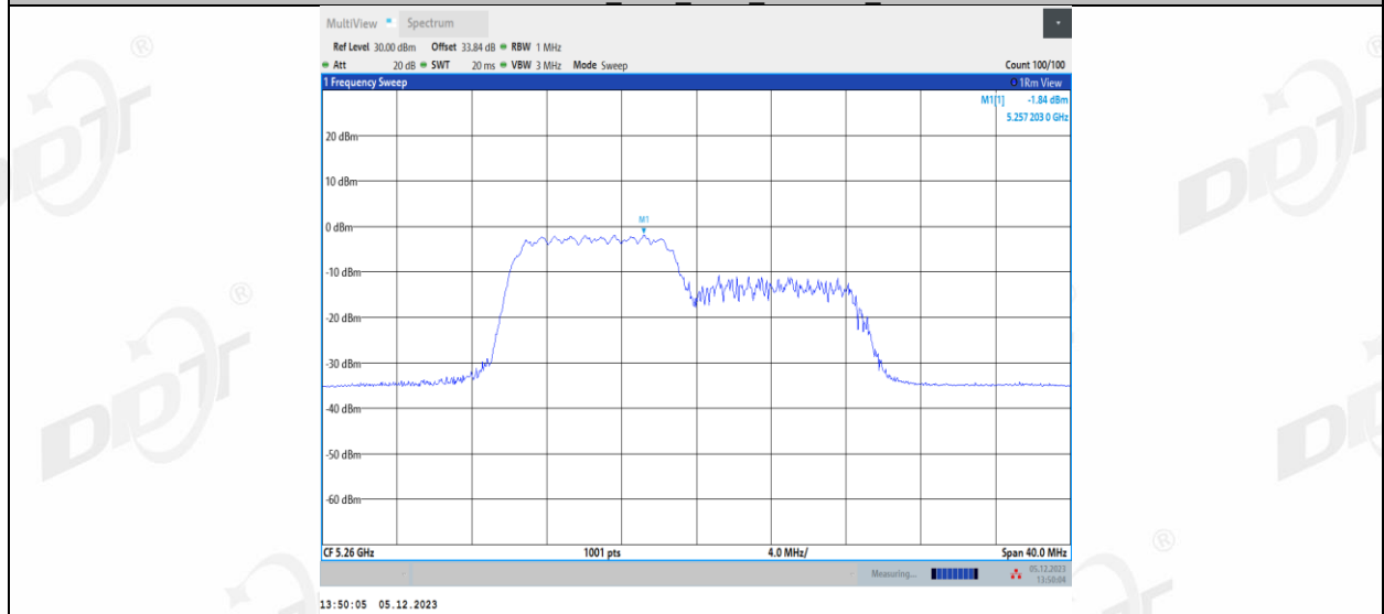
11AX20MIMO_Ant1_5260_106Tone_RU54
