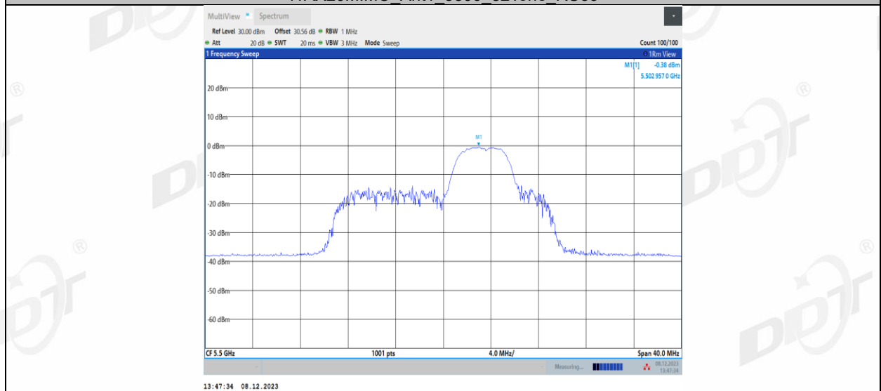
11AX20MIMO_Ant1_5500_52Tone_RU40
