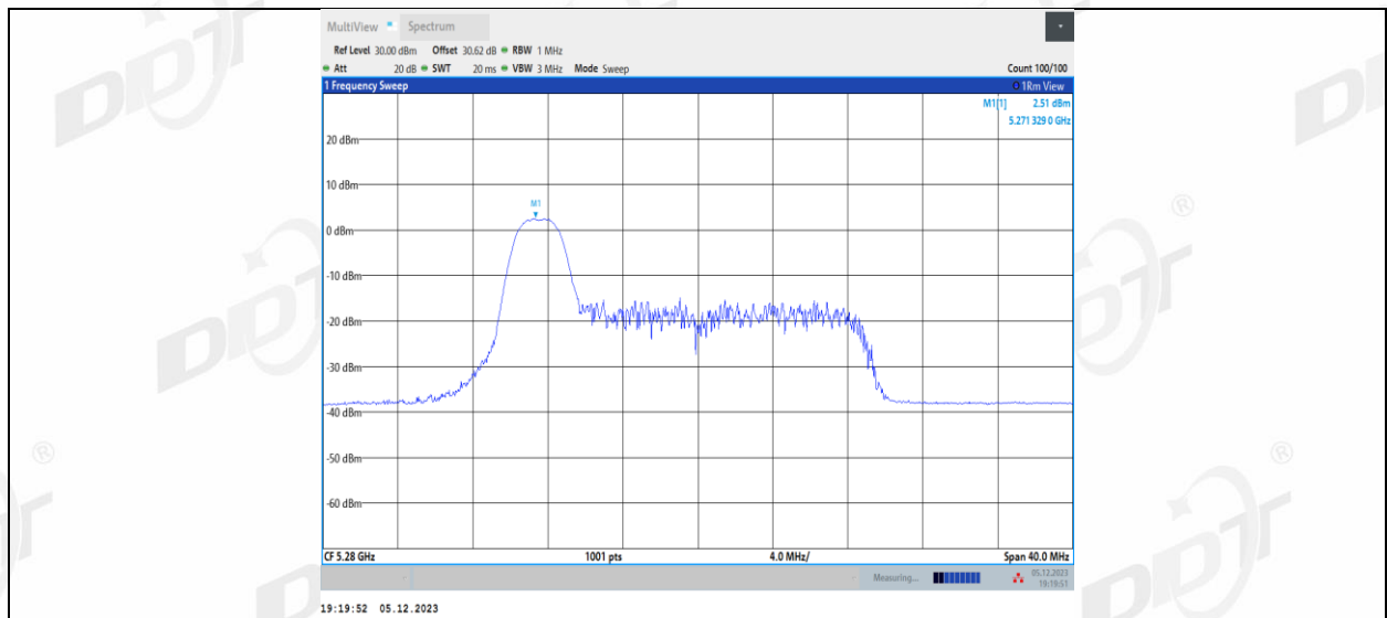
11AX20MIMO_Ant1_5280_26Tone_RU4
