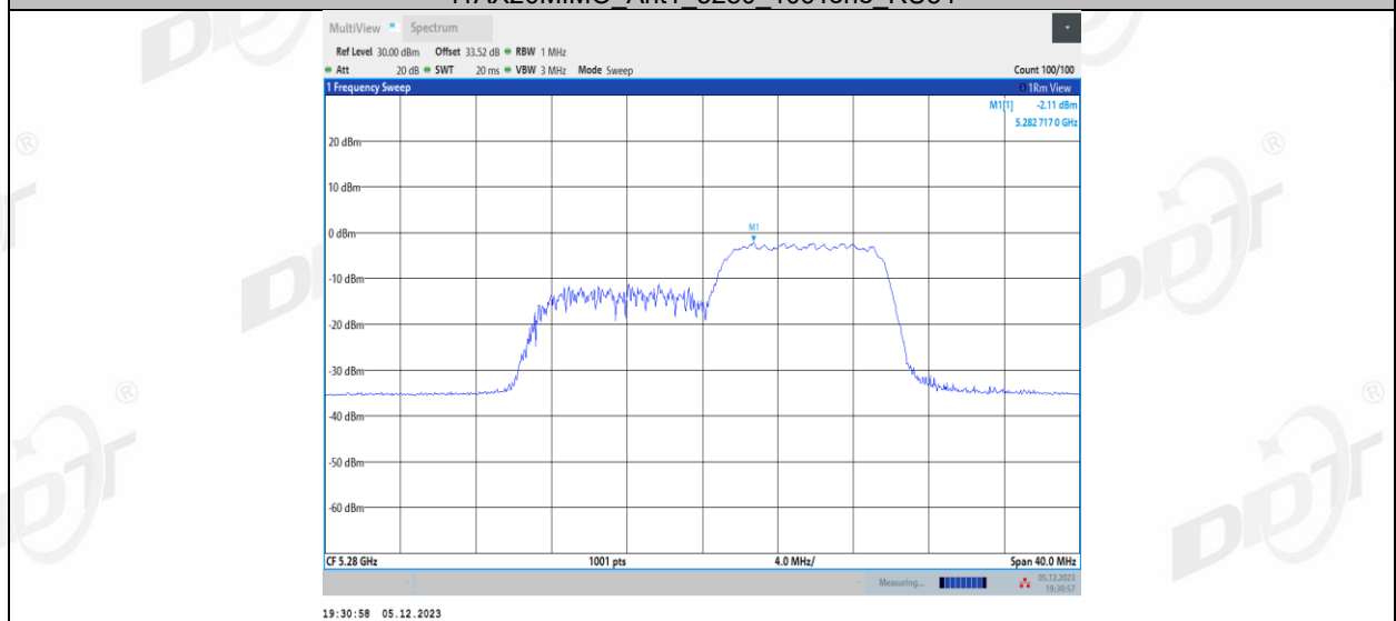
11AX20MIMO_Ant2_5280_26Tone_RU0
