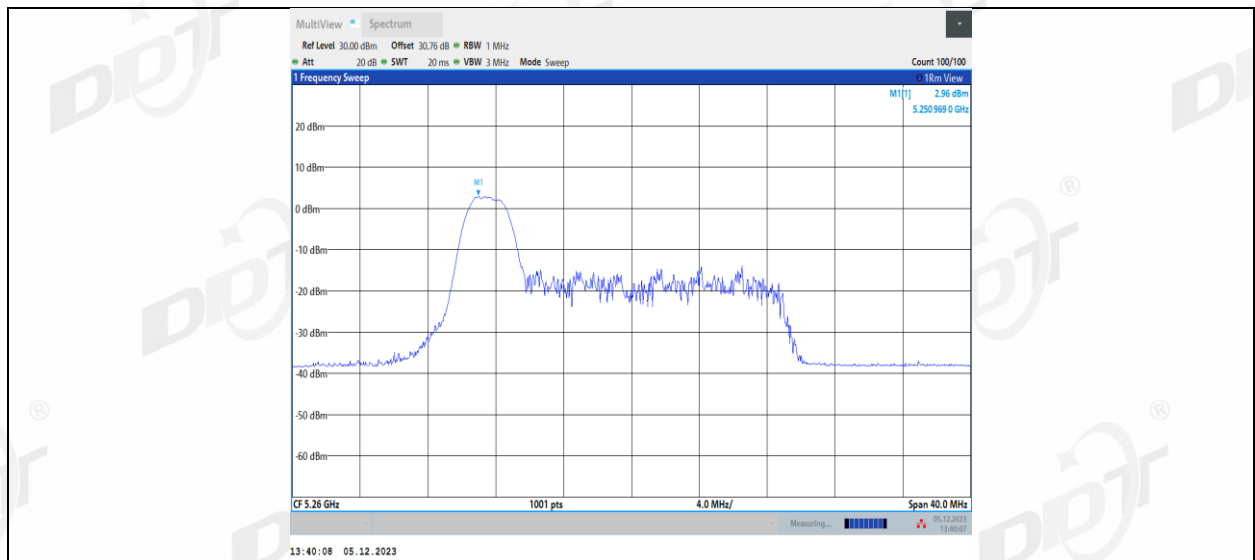
11AX20MIMO_Ant1_5260_26Tone_RU4
