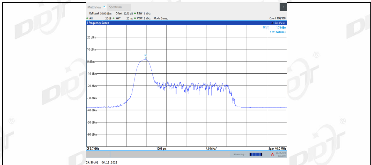
11AX20MIMO_Ant1_5700_26Tone_RU4
