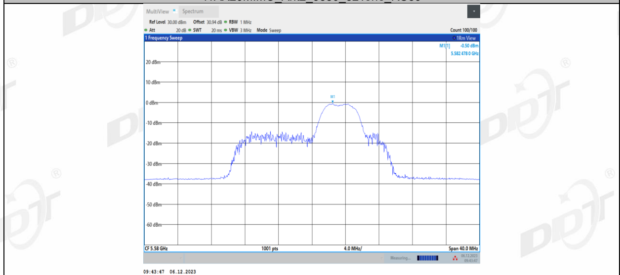
11AX20MIMO_Ant2_5580_52Tone_RU40
