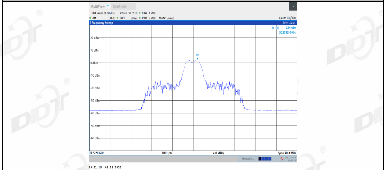
11AX20MIMO_Ant1_5280_26Tone_RU8
