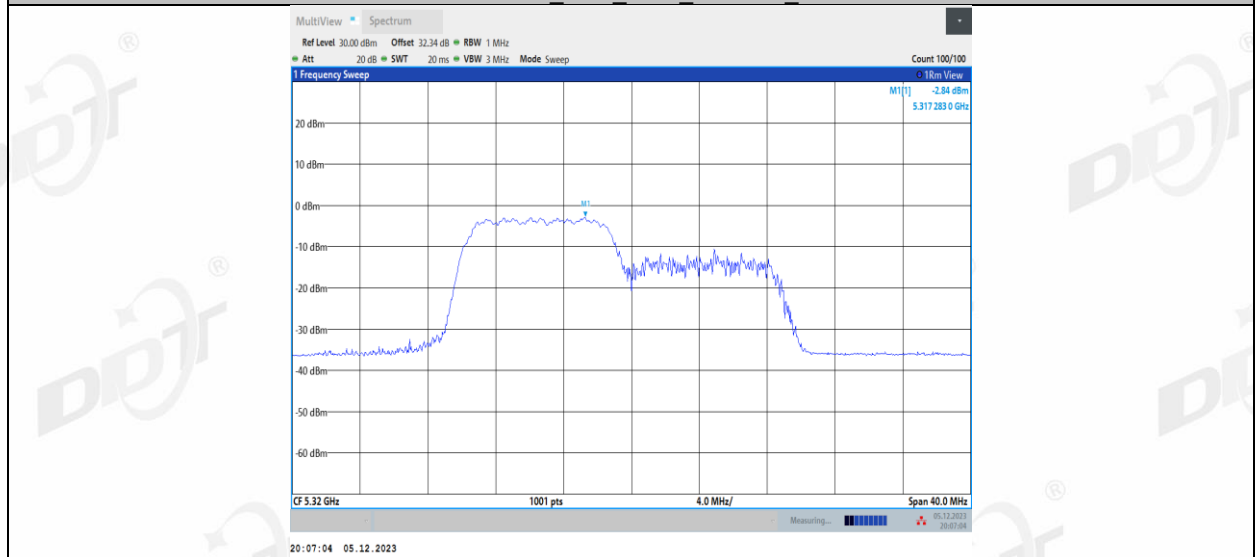
11AX20MIMO_Ant2_5320_106Tone_RU54
