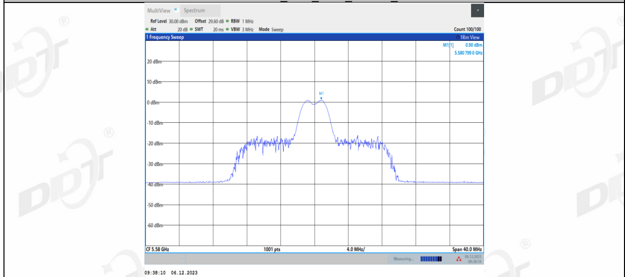
11AX20MIMO_Ant2_5580_26Tone_RU8
