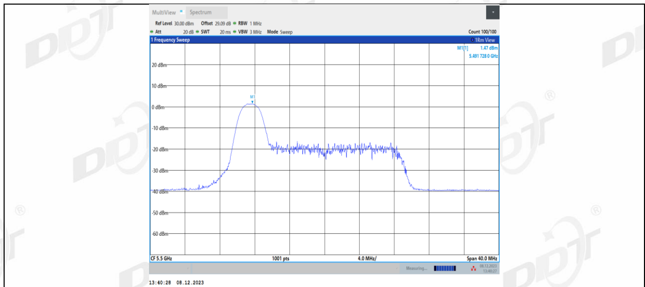
11AX20MIMO_Ant1_5500_26Tone_RU4
