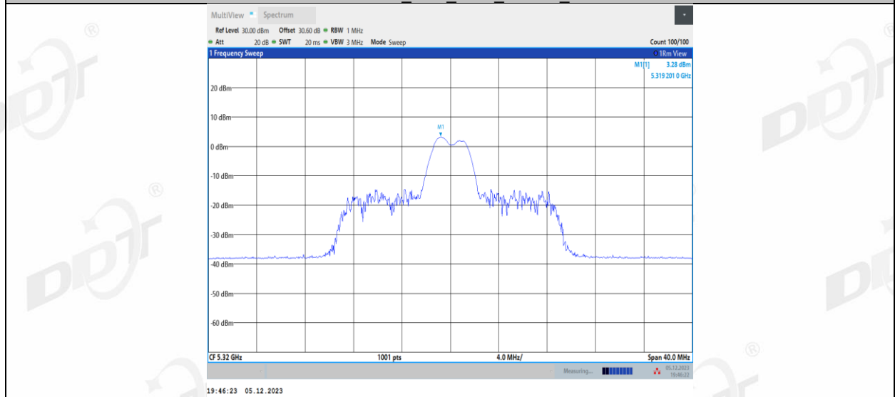
11AX20MIMO_Ant1_5320_26Tone_RU8
