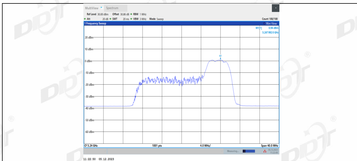
11AX20MIMO_Ant2_5240_106Tone_RU53
