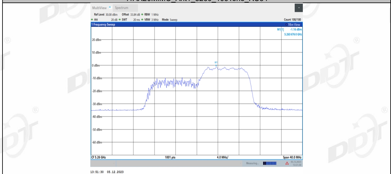
11AX20MIMO_Ant2_5260_26Tone_RU0
