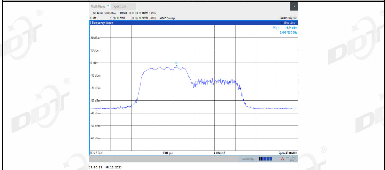
11AX20MIMO_Ant1_5500_106Tone_RU54
