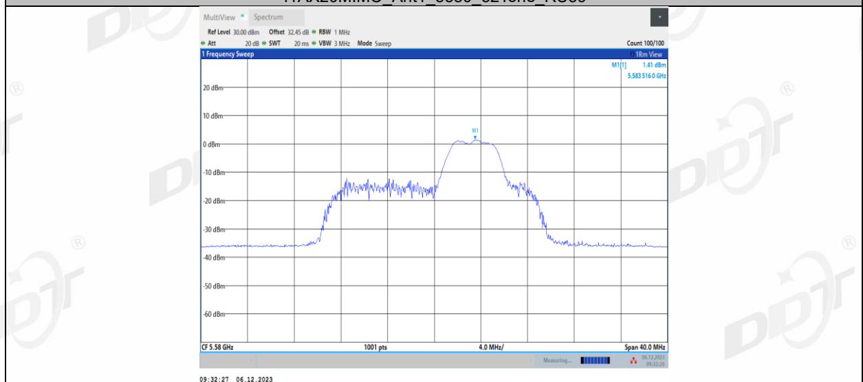
11AX20MIMO Ant1 5580_52Tone_RU40
