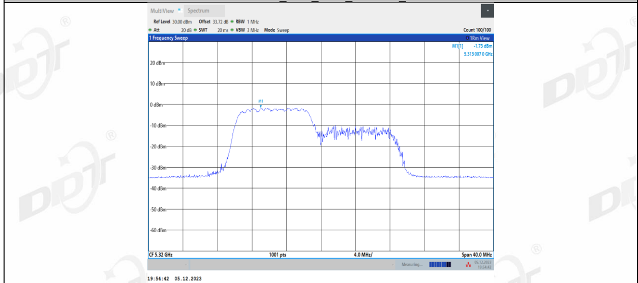
11AX20MIMO_Ant1_5320_106Tone_RU54
