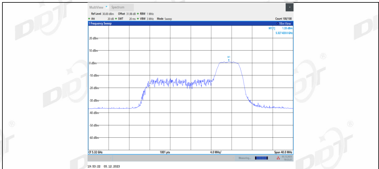
11AX20MIMO_Ant1_5320_106Tone_RU53
