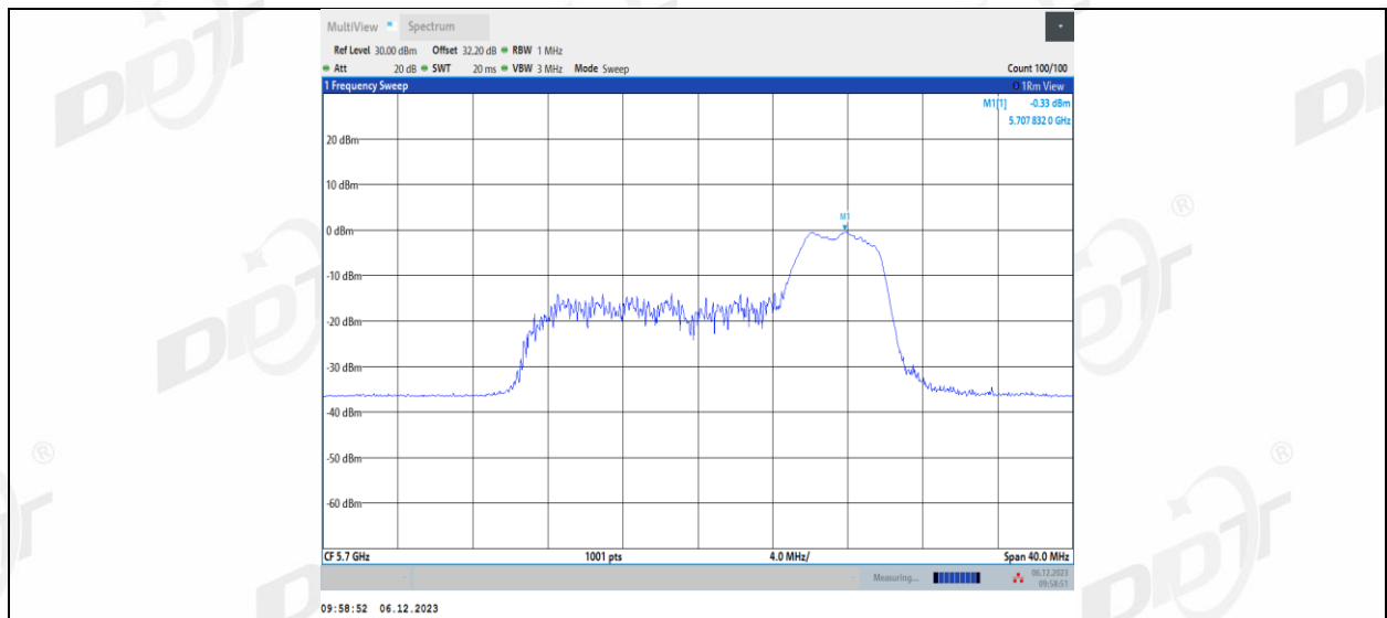
11AX20MIMO_Ant1_5700_106Tone_RU53
