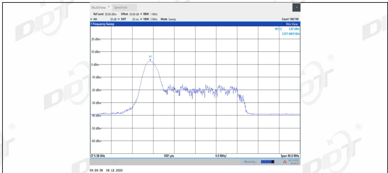
11AX20MIMO_Ant2_5580_26Tone_RU4
