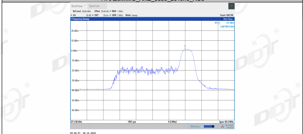
11AX20MIMO_Ant2_5580_52Tone_RU37
