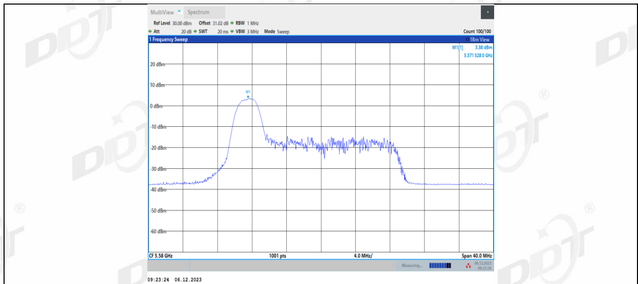
11AX20MIMO_Ant1_5580_26Tone_RU4
