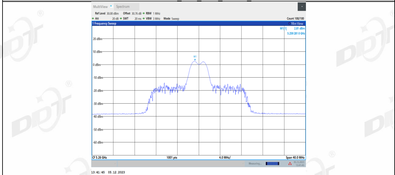
11AX20MIMO_Ant1_5260_26Tone_RU8
