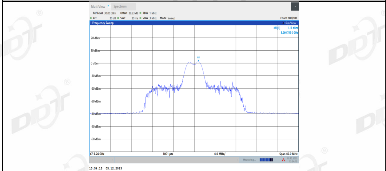
11AX20MIMO_Ant2_5260_26Tone_RU8
