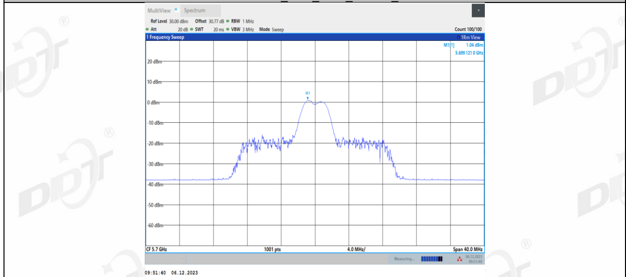
11AX20MIMO_Ant1_5700_26Tone_RU8
