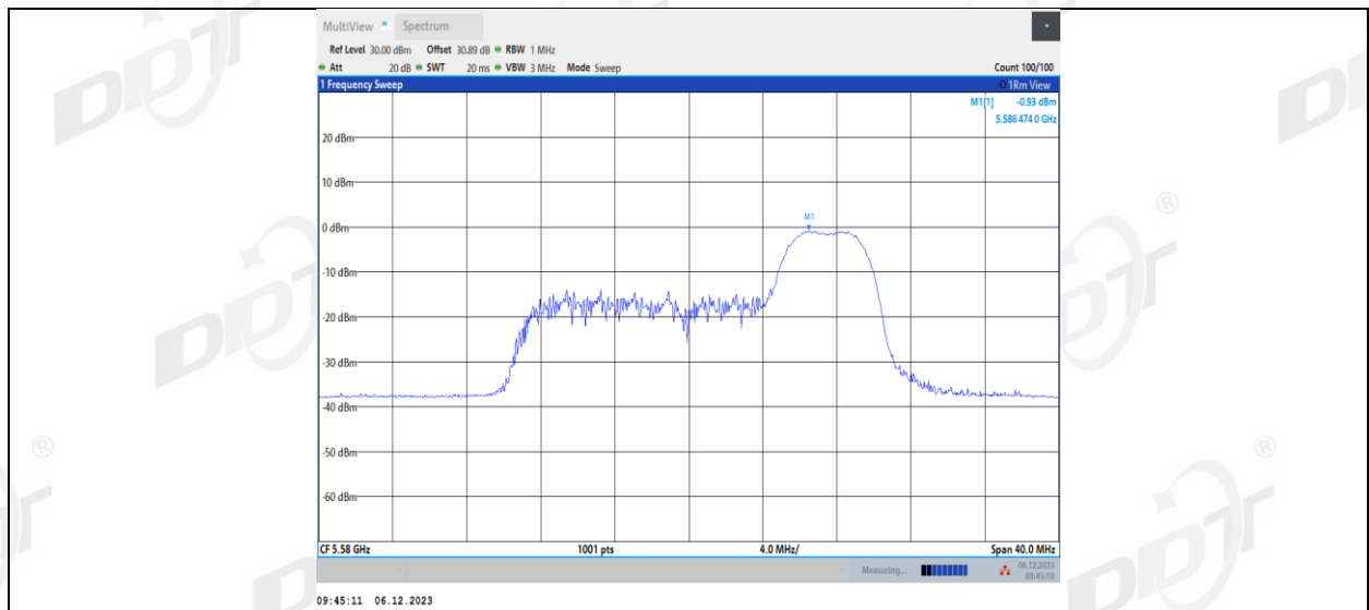
11AX20MIMO_Ant2_5580_106Tone_RU53
