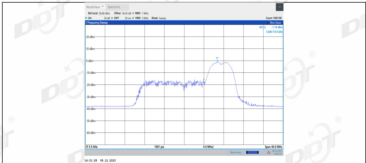
11AX20MIMO_Ant2_5500_106Tone_RU53
