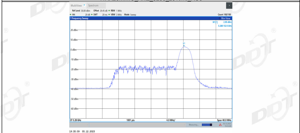
11AX20MIMO_Ant2_5280_52Tone_RU37
