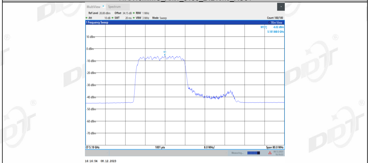
11AX40MIMO_Ant1_5190_242Tone_RU62
