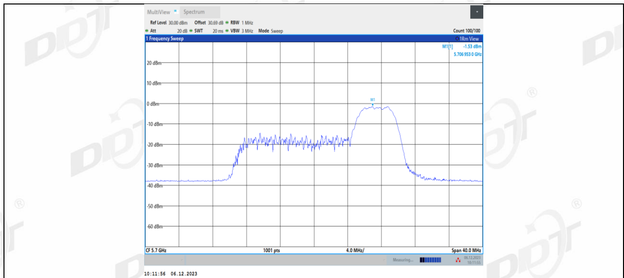
11AX20MIMO_Ant2_5700_106Tone_RU53
