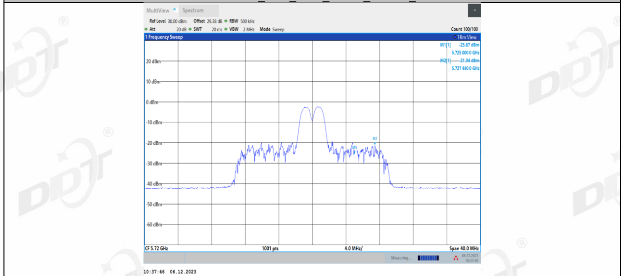
11AX20MIMO_Ant2_5720_UNII-3_26Tone_RU8
