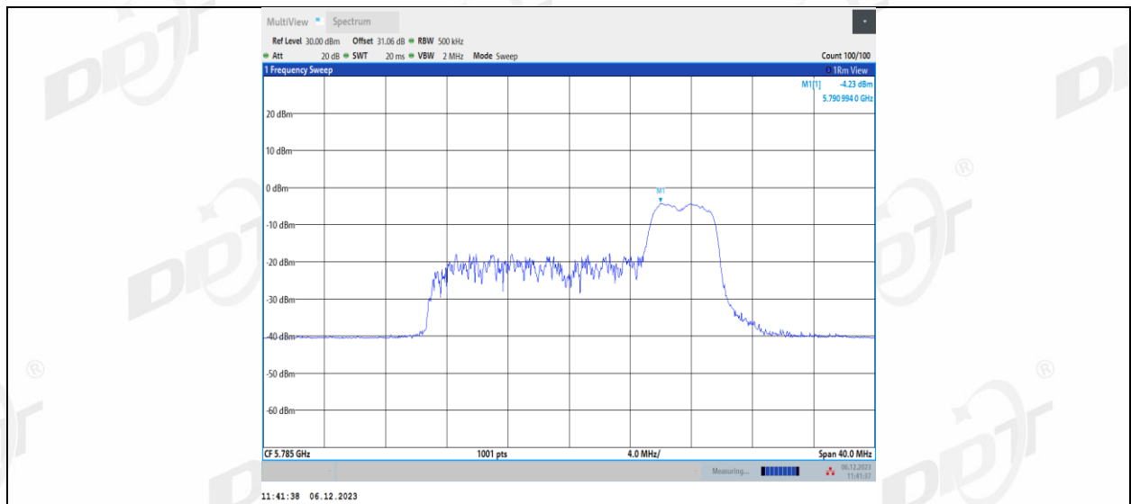
11AX20MIMO_Ant2_5785_106Tone_RU53
