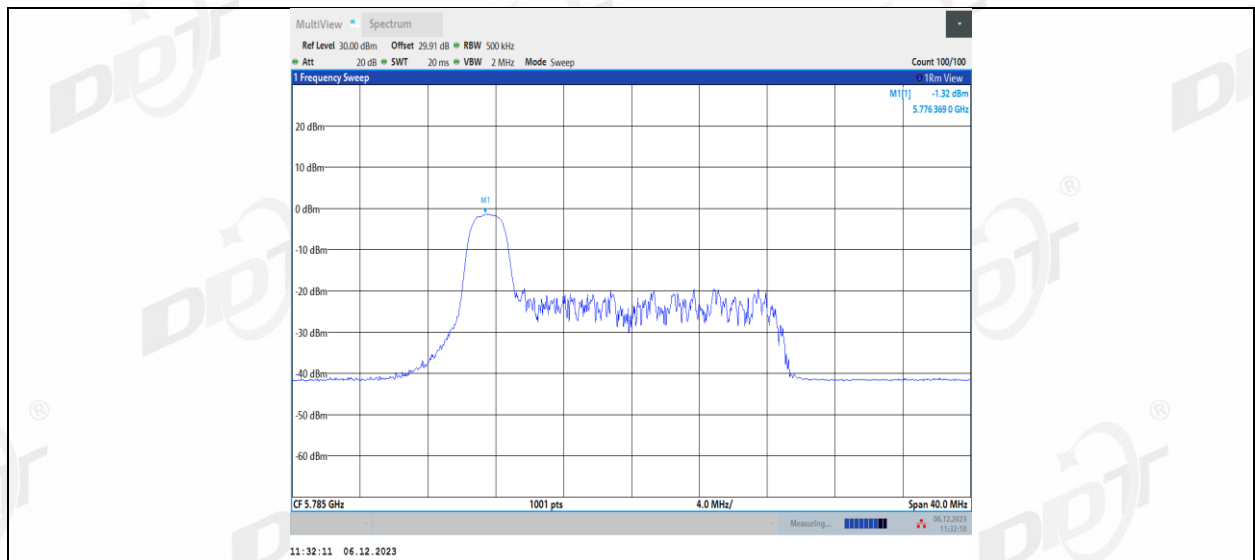
11AX20MIMO_Ant2_5785_26Tone_RU4
