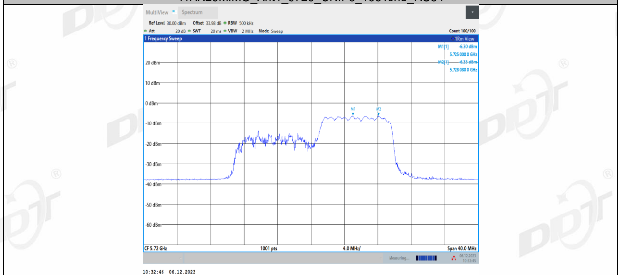
11AX20MIMO_Ant2_5720_UNII-3_26Tone_RU0
