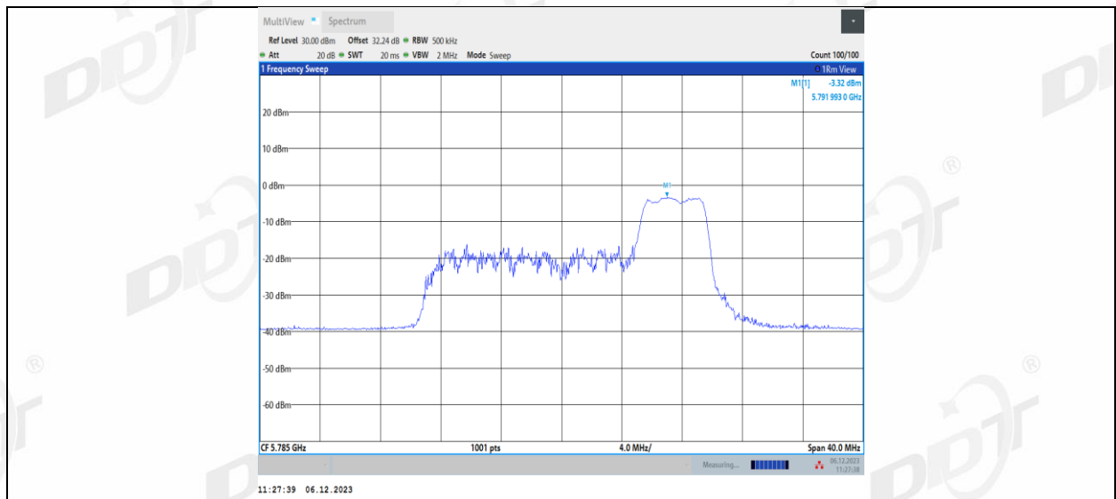
11AX20MIMO_Ant1_5785_106Tone_RU53
