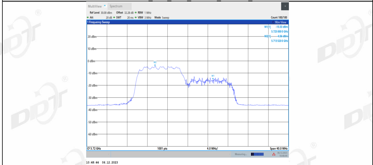
11AX20MIMO_Ant2_5720_UNII-2C_106Tone_RU54
