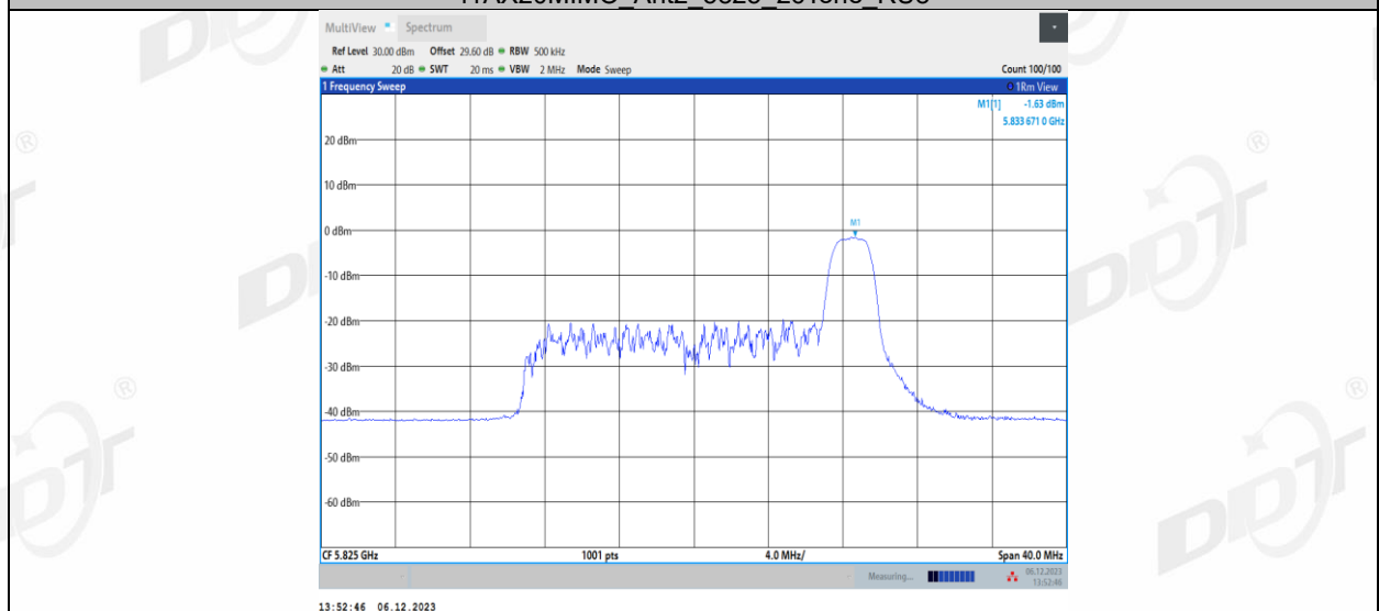
11AX20MIMO_Ant2_5825_52Tone_RU37
