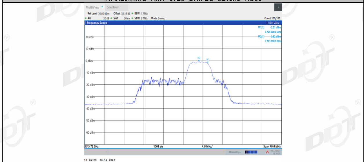
11AX20MIMO_Ant1_5720_UNII-2C_52Tone_RU40
