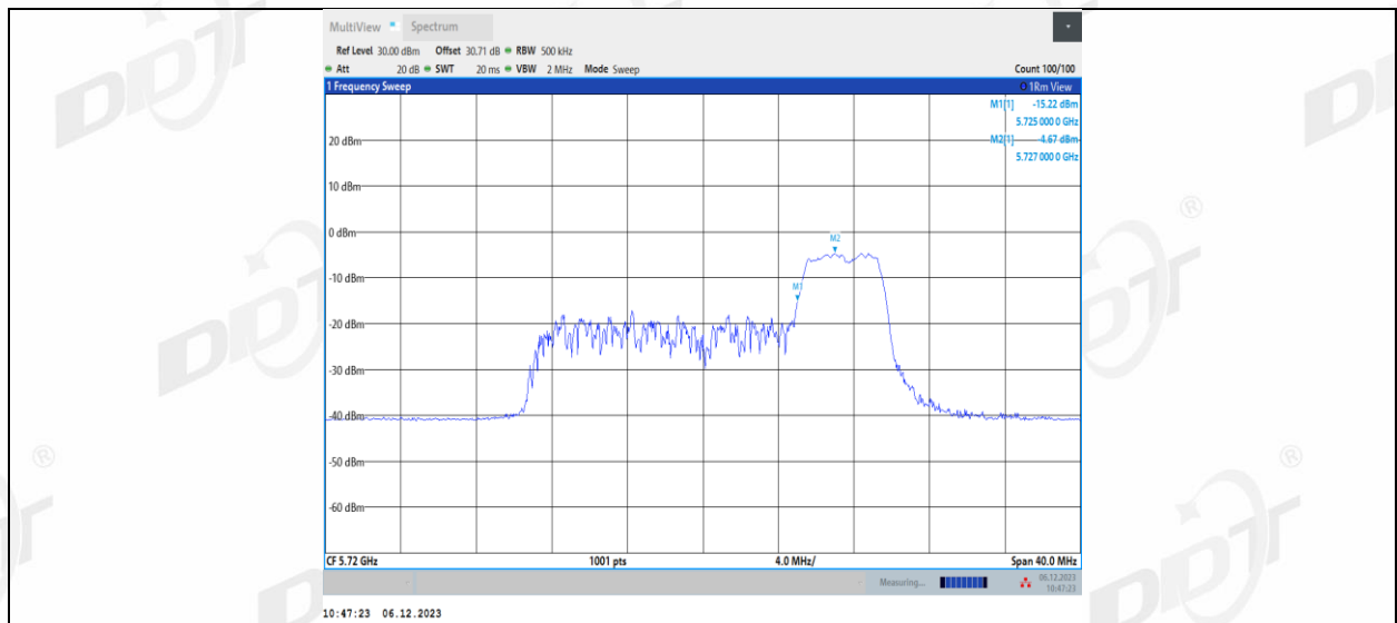
11AX20MIMO_Ant2_5720_UNII-3_106Tone_RU53
