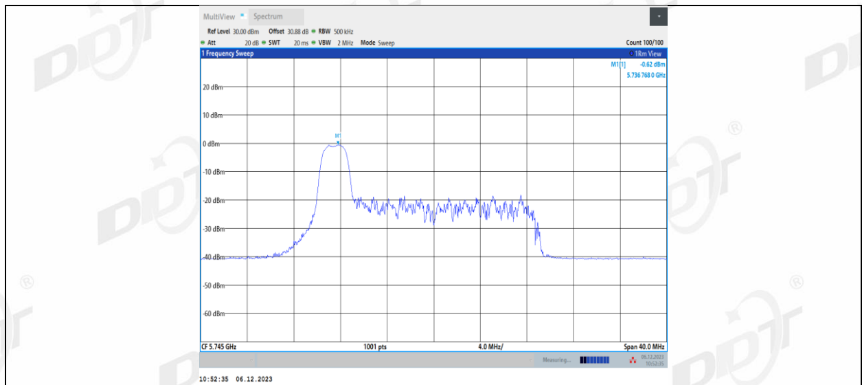
11AX20MIMO_Ant1_5745_26Tone_RU4
