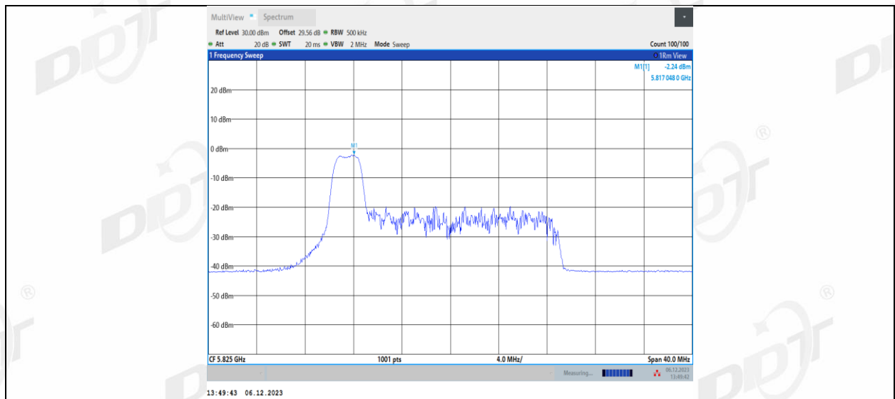
11AX20MIMO_Ant2_5825_26Tone_RU4
