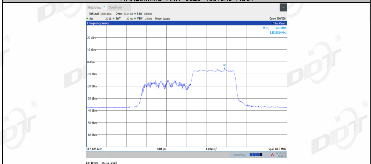
11AX20MIMO_Ant2_5825_26Tone_RU0
