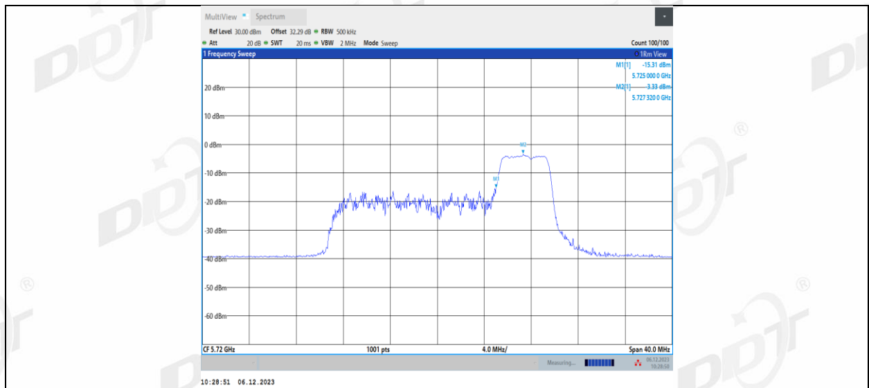
11AX20MIMO_Ant1_5720_UNII-3_106Tone_RU53
