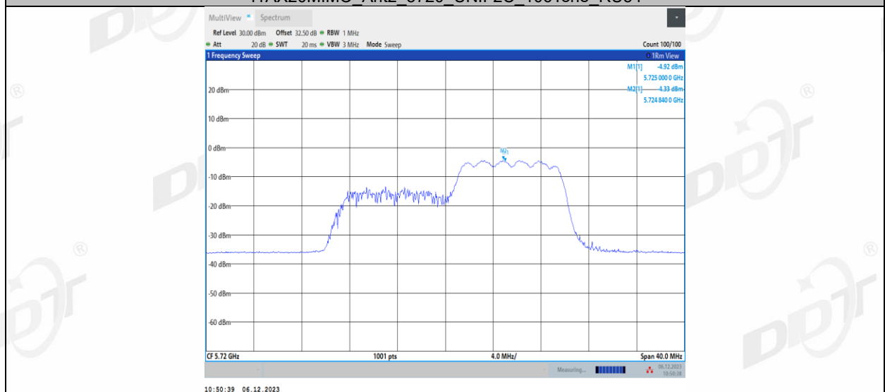
11AX20MIMO_Ant1_5720_UNII-3_26Tone_RU0
