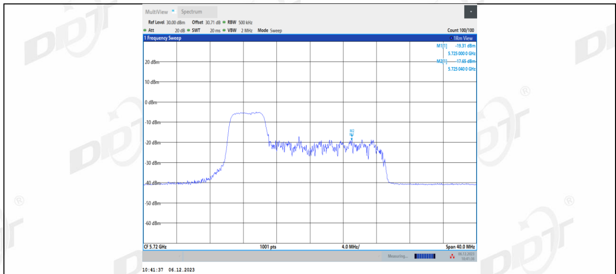
11AX20MIMO_Ant2_5720_UNII-3_52Tone_RU38
