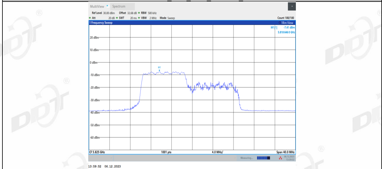
11AX20MIMO_Ant2_5825_106Tone_RU54
