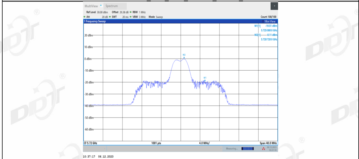
11AX20MIMO_Ant2_5720_UNII-2C_26Tone_RU8
