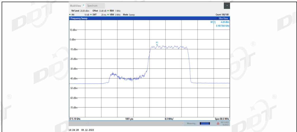
11AX40MIMO_Ant2_5190_106Tone_RU55
