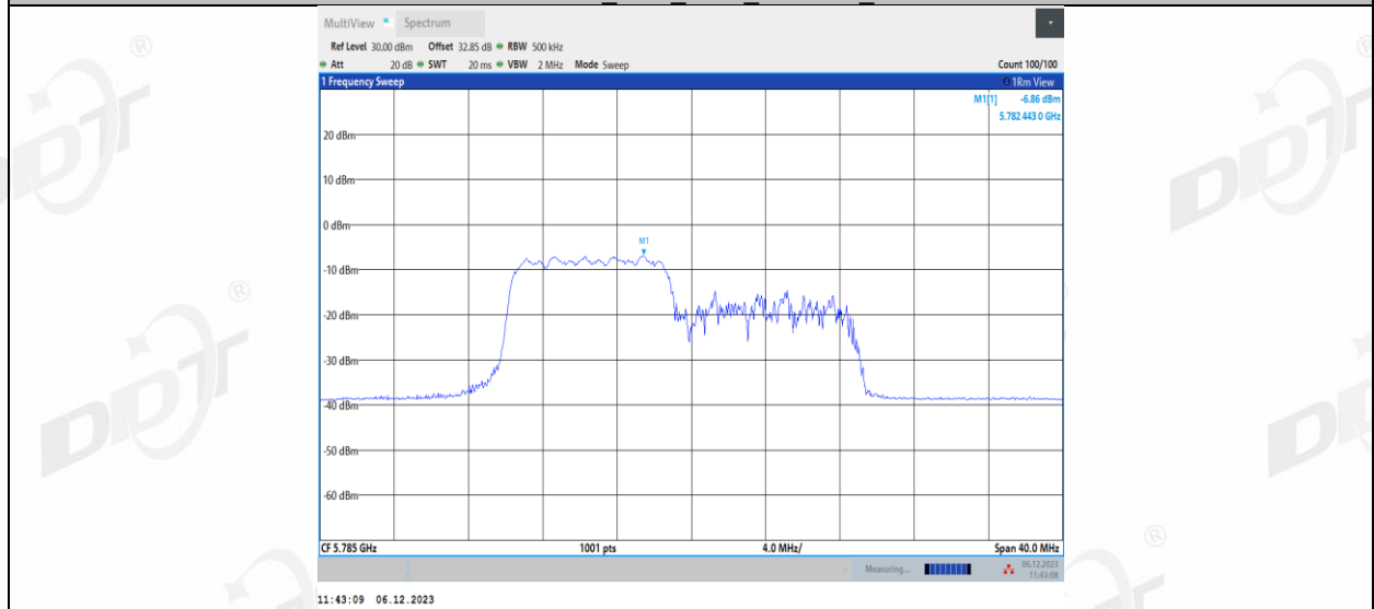
11AX20MIMO_Ant2_5785_106Tone_RU54
