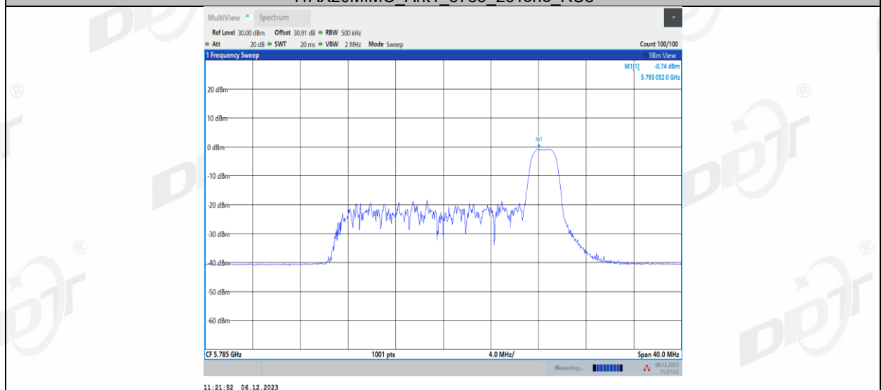
11AX20MIMO_Ant1_5785_52Tone_RU37
