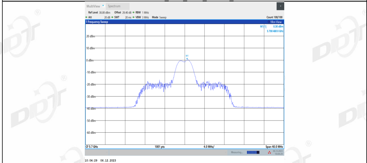
11AX20MIMO_Ant2_5700_26Tone_RU8
