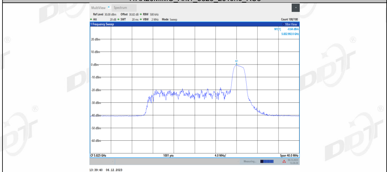
11AX20MIMO_Ant1_5825_52Tone_RU37
