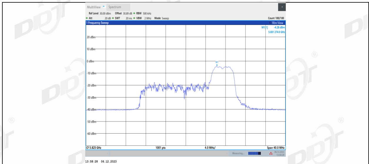
11AX20MIMO_Ant2_5825_106Tone_RU53
