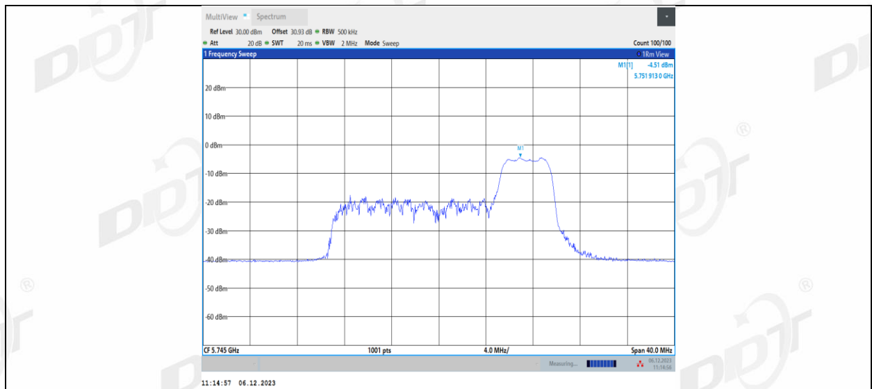
11AX20MIMO_Ant2_5745_106Tone_RU53
