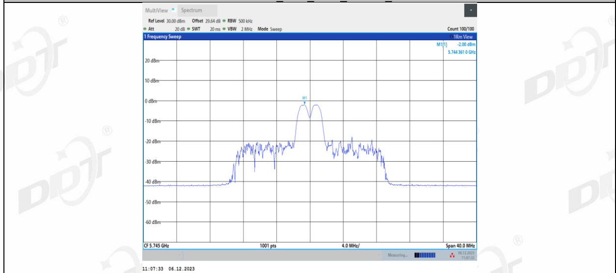
11AX20MIMO_Ant2_5745_26Tone_RU8
