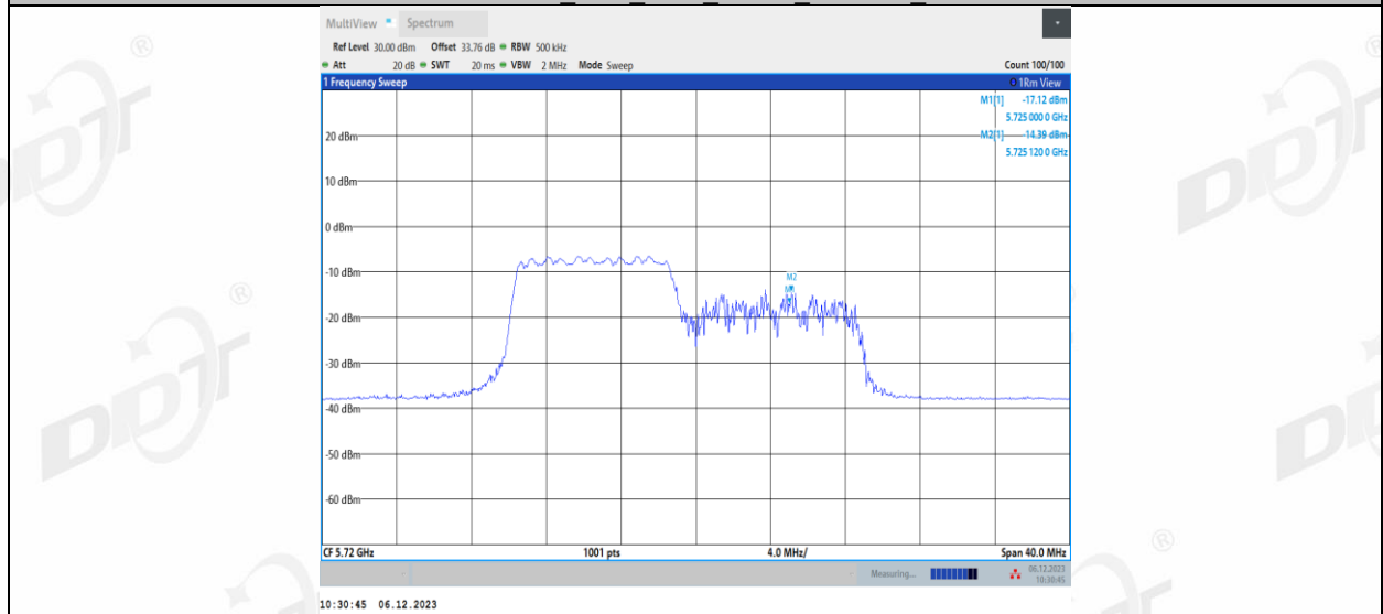
11AX20MIMO_Ant1_5720_UNII-3_106Tone_RU54
