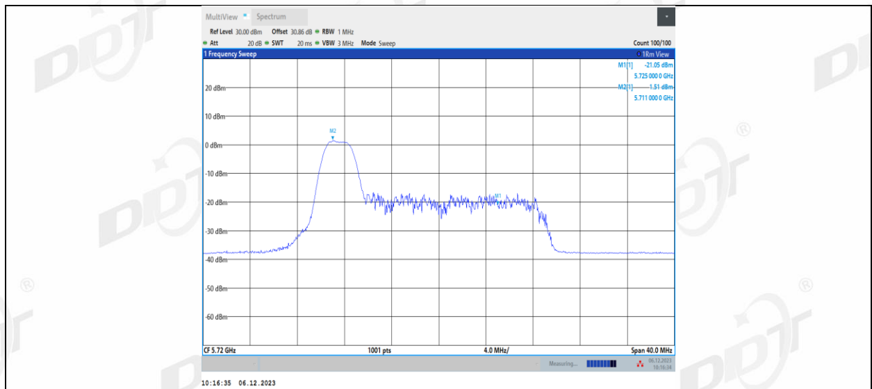
11AX20MIMO_Ant1_5720_UNII-2C_26Tone_RU4
