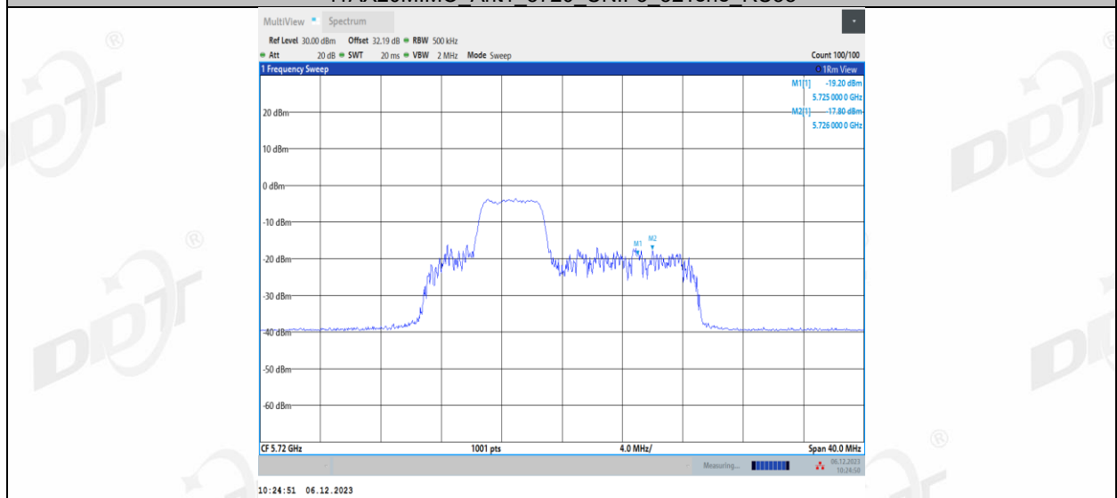
11AX20MIMO_Ant1_5720_UNII-3_52Tone_RU39
