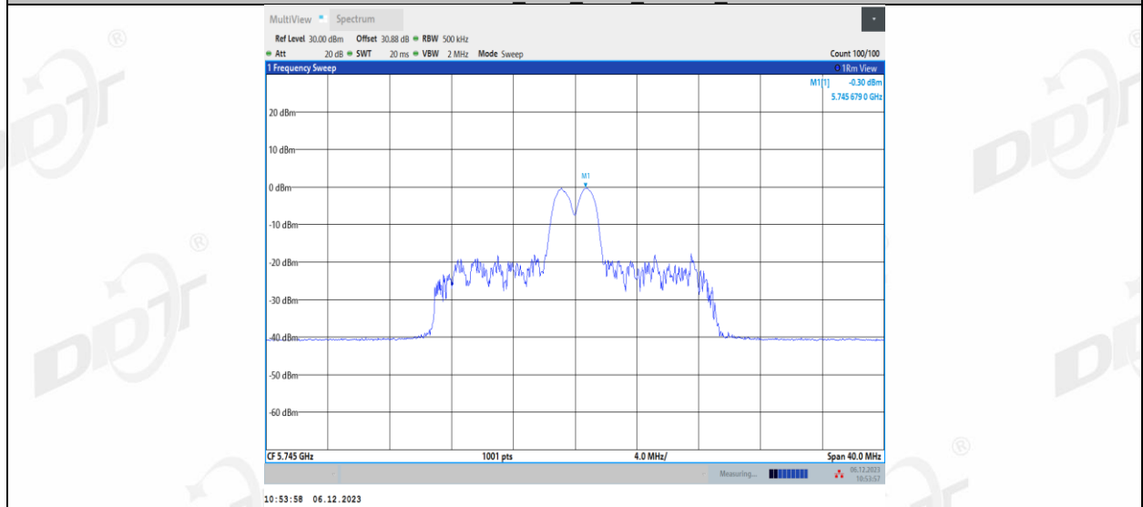
11AX20MIMO_Ant1_5745_26Tone_RU8
