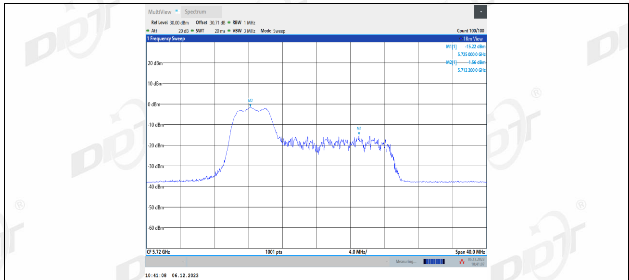
11AX20MIMO_Ant2_5720_UNII-2C_52Tone_RU38
