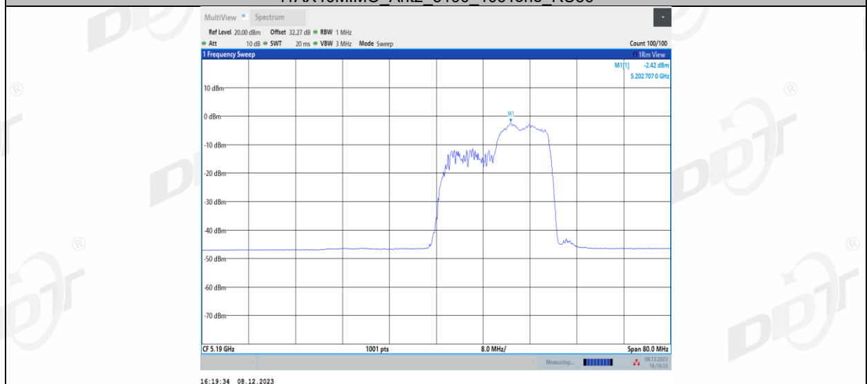
11AX40MIMO_Ant2_5190_242Tone_RU61
