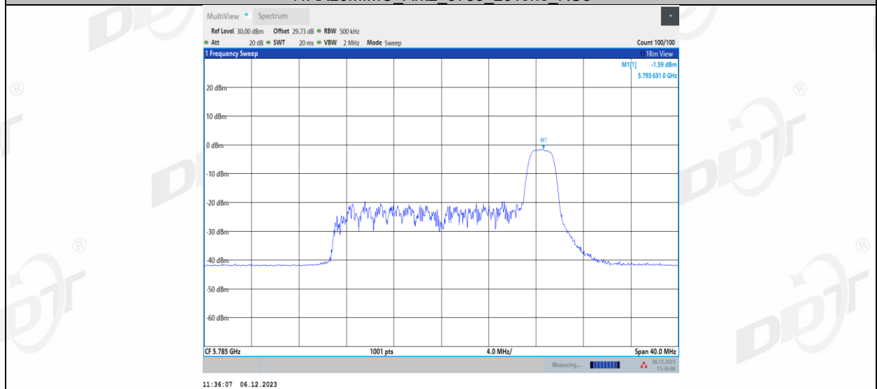
11AX20MIMO_Ant2_5785_52Tone_RU37
