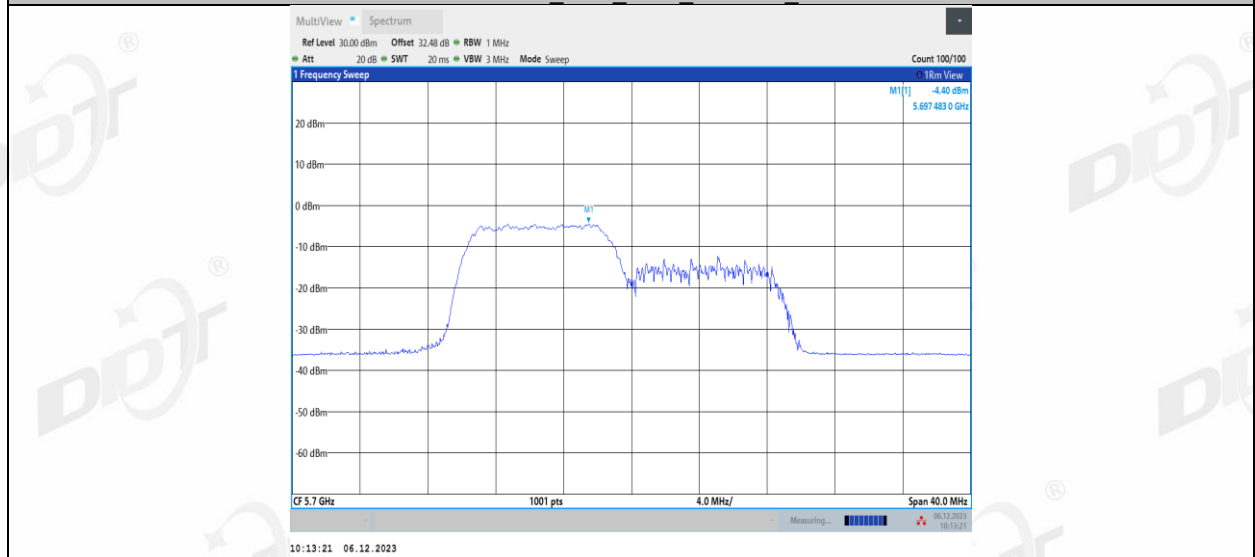
11AX20MIMO_Ant2_5700_106Tone_RU54
