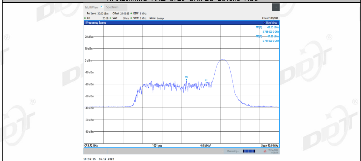
11AX20MIMO_Ant2_5720_UNII-2C_52Tone_RU37
