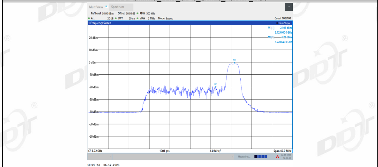
11AX20MIMO_Ant1_5720_UNII-3_52Tone_RU37
