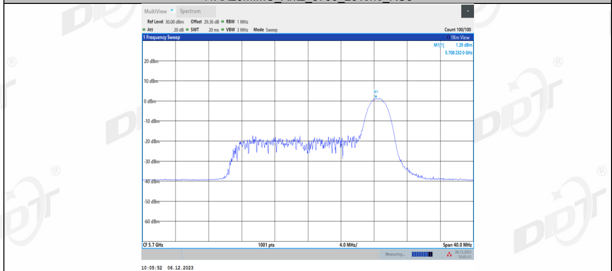
11AX20MIMO_Ant2_5700_52Tone_RU37
