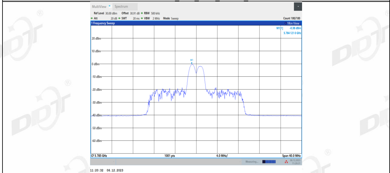
11AX20MIMO_Ant1_5785_26Tone_RU8
