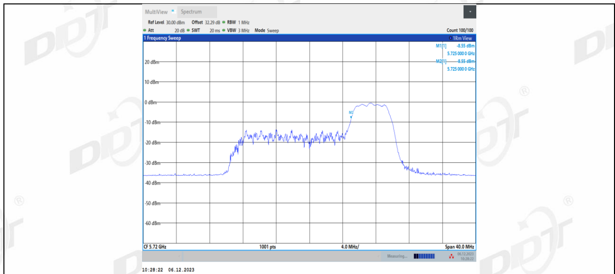
11AX20MIMO_Ant1_5720_UNII-2C_106Tone_RU53
