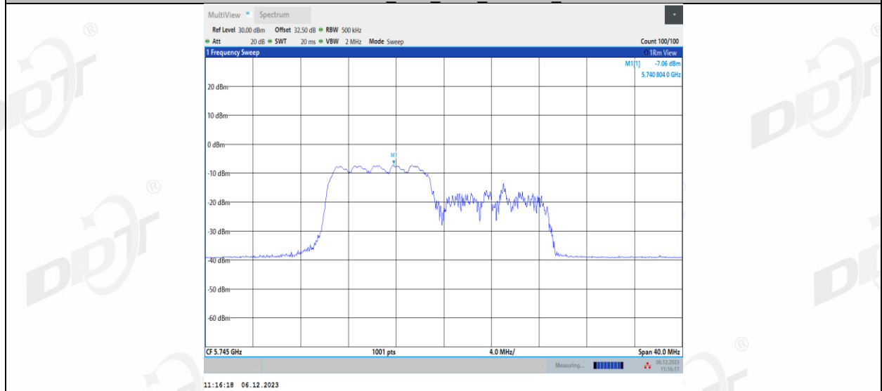
11AX20MIMO_Ant2_5745_106Tone_RU54
