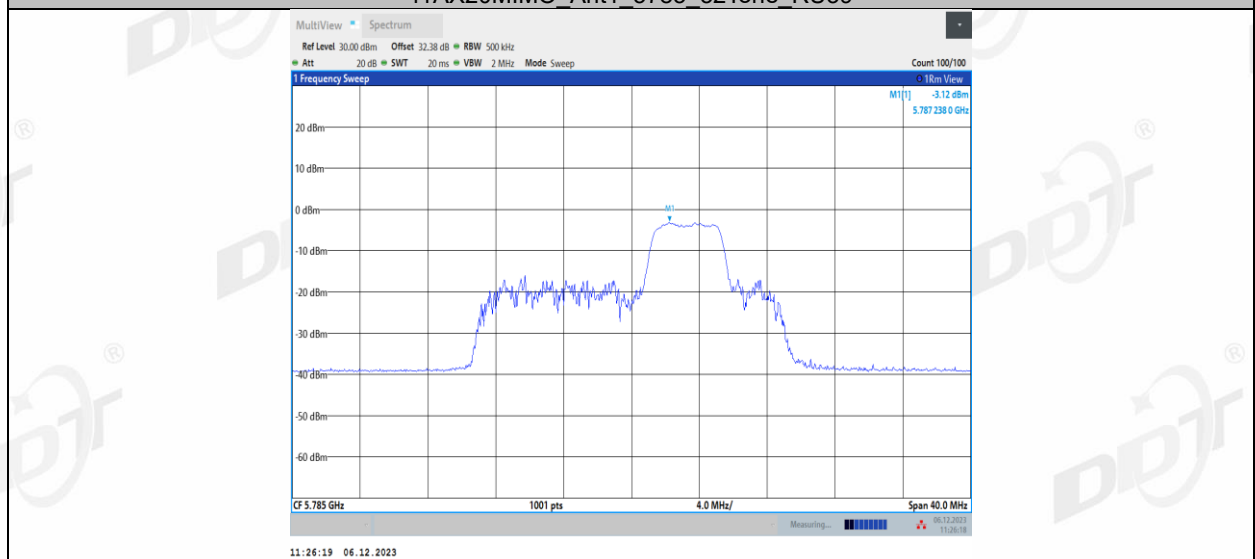
11AX20MIMO_Ant1_5785_52Tone_RU40
