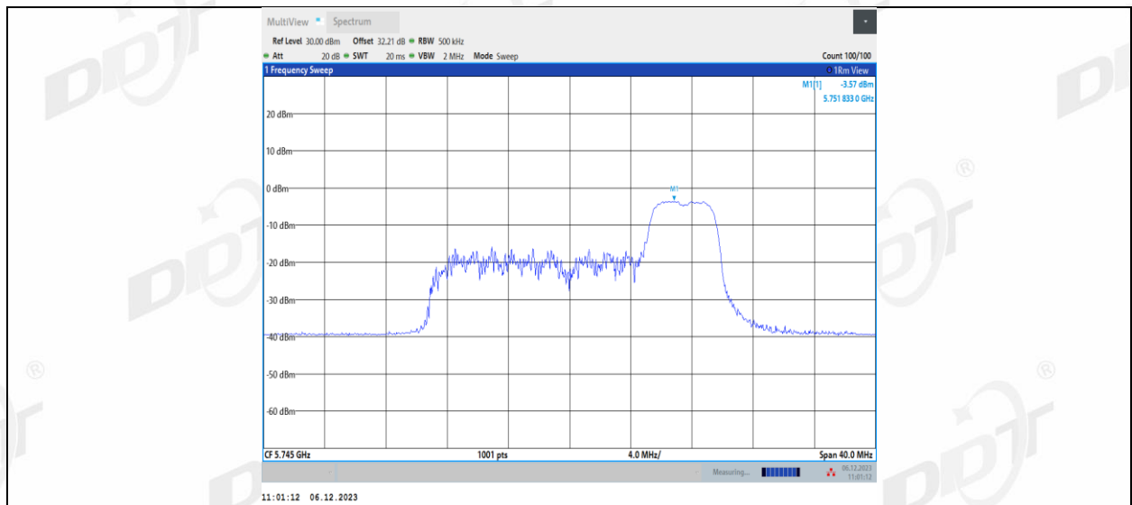
11AX20MIMO_Ant1_5745_106Tone_RU53
