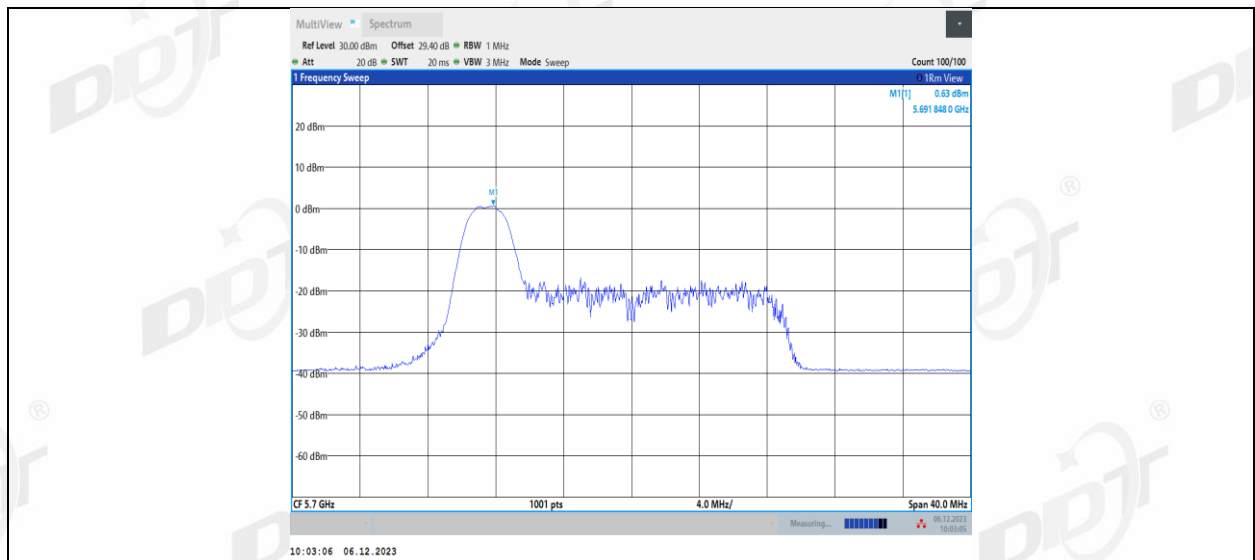
11AX20MIMO_Ant2_5700_26Tone_RU4
