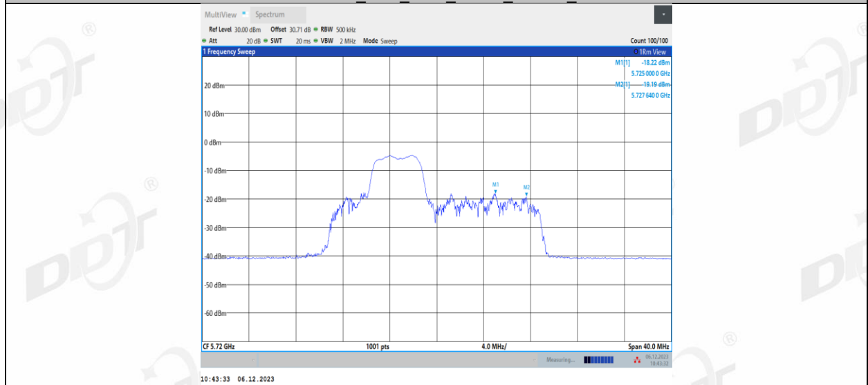
11AX20MIMO_Ant2_5720_UNII-3_52Tone_RU39
