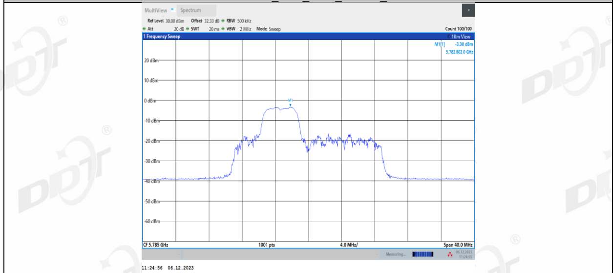
11AX20MIMO_Ant1_5785_52Tone_RU39
