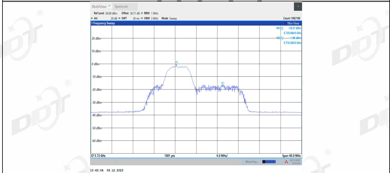
11AX20MIMO_Ant2_5720_UNII-2C_52Tone_RU39
