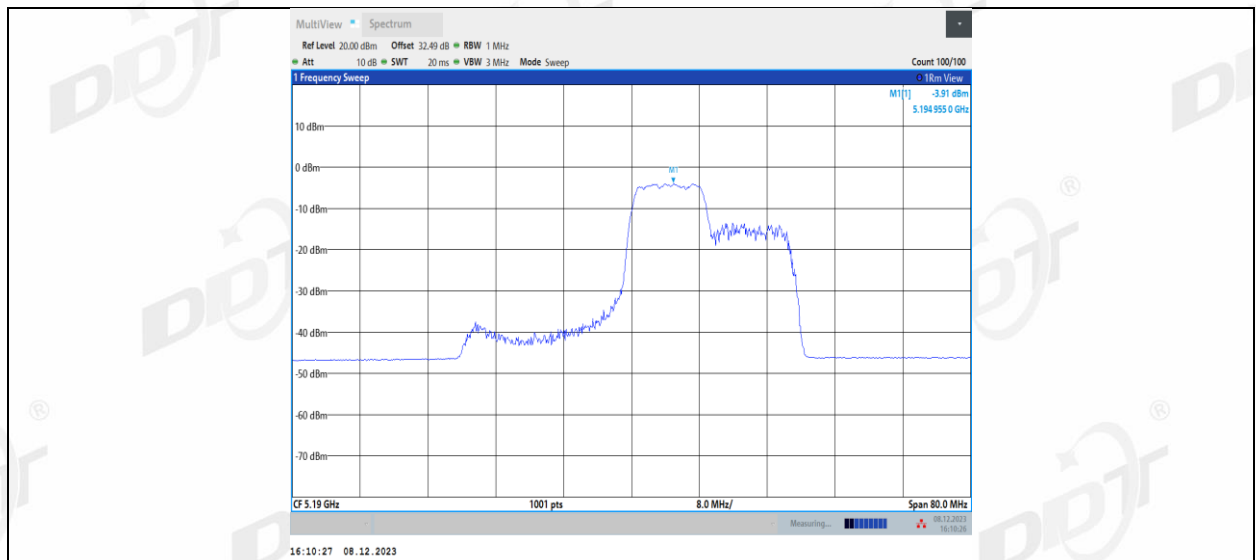
11AX40MIMO_Ant1_5190_106Tone_RU56
