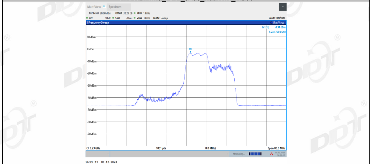
11AX40MIMO_Ant1_5230_106Tone_RU56
