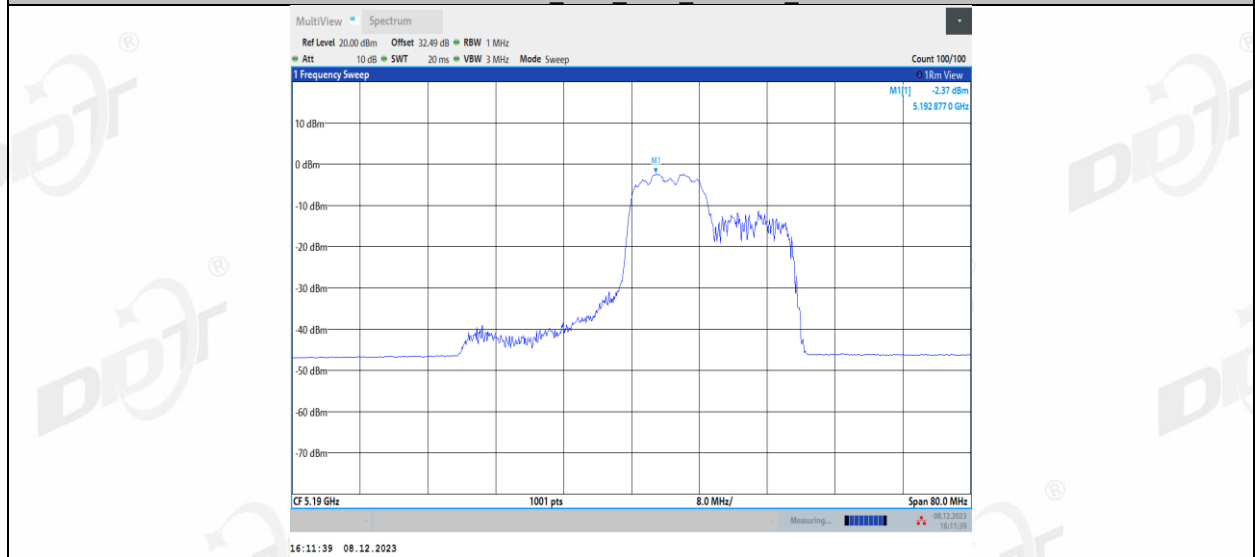
11AX40MIMO_Ant2_5190_106Tone_RU56
