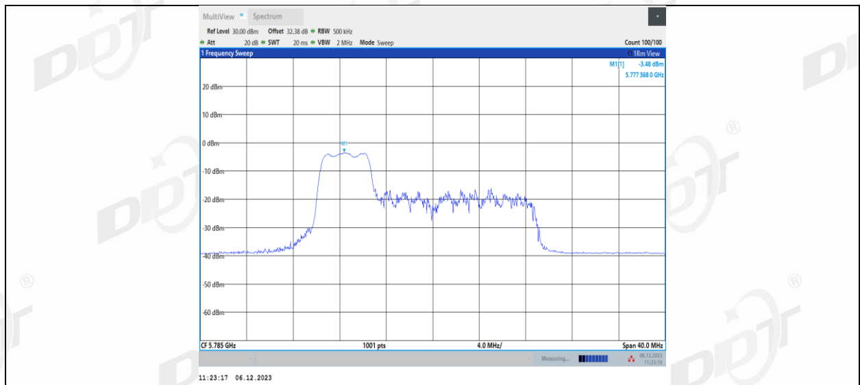
11AX20MIMO_Ant1_5785_52Tone_RU38
