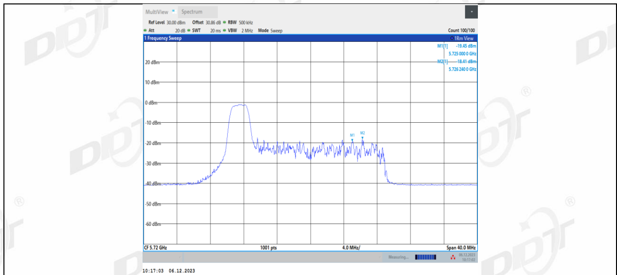
11AX20MIMO_Ant1_5720_UNII-3_26Tone_RU4
