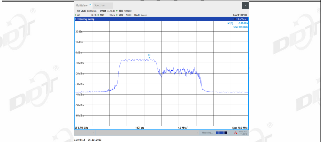
11AX20MIMO_Ant1_5745_106Tone_RU54
