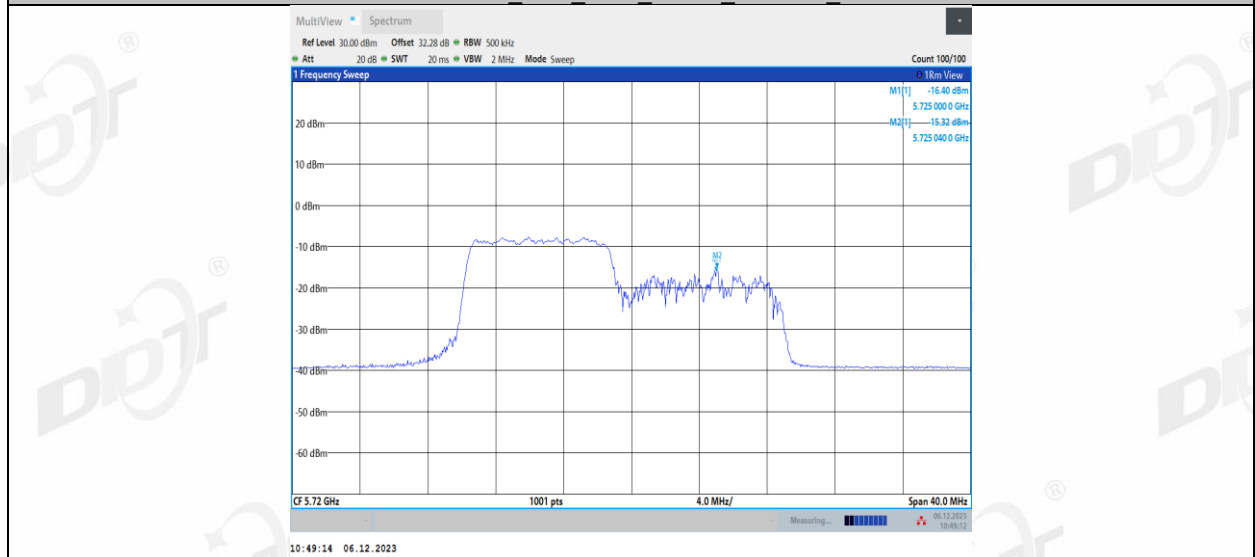
11AX20MIMO_Ant2_5720_UNII-3_106Tone_RU54
