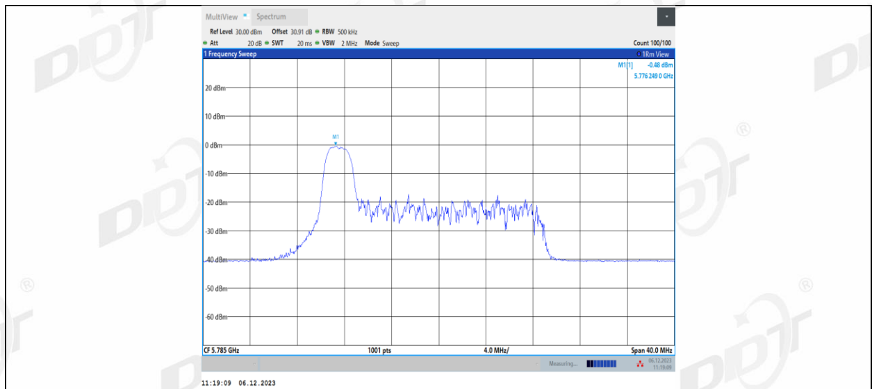
11AX20MIMO_Ant1_5785_26Tone_RU4
