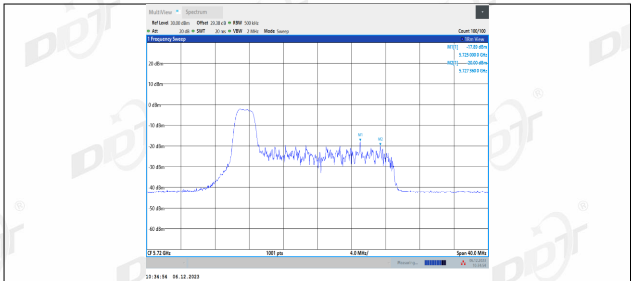
11AX20MIMO_Ant2_5720_UNII-3_26Tone_RU4
