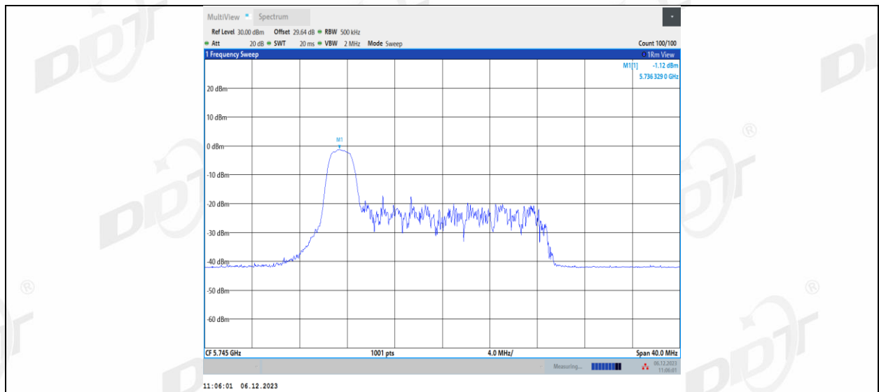
11AX20MIMO_Ant2_5745_26Tone_RU4
