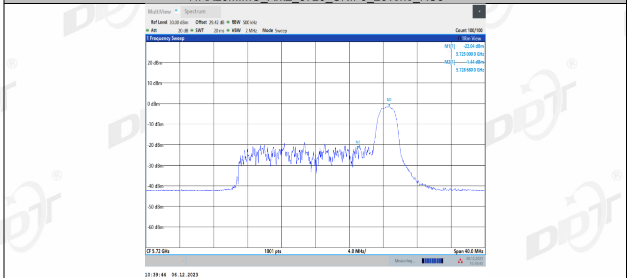
11AX20MIMO_Ant2_5720_UNII-3_52Tone_RU37
