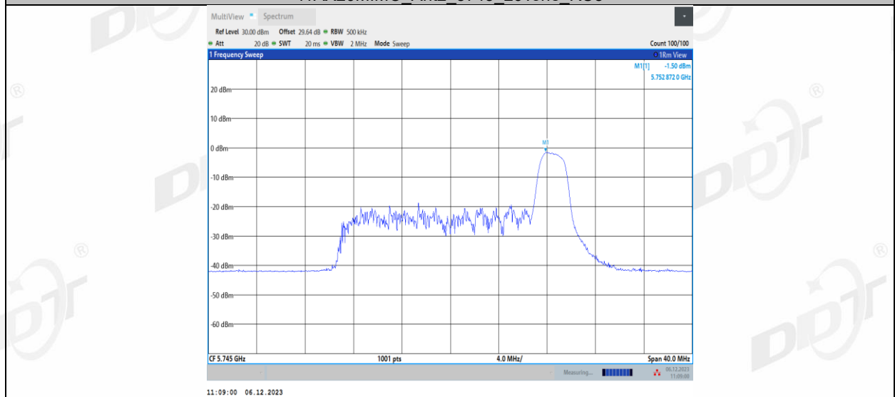
11AX20MIMO_Ant2_5745_52Tone_RU37
