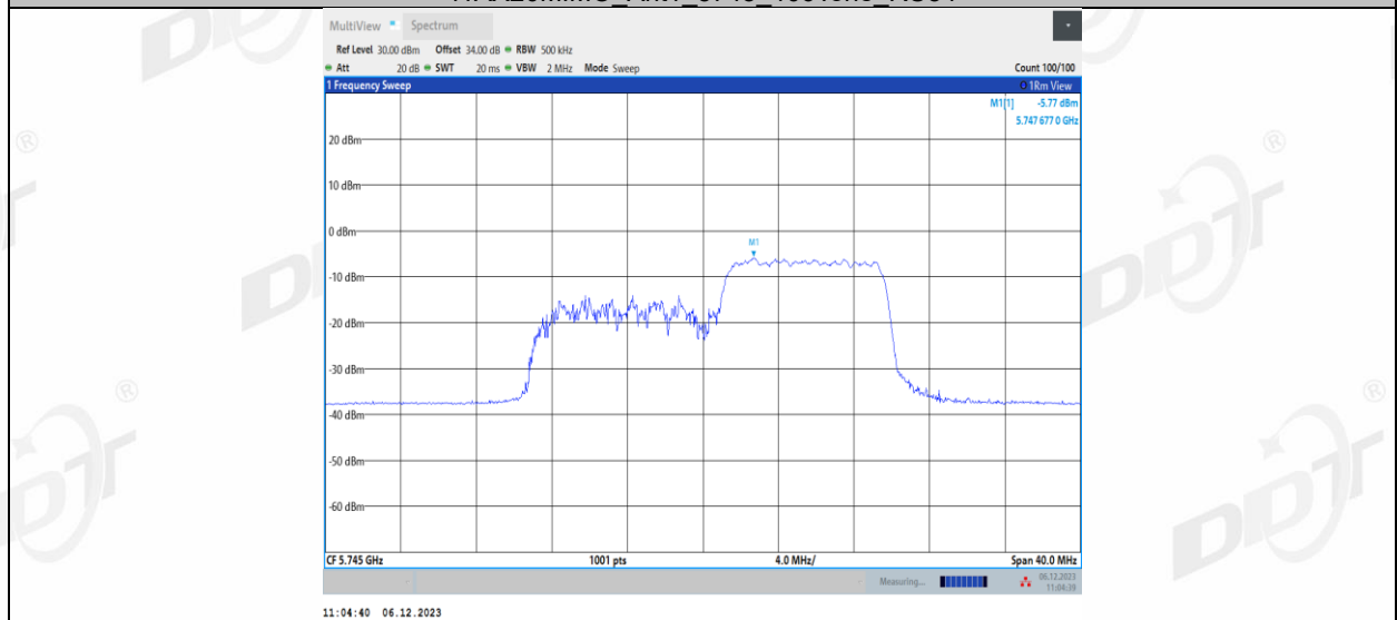
11AX20MIMO_Ant2_5745_26Tone_RU0
