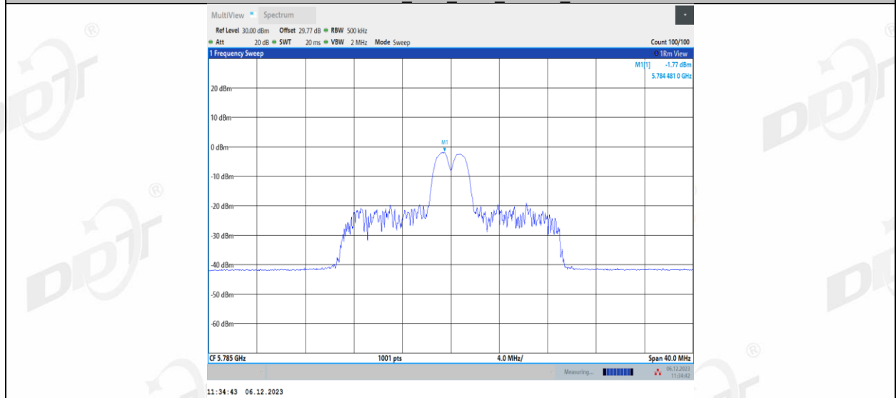
11AX20MIMO_Ant2_5785_26Tone_RU8
