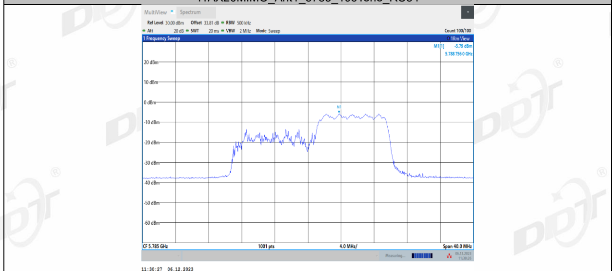
11AX20MIMO_Ant2_5785_26Tone_RU0
