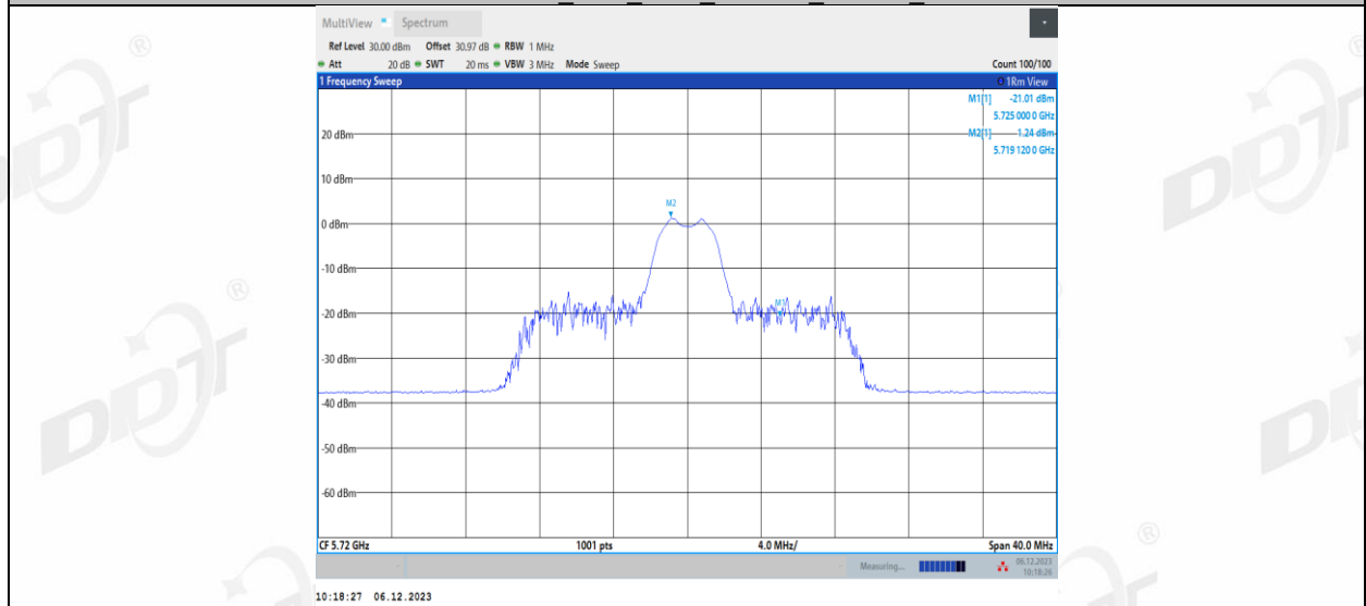
11AX20MIMO_Ant1_5720_UNII-2C_26Tone_RU8
