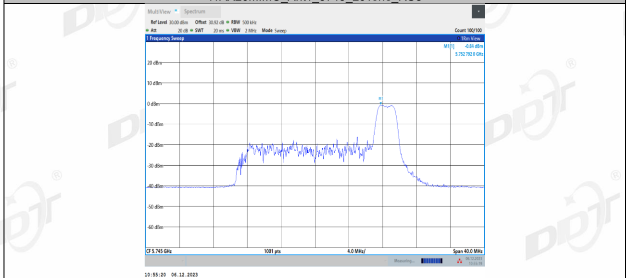
11AX20MIMO_Ant1_5745_52Tone_RU37
