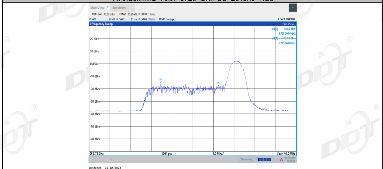
11AX20MIMO_Ant1_5720_UNII-2C_52Tone_RU37
