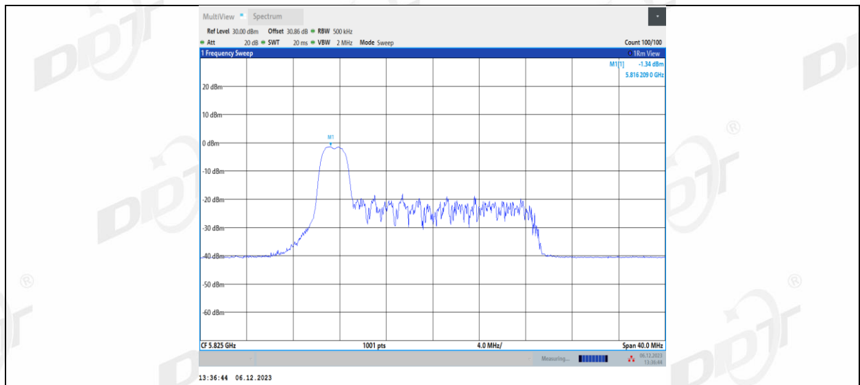
11AX20MIMO_Ant1_5825_26Tone_RU4
