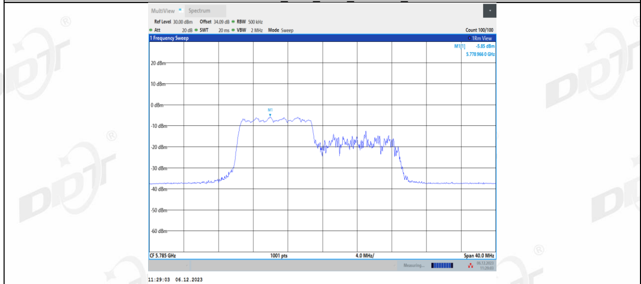
11AX20MIMO_Ant1_5785_106Tone_RU54
