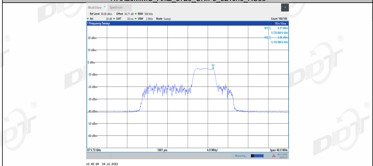
11AX20MIMO_Ant2_5720_UNII-3_52Tone_RU40
