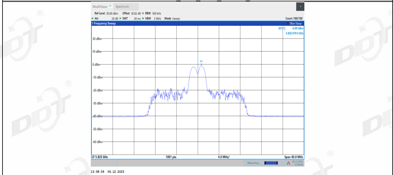
11AX20MIMO_Ant1_5825_26Tone_RU8
