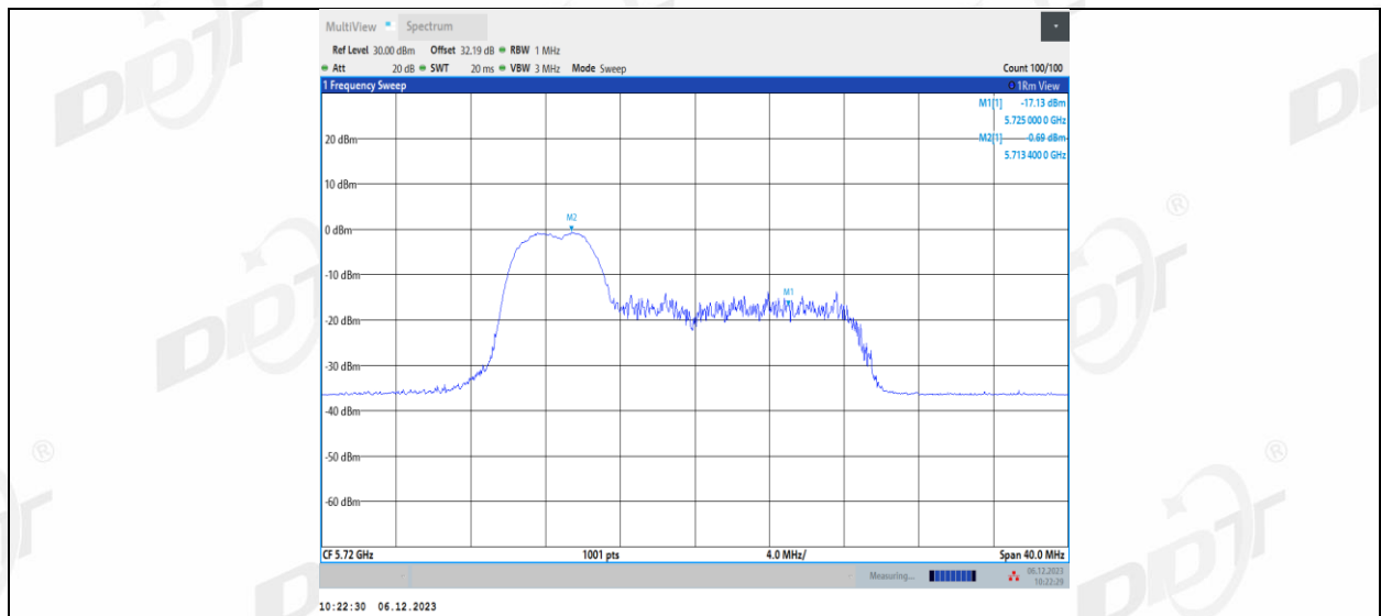
11AX20MIMO_Ant1_5720_UNII-2C_52Tone_RU38
