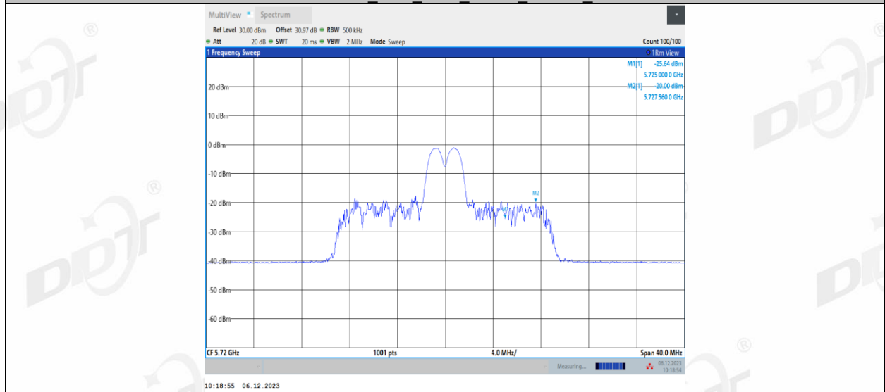
11AX20MIMO_Ant1_5720_UNII-3_26Tone_RU8
