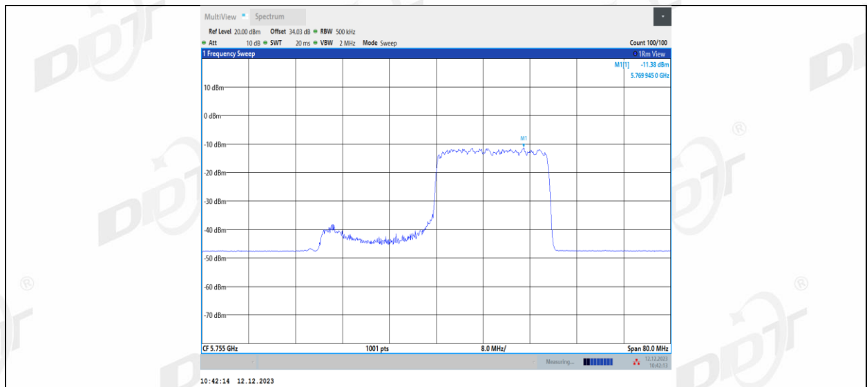
11AX40MIMO_Ant2_5755_106Tone_RU55
