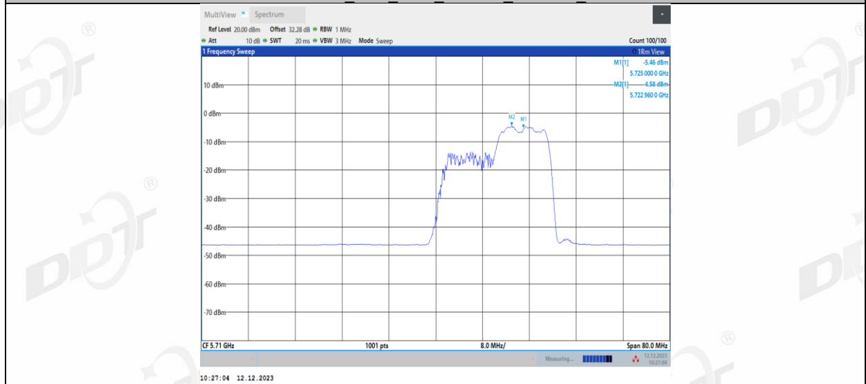
11AX40MIMO_Ant2_5710_UNII-2C_242Tone_RU61
