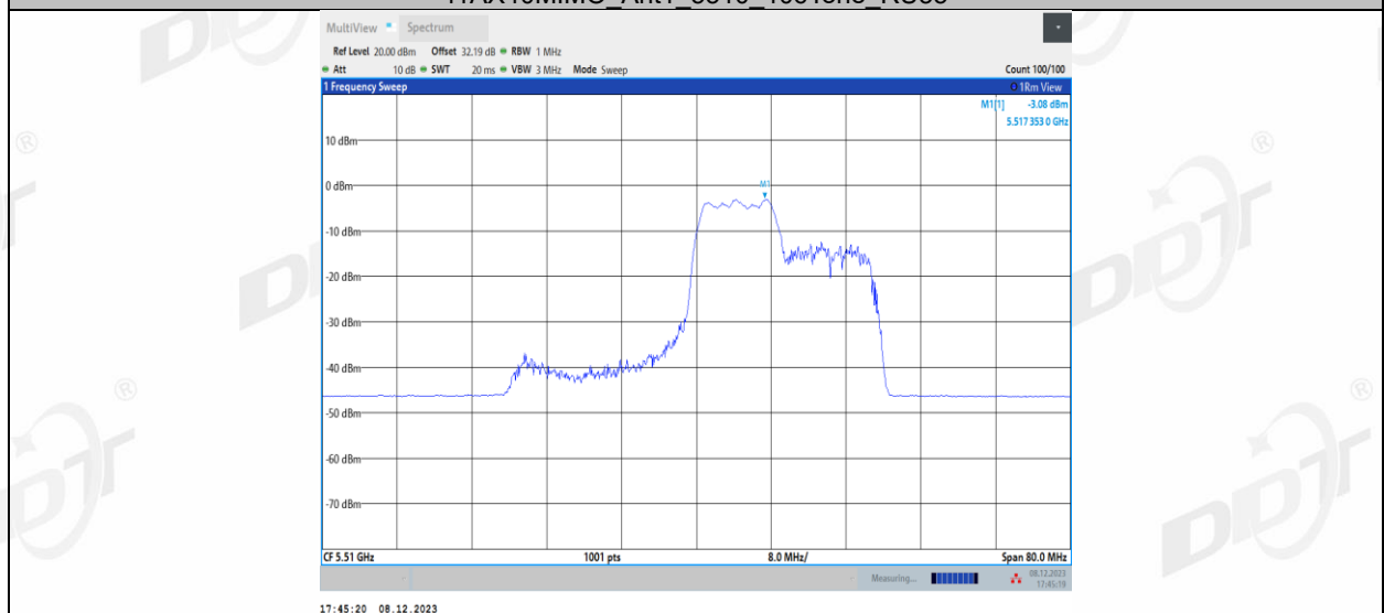
11AX40MIMO_Ant1_5510_106Tone_RU56
