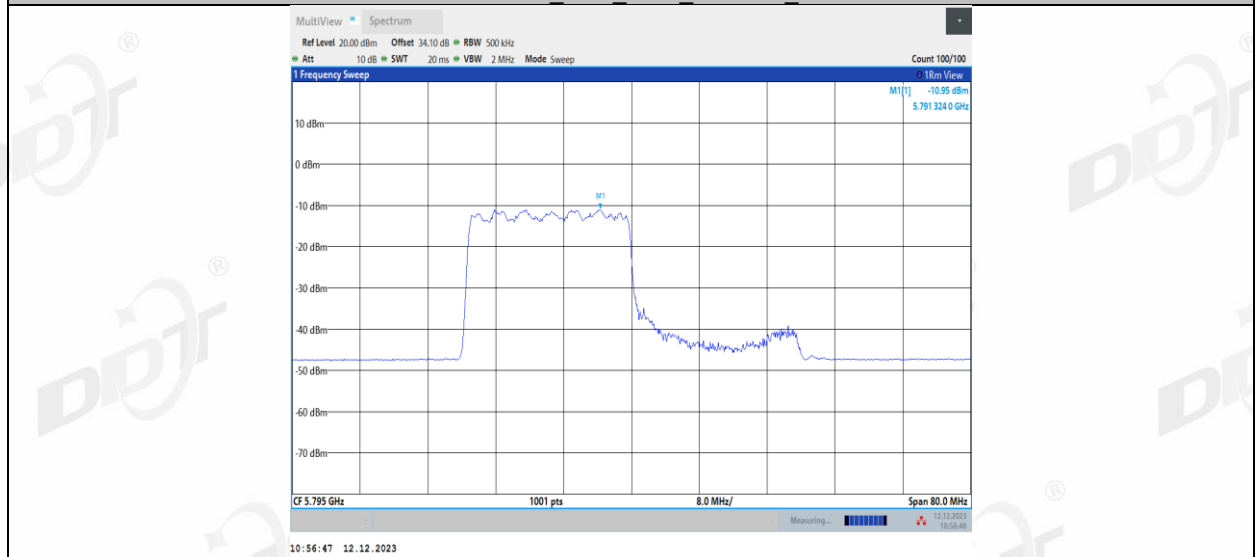
11AX40MIMO_Ant1_5795_242Tone_RU62
