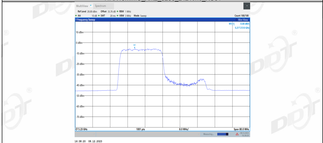
11AX40MIMO_Ant2_5230_242Tone_RU62
