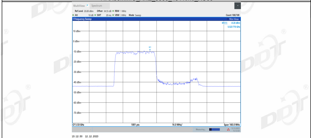
11AX80MIMO_Ant2_5530_484Tone_RU66
