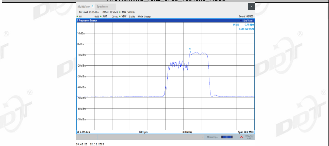
11AX40MIMO_Ant2_5755_242Tone_RU61
