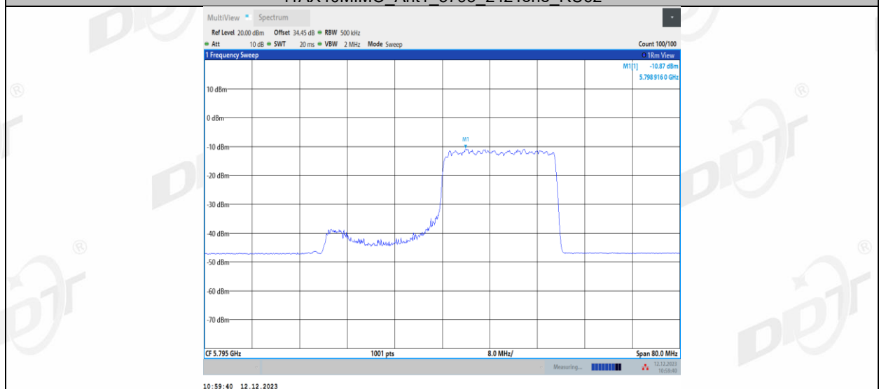
11AX40MIMO_Ant2_5795_106Tone_RU55
