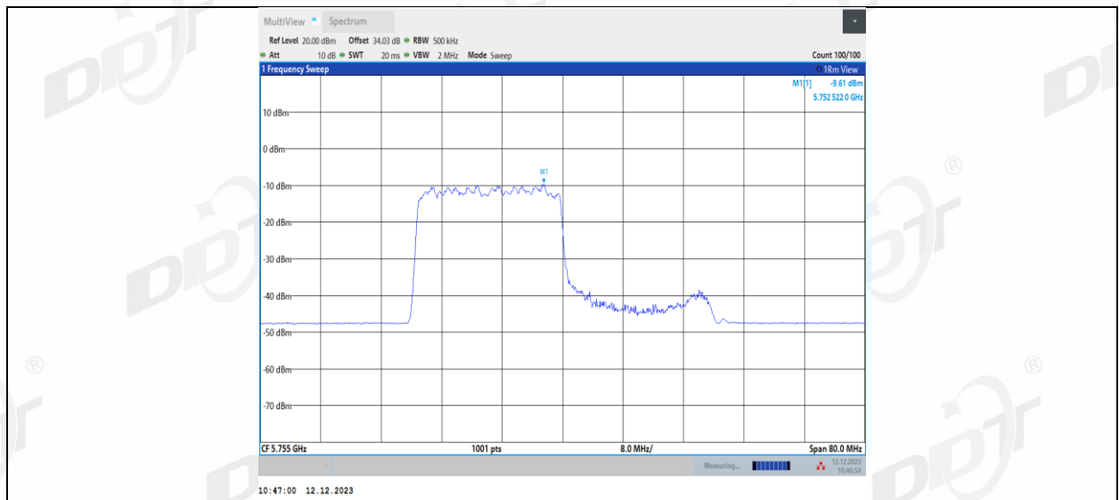
11AX40MIMO_Ant2_5755_242Tone_RU62
