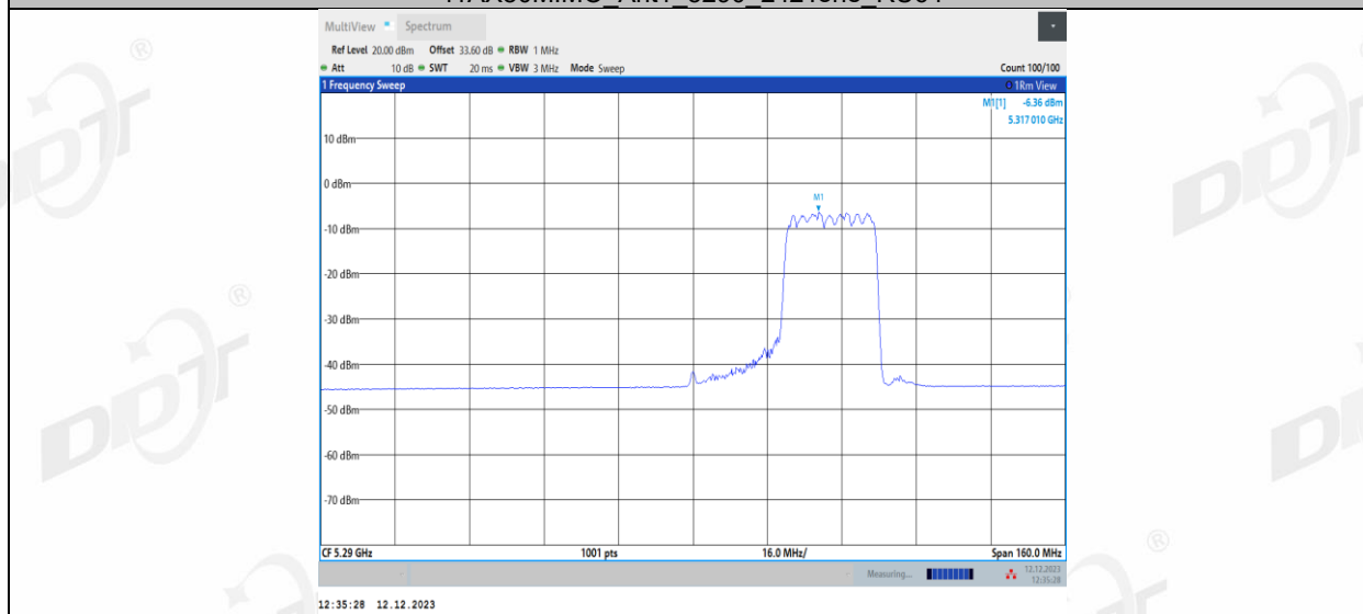
11AX80MIMO_Ant1_5290_484Tone_RU65
