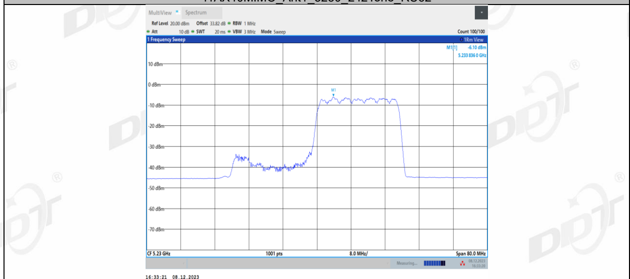
11AX40MIMO_Ant2_5230_106Tone_RU55
