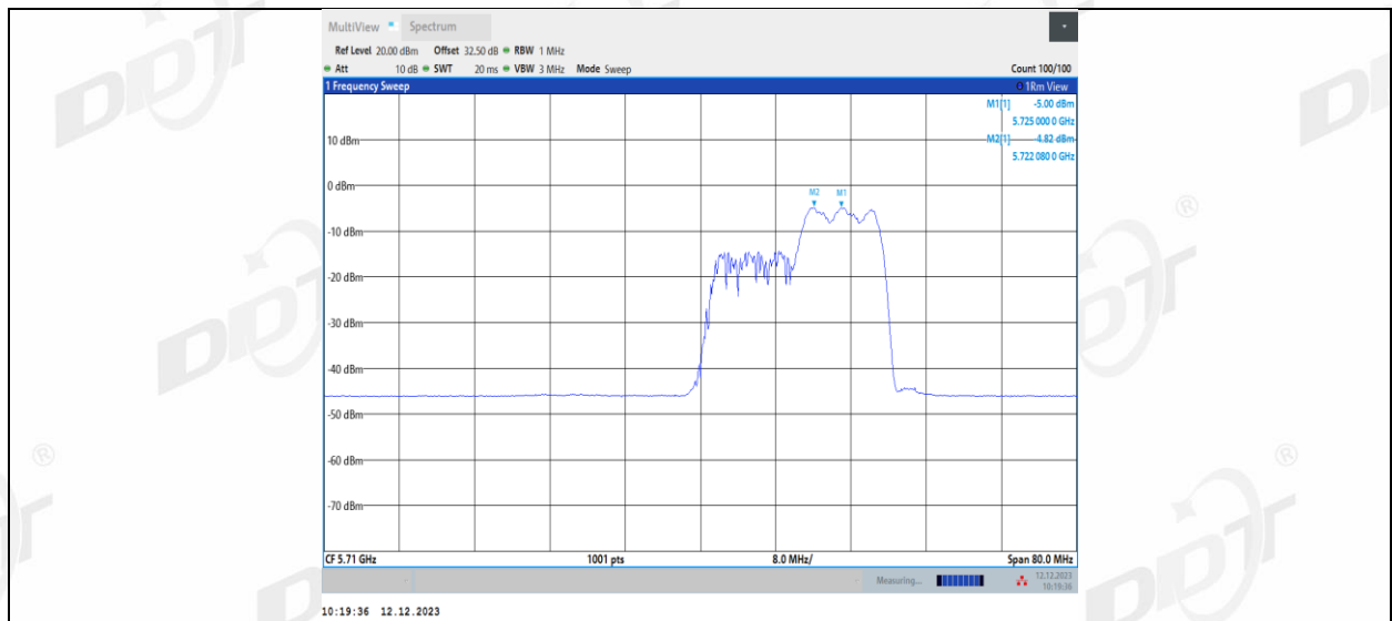
11AX40MIMO_Ant1_5710_UNII-2C_242Tone_RU61
