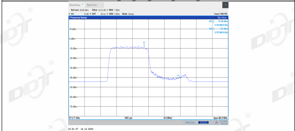
11AX40MIMO_Ant1_5710_UNII-2C_242Tone_RU62
