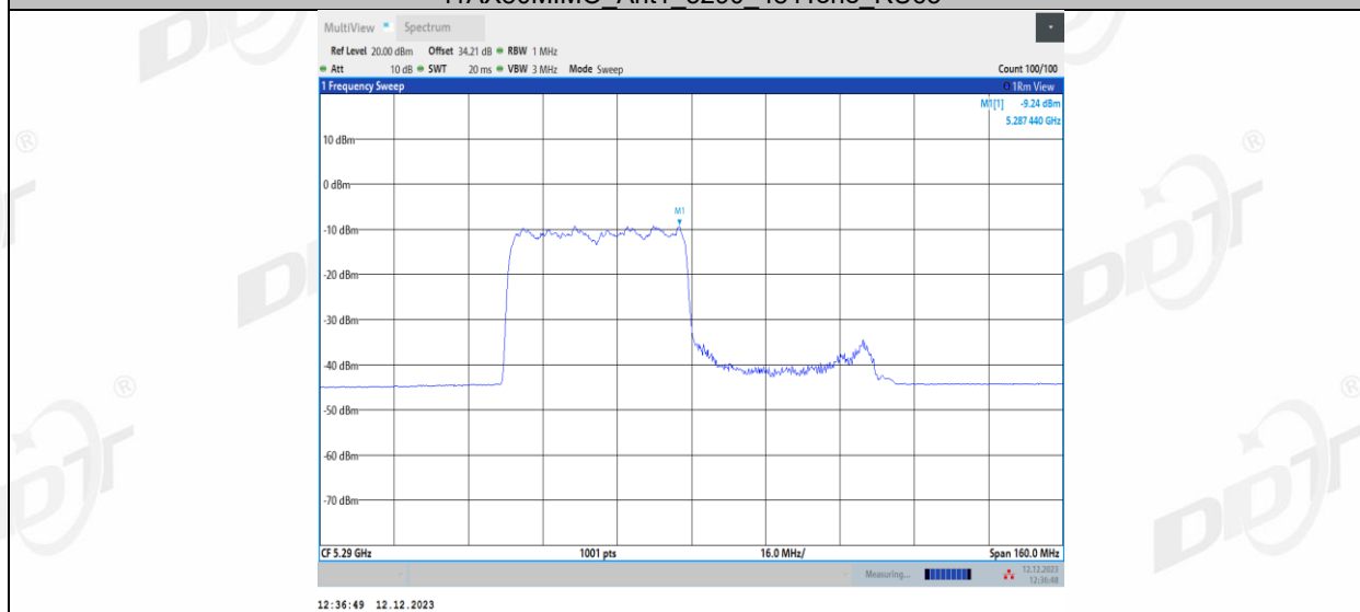
11AX80MIMO_Ant1_5290_484Tone_RU66
