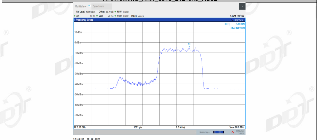
11AX40MIMO_Ant2_5510_106Tone_RU55
