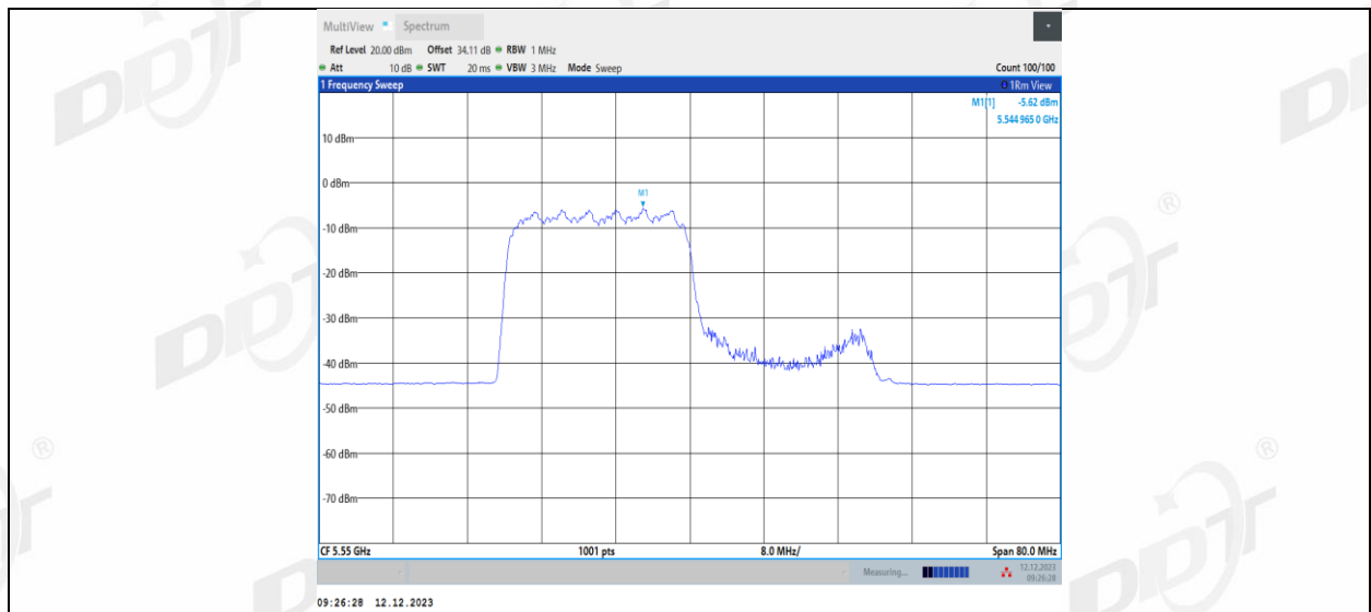
11AX40MIMO_Ant1_5550_242Tone_RU62
