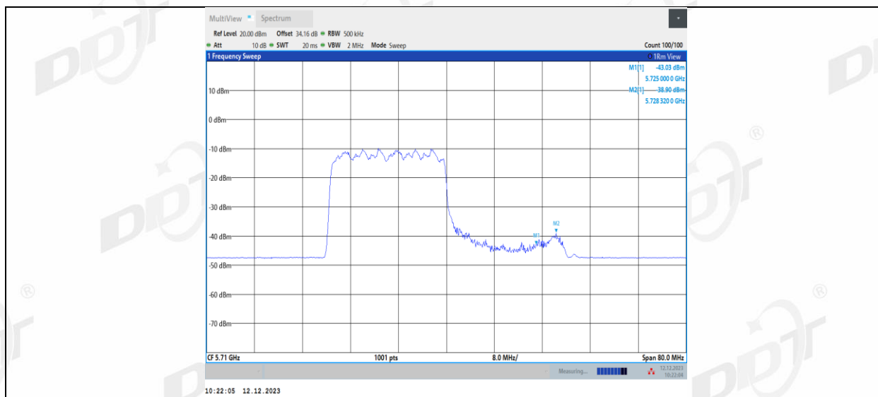
11AX40MIMO_Ant1_5710_UNII-3_242Tone_RU62
