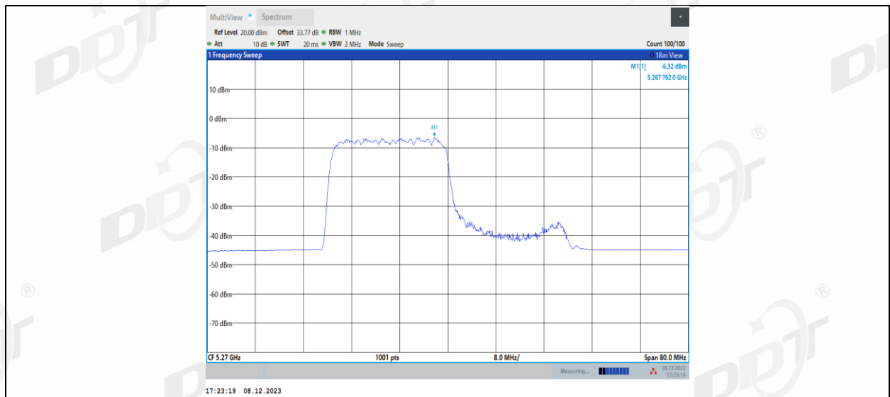
11AX40MIMO_Ant1_5270_242Tone_RU62
