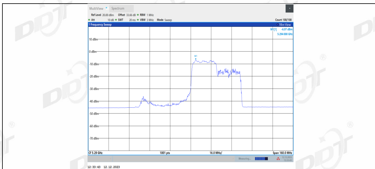
11AX80MIMO_Ant1_5290_242Tone_RU64
