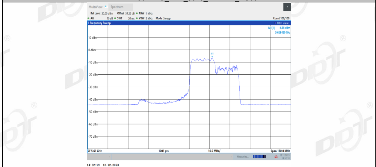
11AX80MIMO_Ant2_5610_242Tone_RU64
