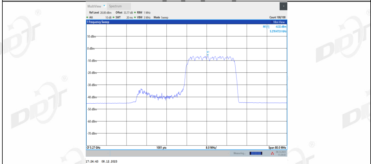
11AX40MIMO_Ant2_5270_106Tone_RU55
