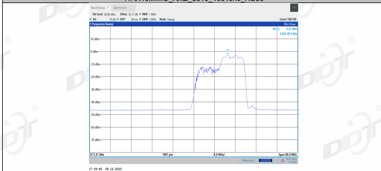
11AX40MIMO_Ant2_5310_242Tone_RU61
