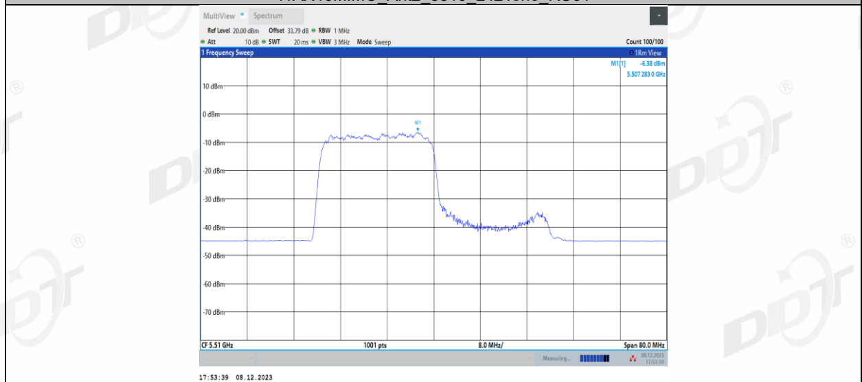
11AX40MIMO_Ant2_5510_242Tone_RU62
