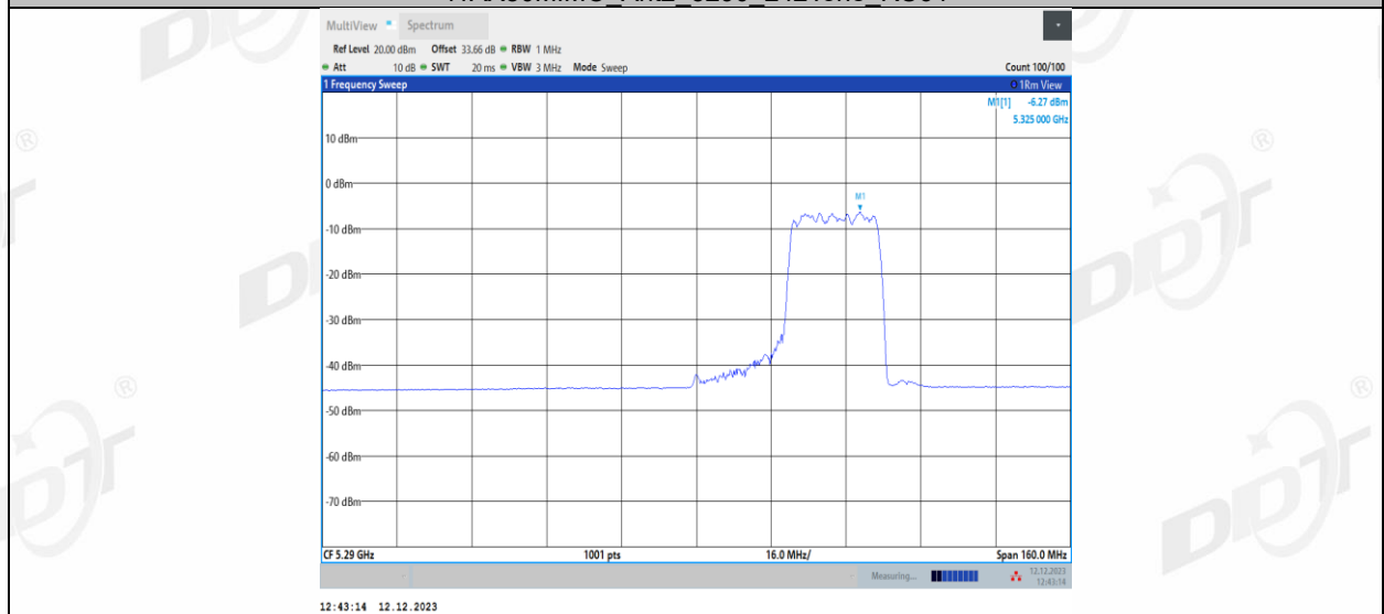
11AX80MIMO_Ant2_5290_484Tone_RU65
