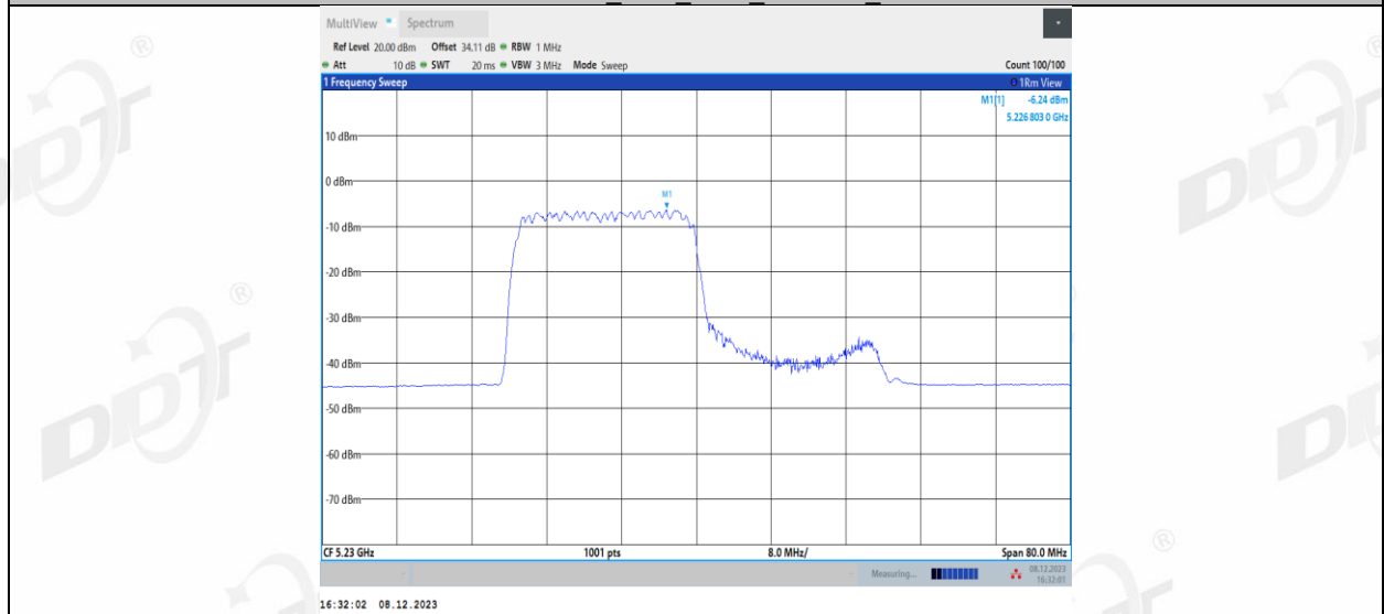
11AX40MIMO_Ant1_5230_242Tone_RU62
