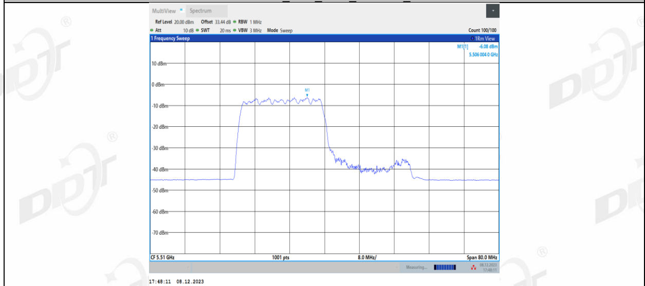
11AX40MIMO_Ant1_5510_242Tone_RU62
