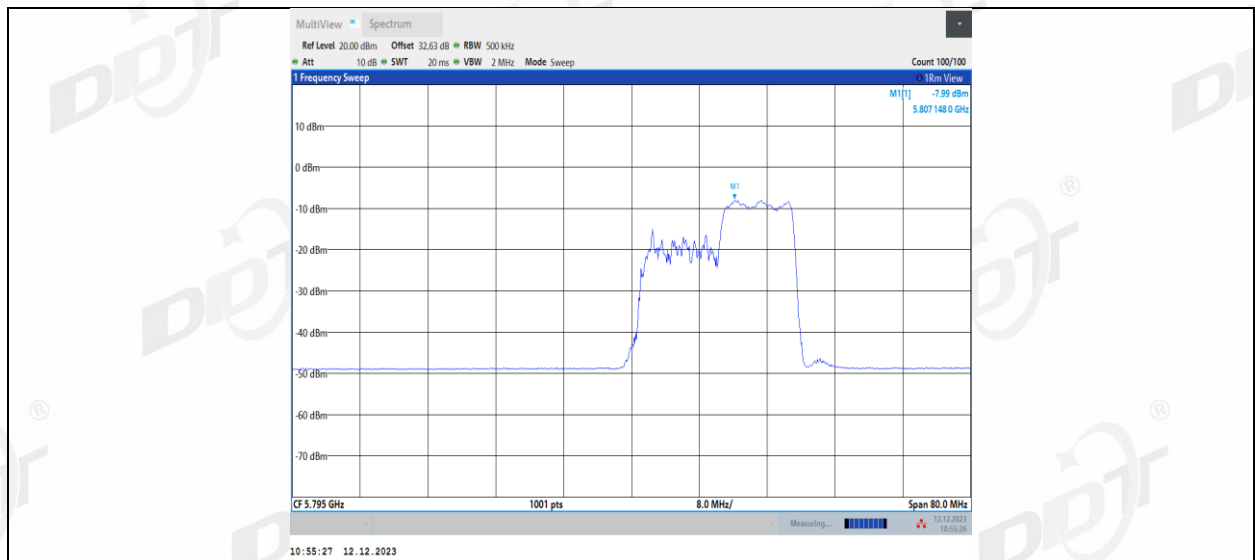
11AX40MIMO_Ant1_5795_242Tone_RU61
