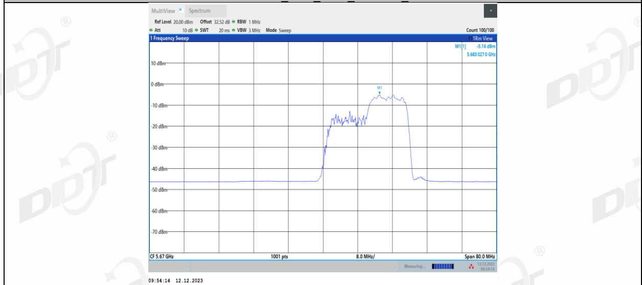
11AX40MIMO_Ant1_5670_242Tone_RU61
