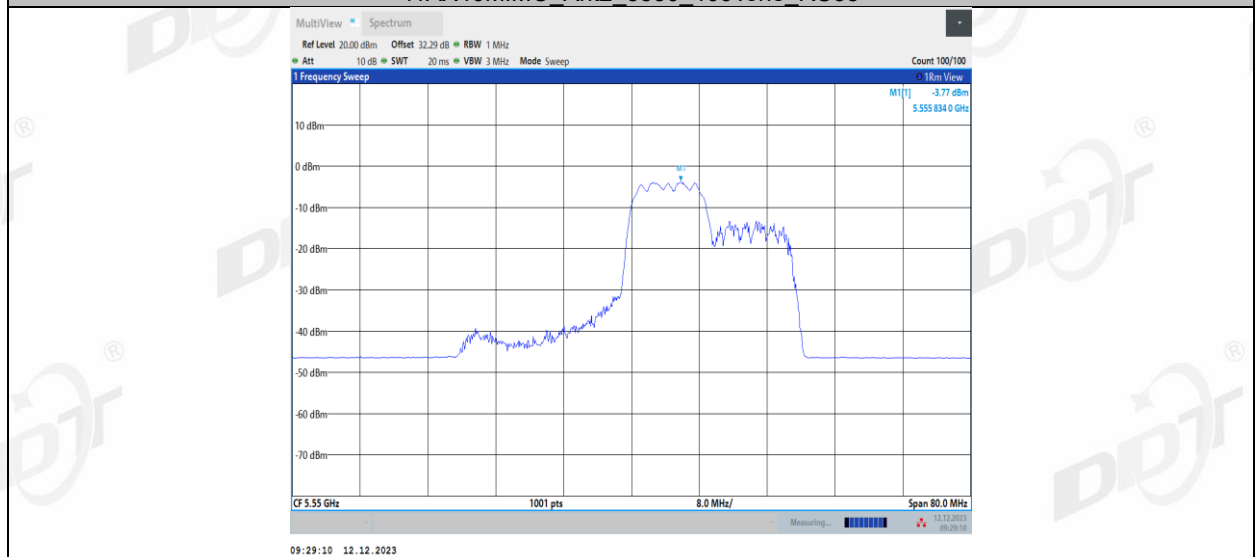
11AX40MIMO_Ant2_5550_106Tone_RU56
