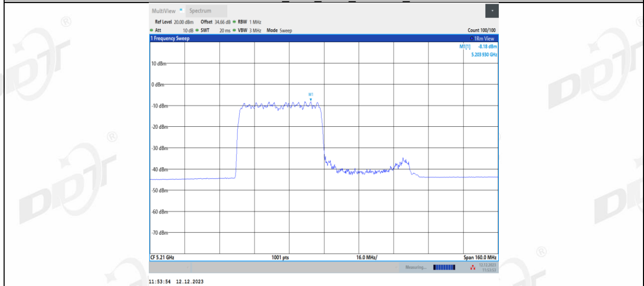
11AX80MIMO_Ant2_5210_484Tone_RU66
