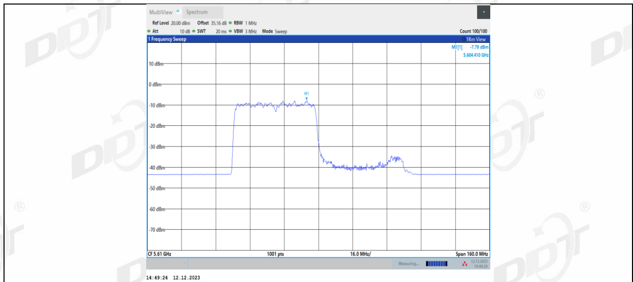
11AX80MIMO_Ant1_5610_484Tone_RU66
