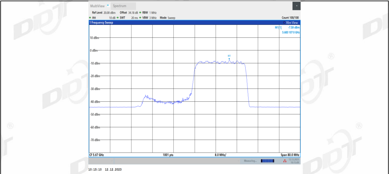
11AX40MIMO_Ant2_5670_106Tone_RU55
