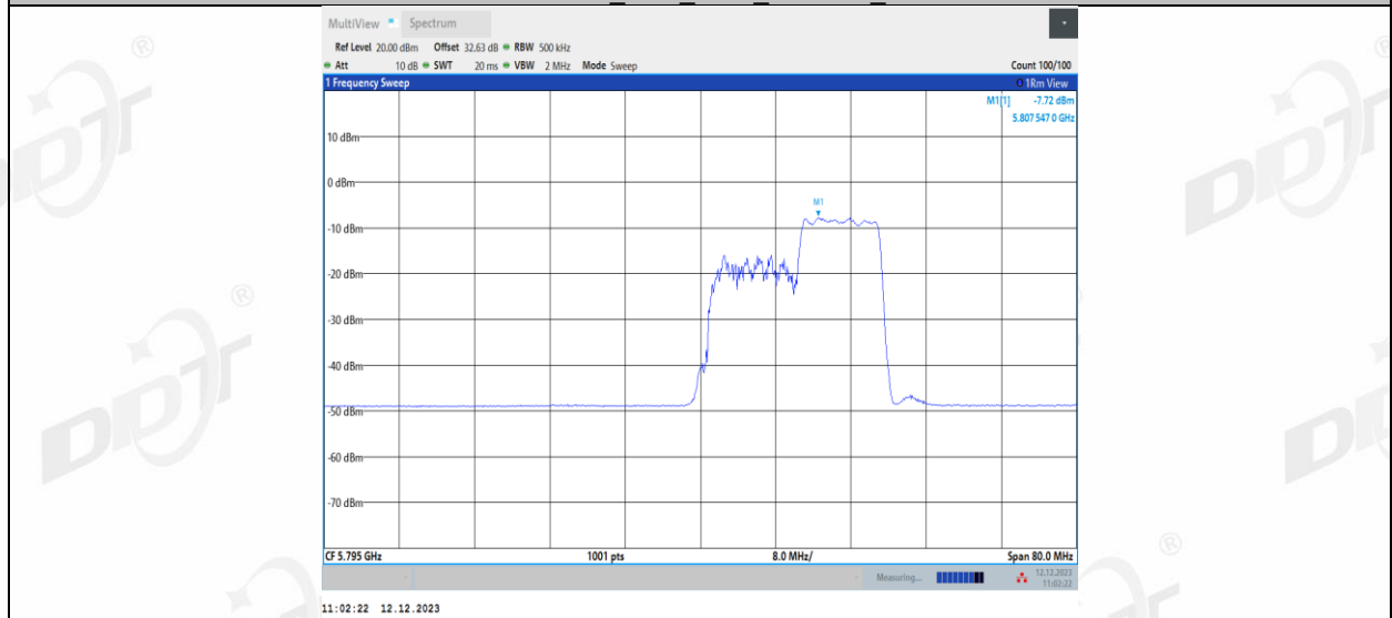
11AX40MIMO_Ant2_5795_242Tone_RU61
