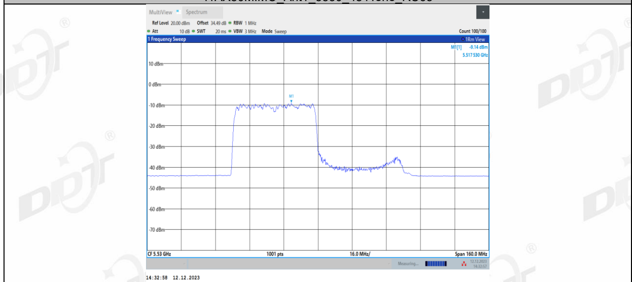
11AX80MIMO_Ant1_5530_484Tone_RU66
