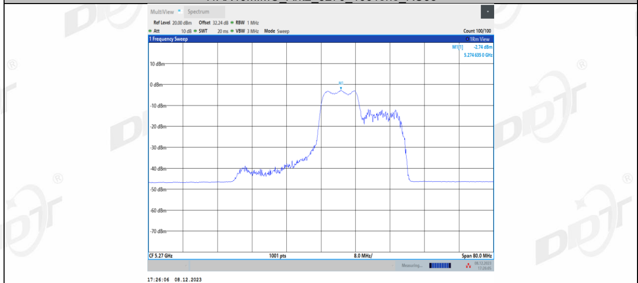
11AX40MIMO_Ant2_5270_106Tone_RU56
