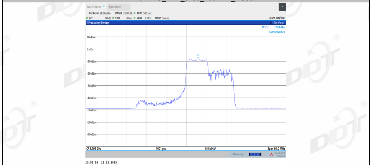
11AX40MIMO_Ant1_5795_106Tone_RU56
