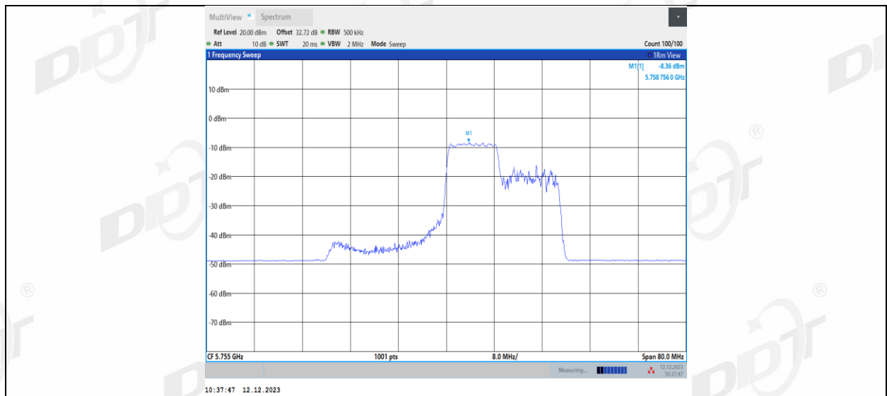
11AX40MIMO_Ant1_5755_106Tone_RU56
