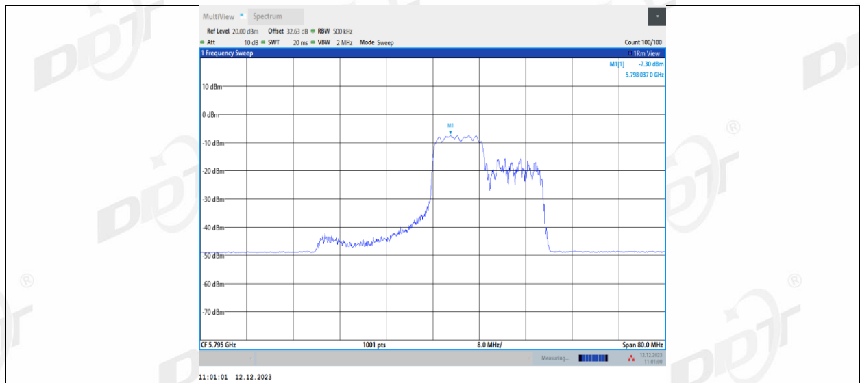
11AX40MIMO_Ant2_5795_106Tone_RU56
