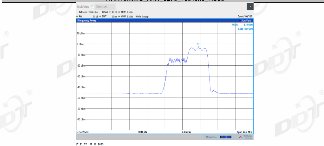
11AX40MIMO_Ant1_5270_242Tone_RU61
