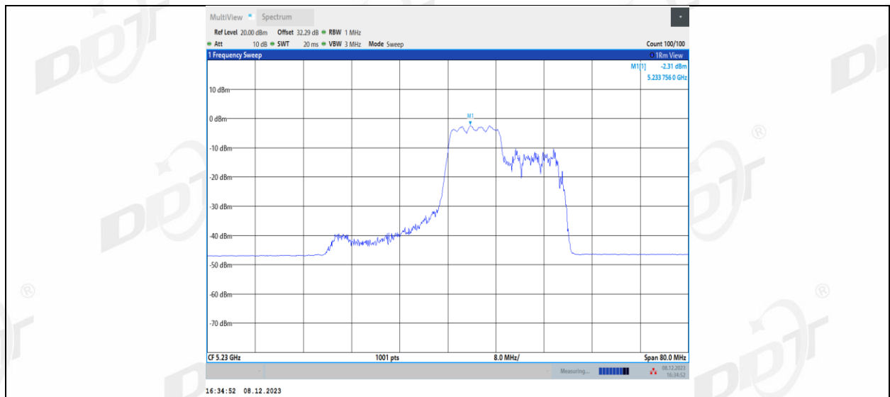
11AX40MIMO_Ant2_5230_106Tone_RU56
