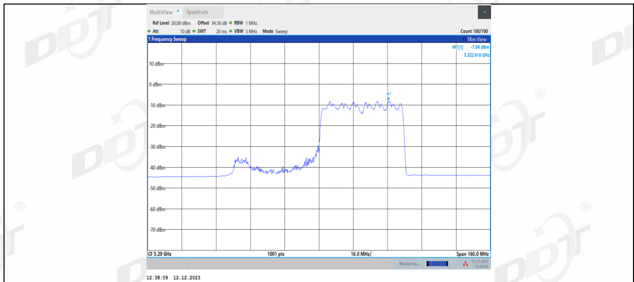
11AX80MIMO_Ant2_5290_242Tone_RU63
