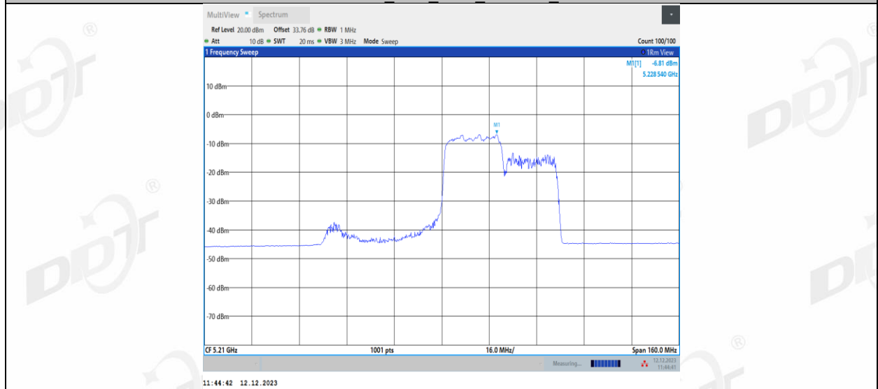
11AX80MIMO_Ant1_5210_242Tone_RU64
