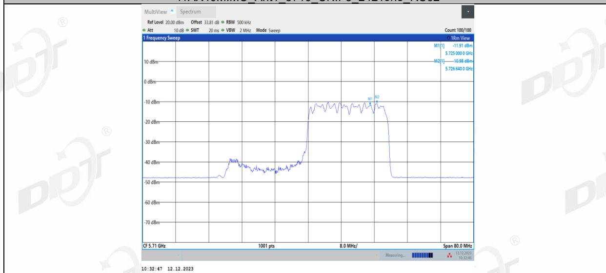
11AX40MIMO_Ant2_5710_UNII-3_106Tone_RU55
