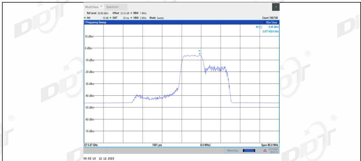
11AX40MIMO_Ant1_5670_106Tone_RU56
