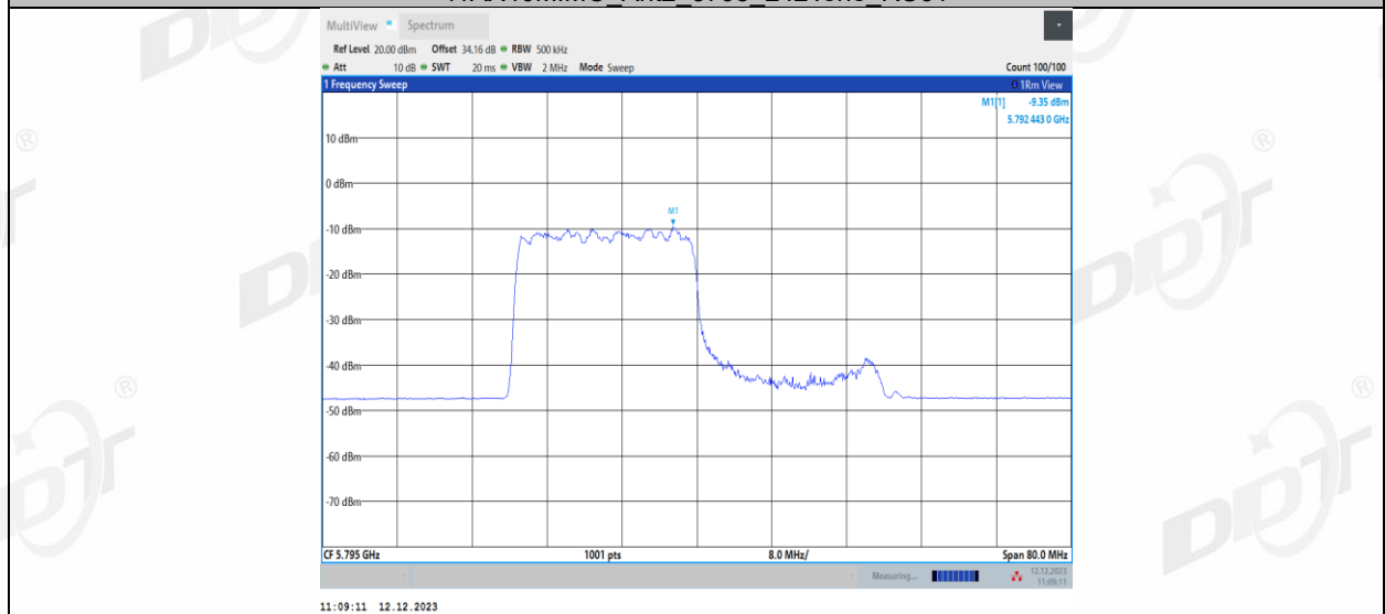
11AX40MIMO_Ant2_5795_242Tone_RU62
