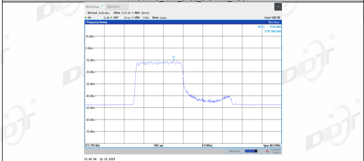
11AX40MIMO_Ant1_5755_242Tone_RU62
