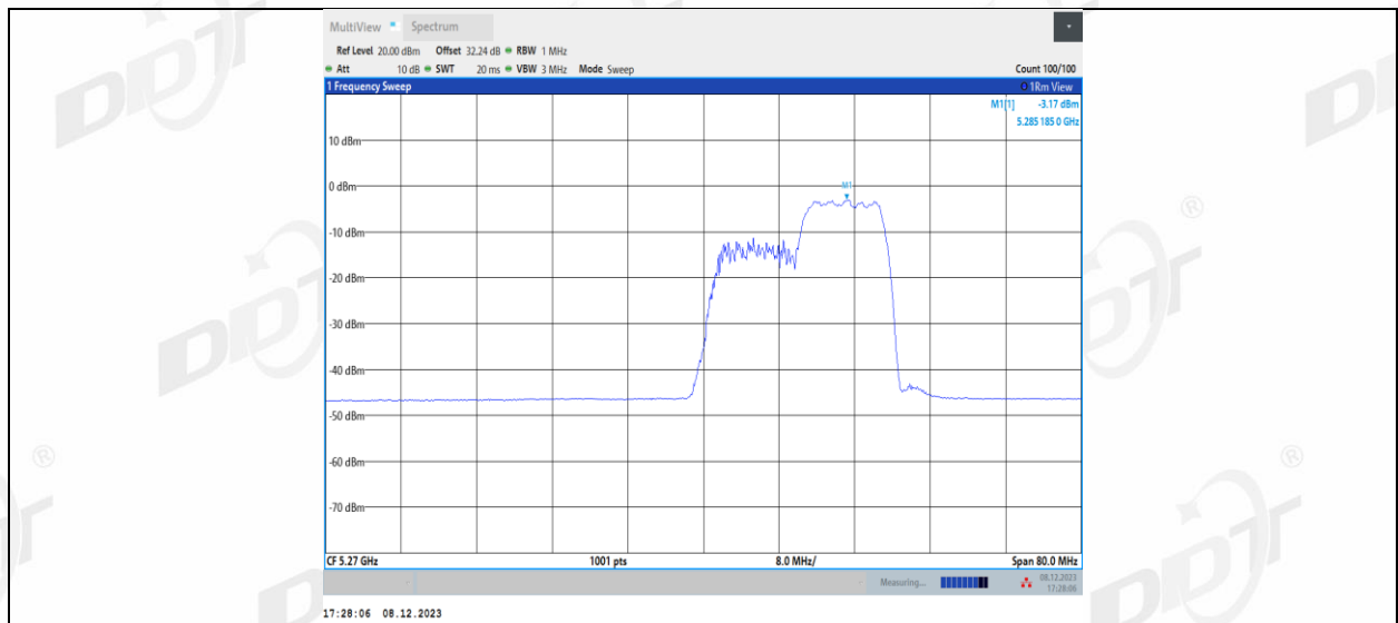
11AX40MIMO_Ant2_5270_242Tone_RU61
