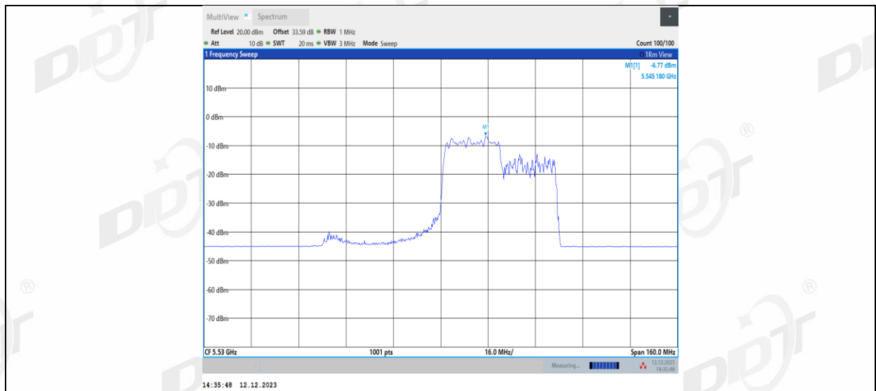
11AX80MIMO_Ant2_5530_242Tone_RU64
