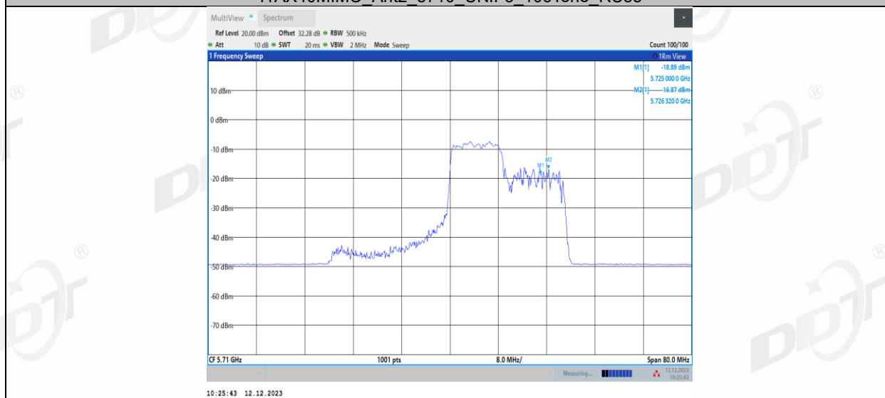
11AX40MIMO_Ant2_5710_UNII-3_106Tone_RU56
