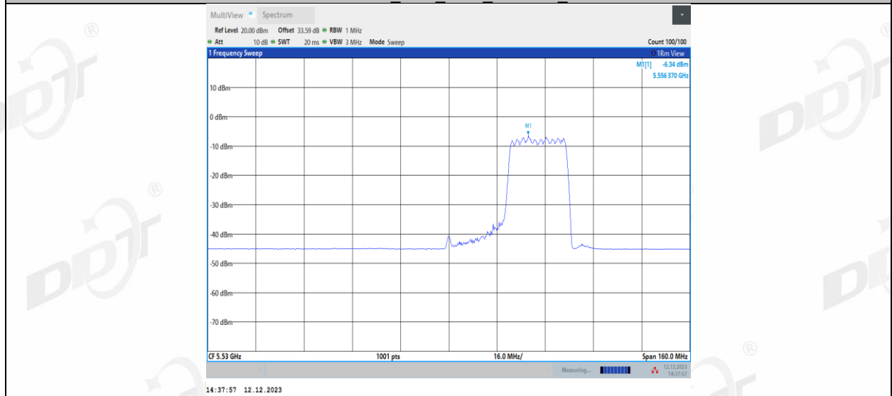
11AX80MIMO_Ant2_5530_484Tone_RU65
