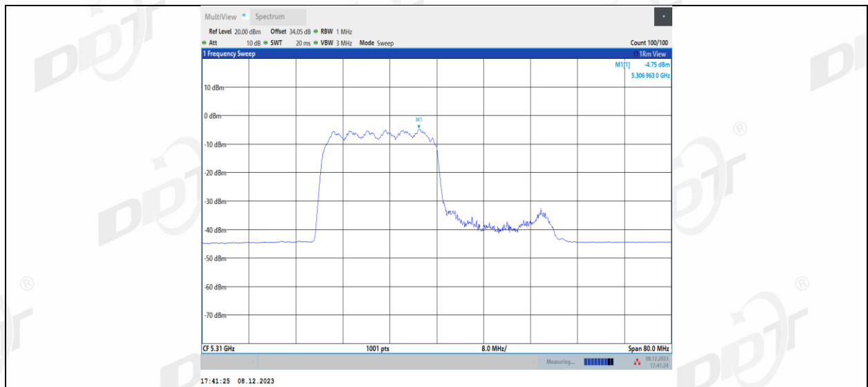
11AX40MIMO_Ant2_5310_242Tone_RU62
