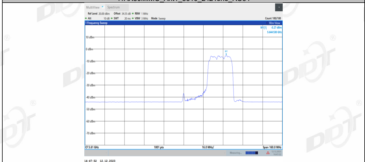
11AX80MIMO_Ant1_5610_484Tone_RU65
