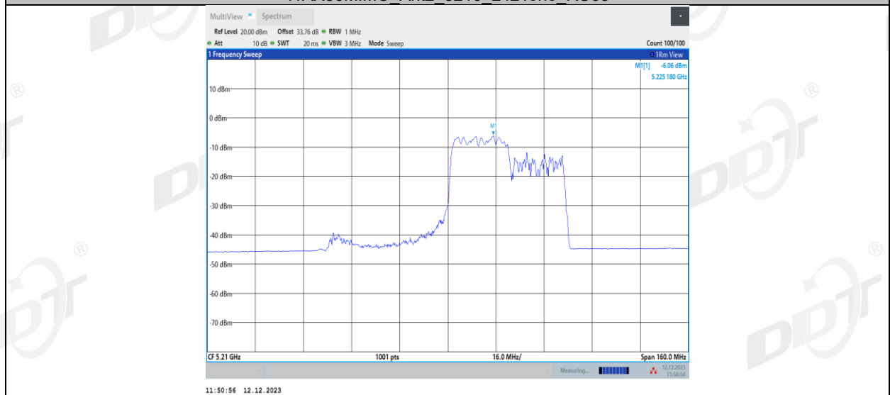
11AX80MIMO_Ant2_5210_242Tone_RU64
