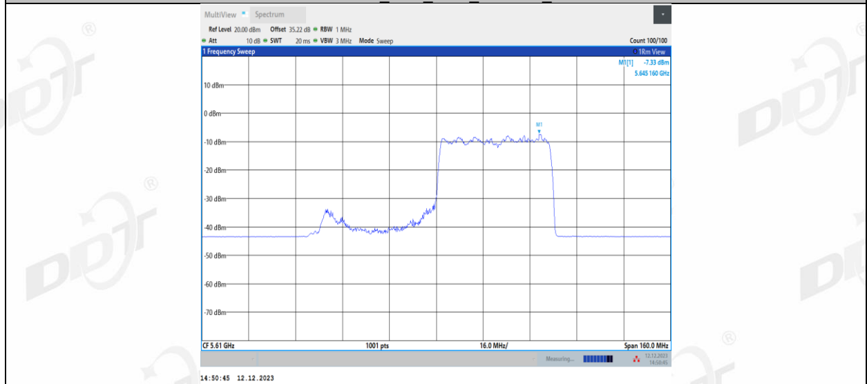
11AX80MIMO_Ant2_5610_242Tone_RU63
