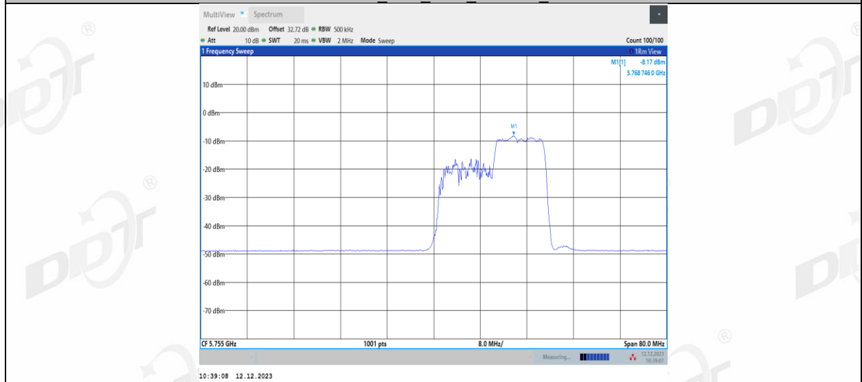
11AX40MIMO_Ant1_5755_242Tone_RU61
