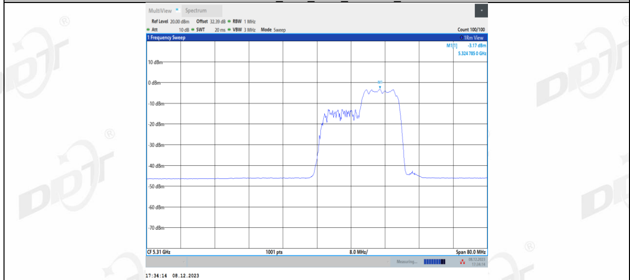
11AX40MIMO_Ant1_5310_242Tone_RU61
