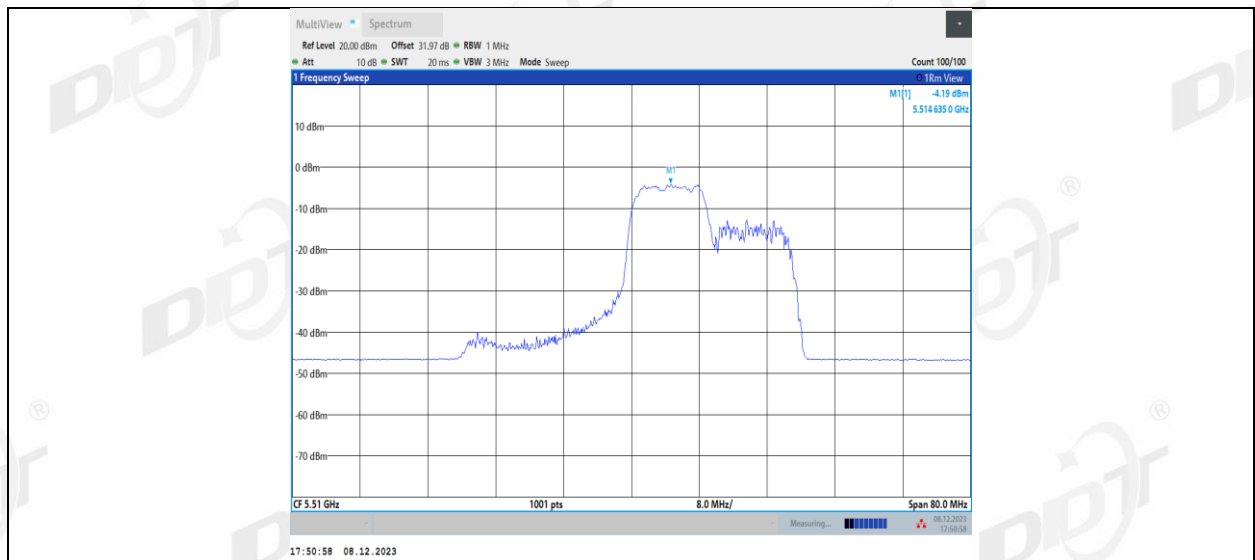
11AX40MIMO_Ant2_5510_106Tone_RU56
