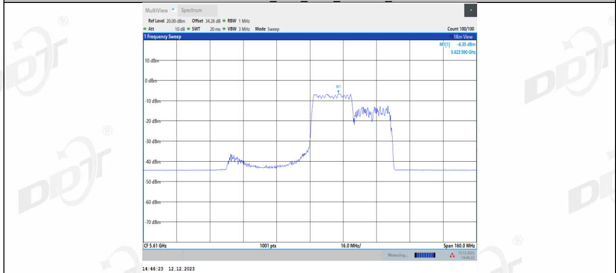
11AX80MIMO_Ant1_5610_242Tone_RU64
