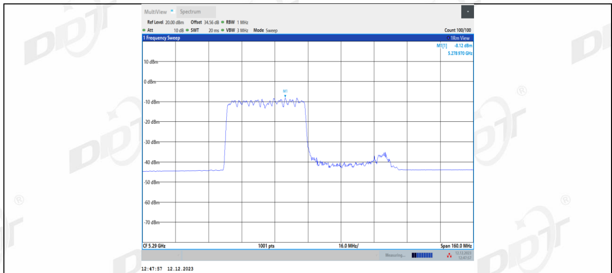
11AX80MIMO_Ant2_5290_484Tone_RU66
