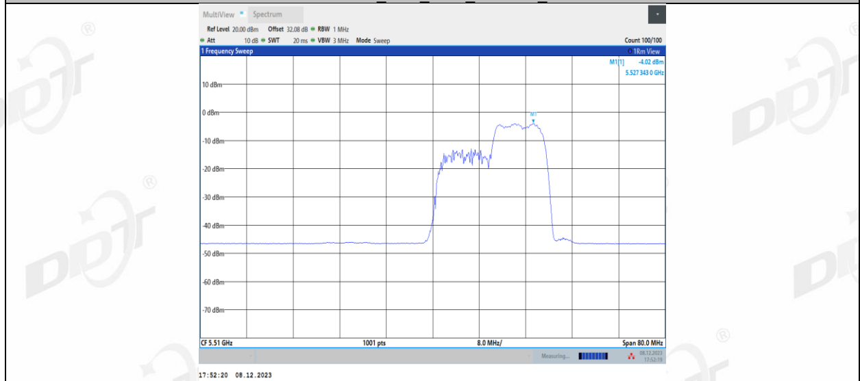
11AX40MIMO_Ant2_5510_242Tone_RU61
