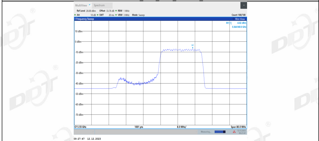
11AX40MIMO_Ant2_5550_106Tone_RU55
