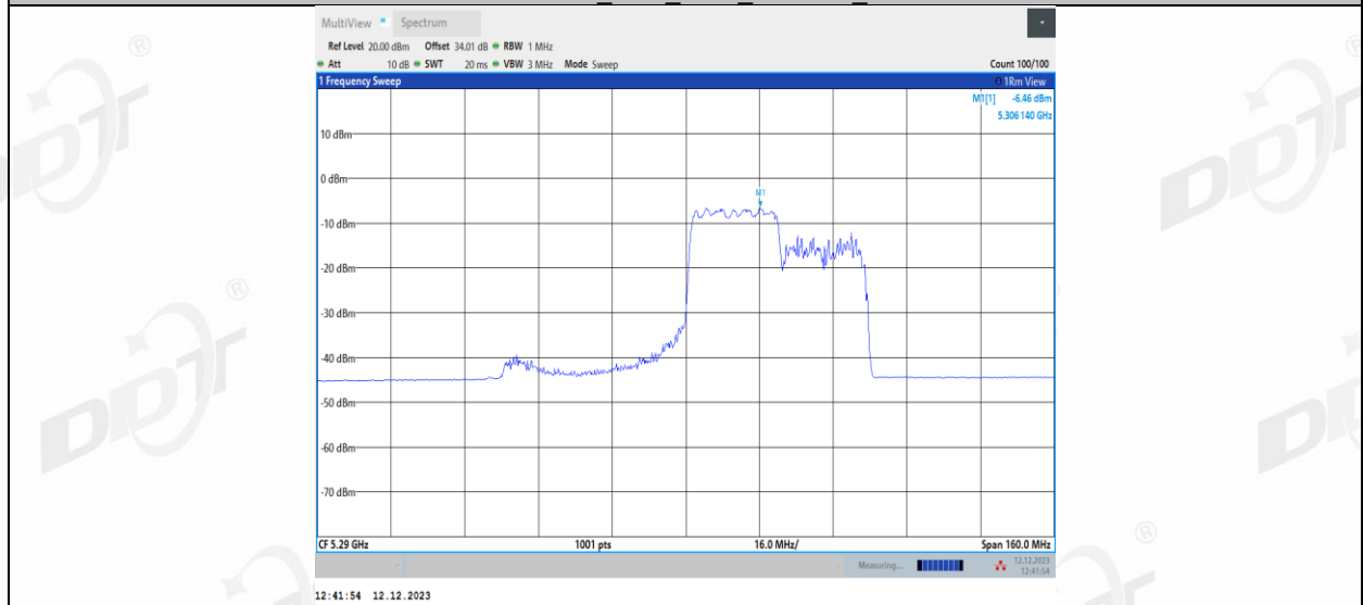
11AX80MIMO_Ant2_5290_242Tone_RU64
