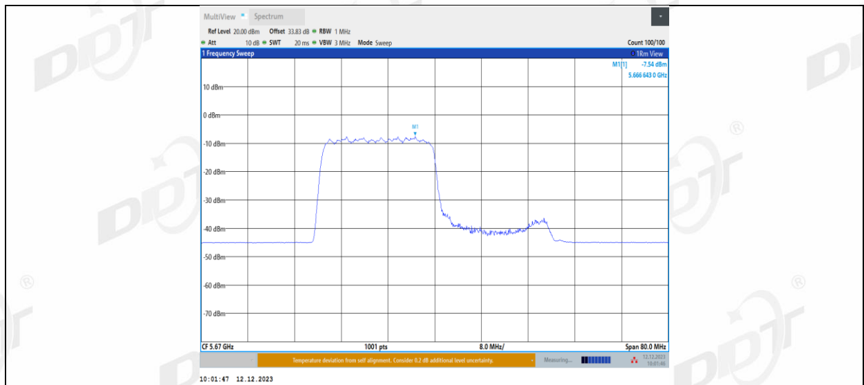
11AX40MIMO_Ant2_5670_242Tone_RU62
