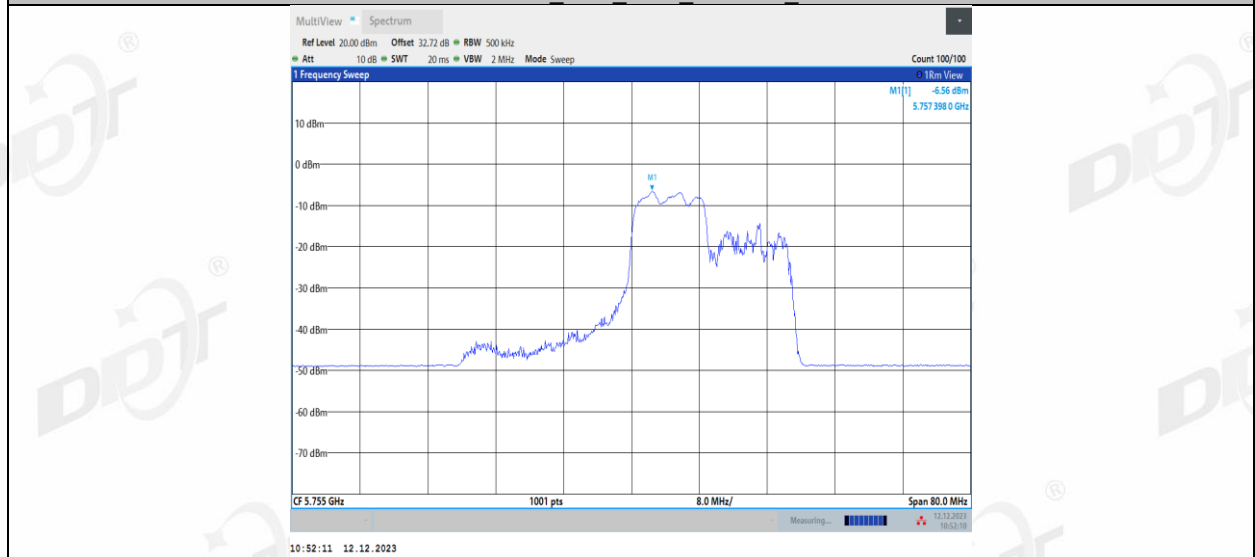
11AX40MIMO_Ant2_5755_106Tone_RU56
