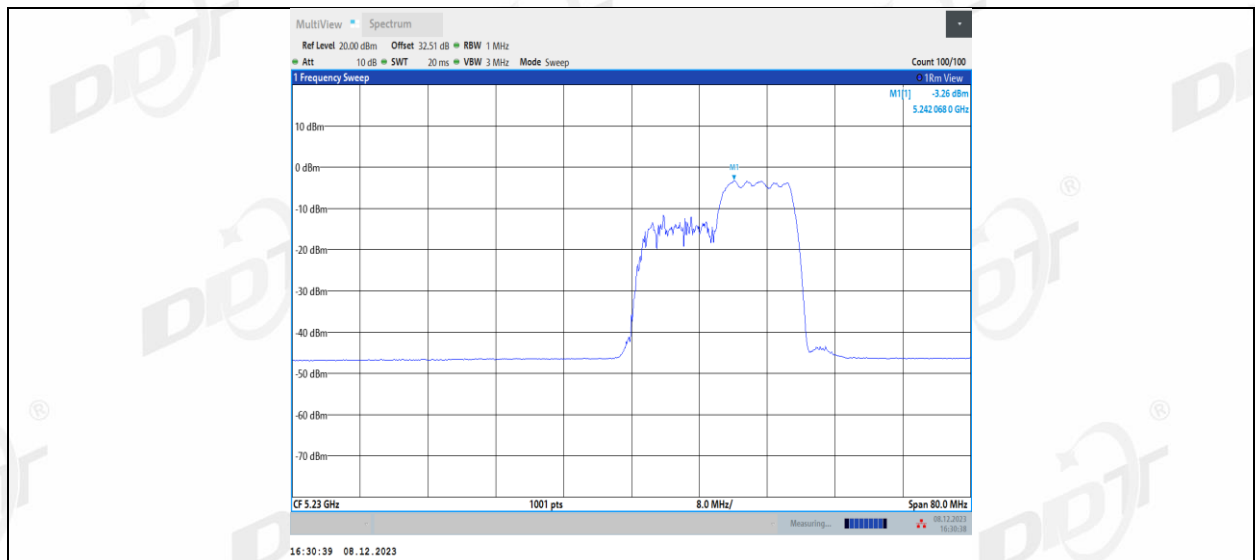
11AX40MIMO_Ant1_5230_242Tone_RU61
