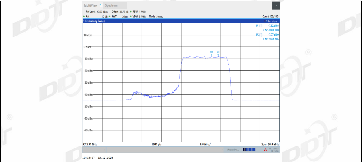
11AX40MIMO_Ant1_5710_UNII-3_106Tone_RU55
