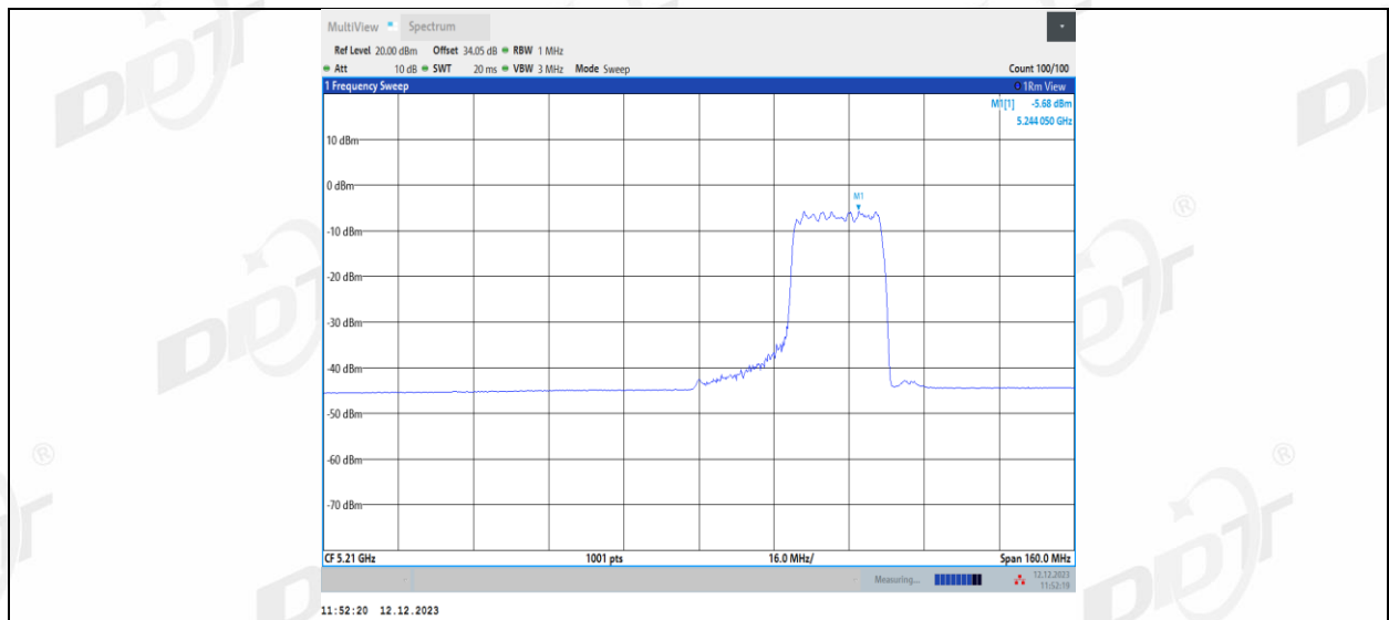
11AX80MIMO_Ant2_5210_484Tone_RU65
