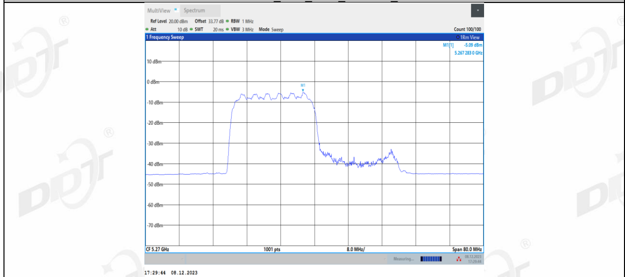
11AX40MIMO_Ant2_5270_242Tone_RU62
