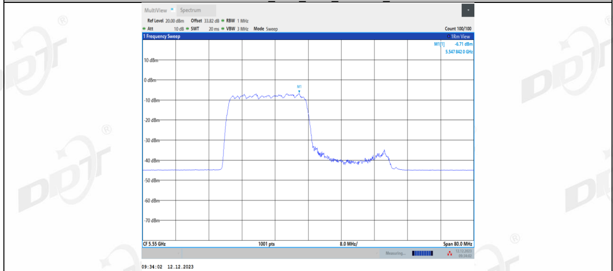
11AX40MIMO_Ant2_5550_242Tone_RU62
