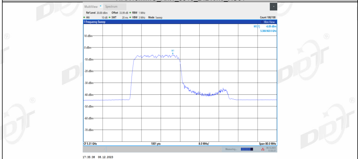
11AX40MIMO_Ant1_5310_242Tone_RU62
