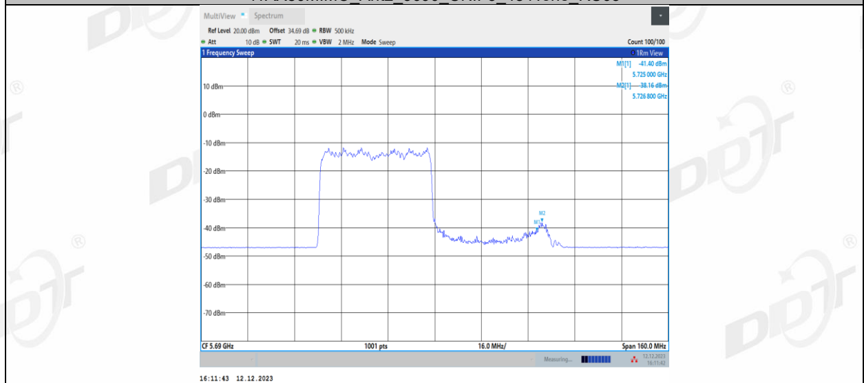
11AX80MIMO_Ant2_5690_UNII-3_484Tone_RU66
