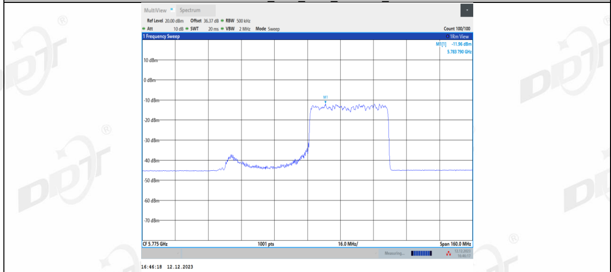
11AX80MIMO_Ant2_5775_242Tone_RU63
