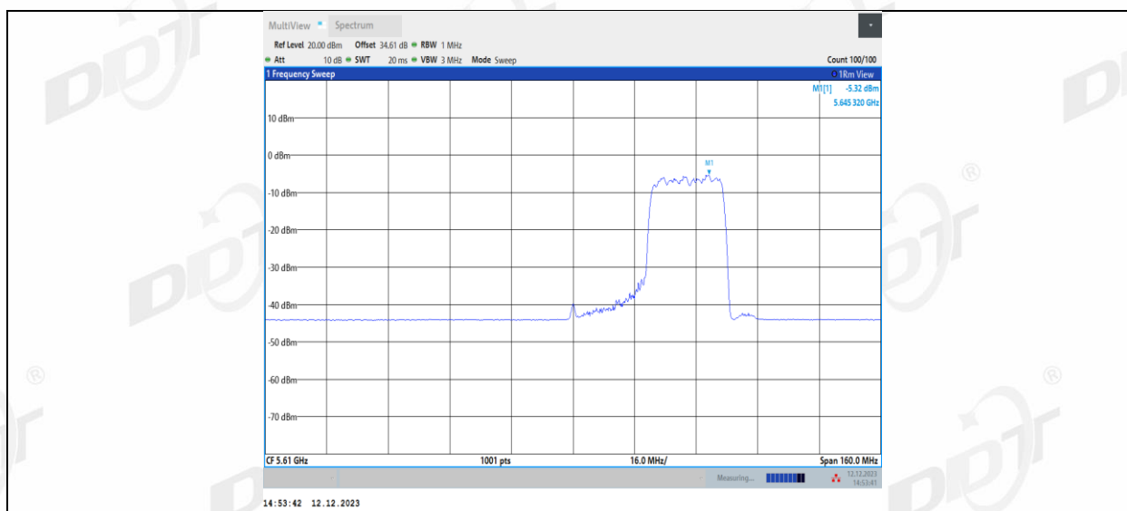
11AX80MIMO_Ant2_5610_484Tone_RU65
