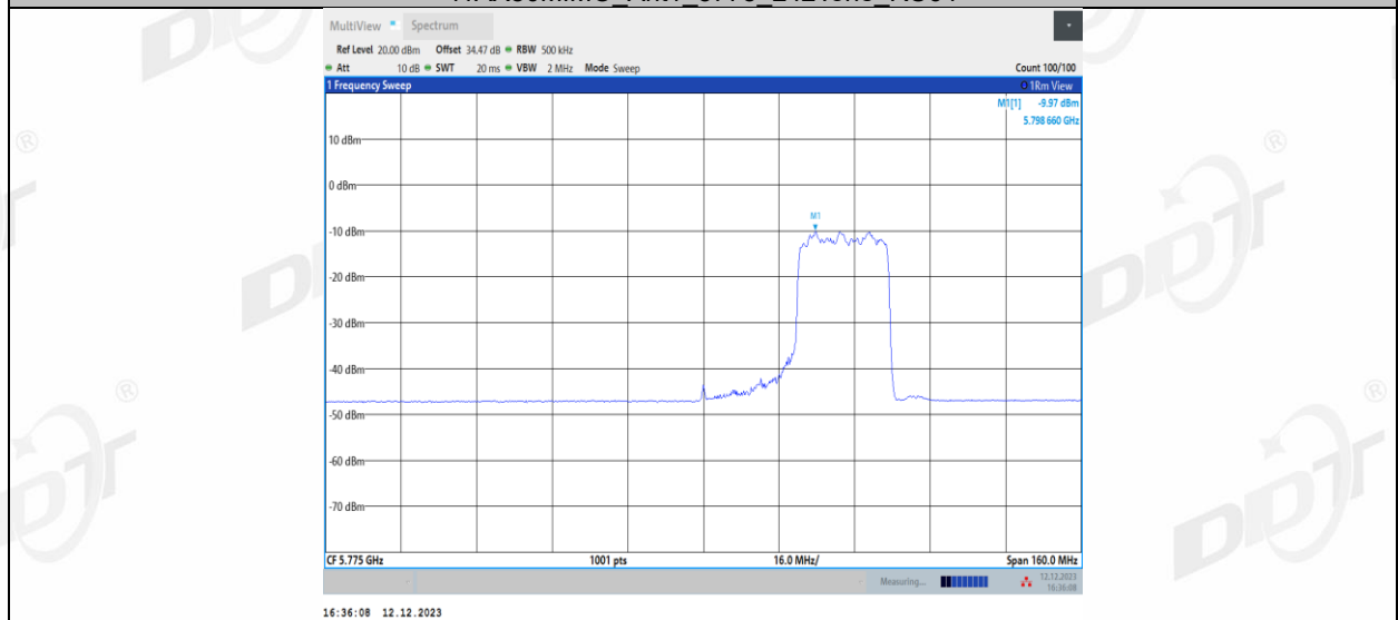
11AX80MIMO_Ant1_5775_484Tone_RU65
