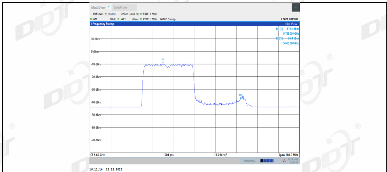
11AX80MIMO_Ant2_5690_UNII-2C_484Tone_RU66
