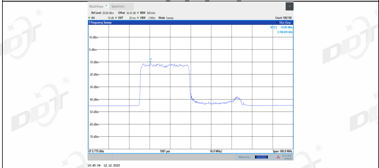
11AX80MIMO_Ant2_5775_484Tone_RU66
