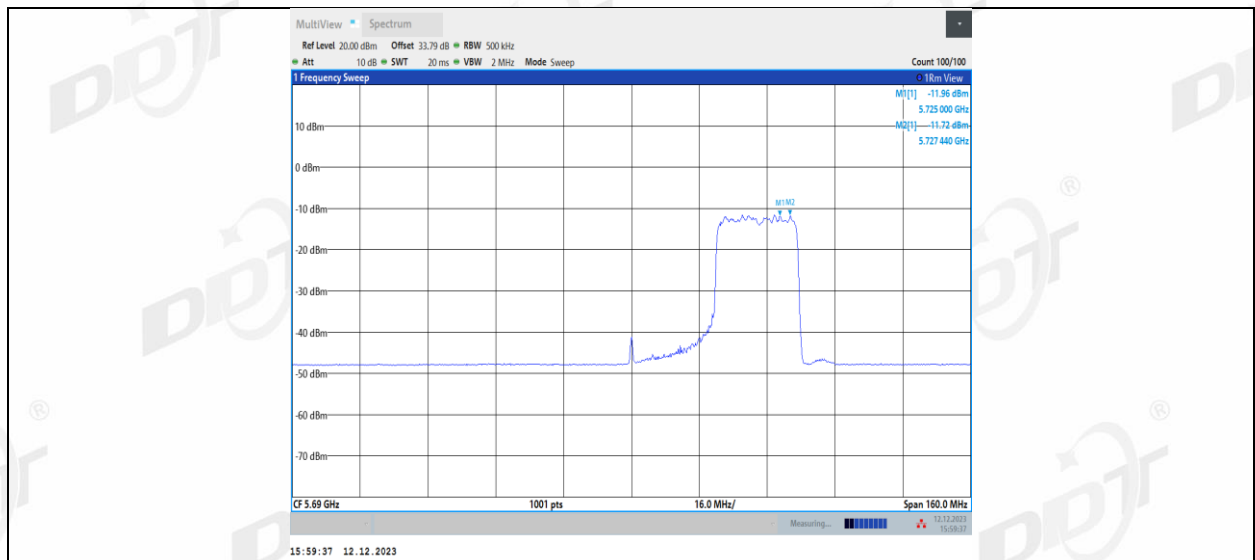
11AX80MIMO_Ant1_5690_UNII-3_484Tone_RU65
