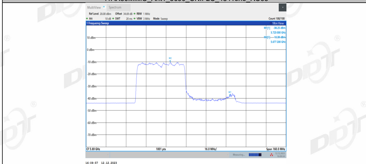
11AX80MIMO_Ant1_5690_UNII-2C_484Tone_RU66
