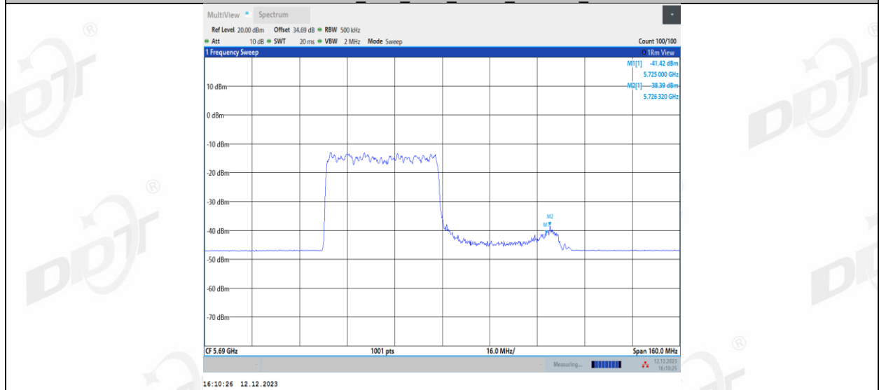
11AX80MIMO_Ant1_5690_UNII-3_484Tone_RU66
