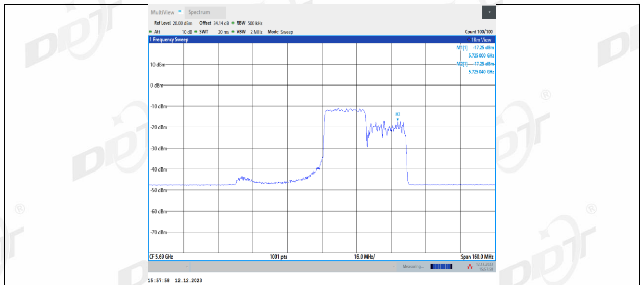
11AX80MIMO_Ant2_5690_UNII-3_242Tone_RU64
