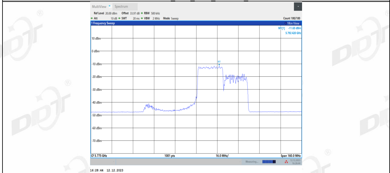
11AX80MIMO_Ant1_5775_242Tone_RU64
