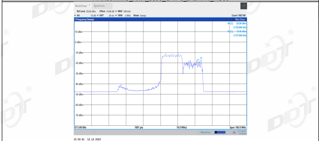
11AX80MIMO_Ant1_5690_UNII-3_242Tone_RU64
