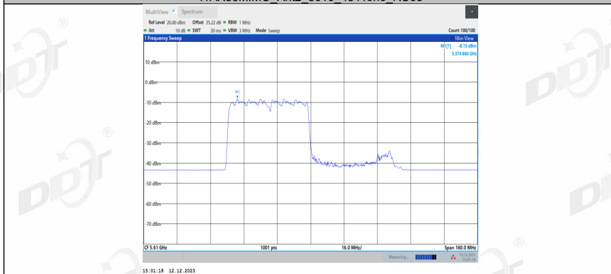
11AX80MIMO_Ant2_5610_484Tone_RU66
