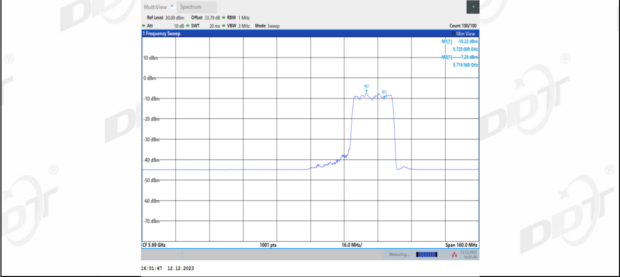
11AX80MIMO_Ant2_5690_UNII-2C_484Tone_RU65
