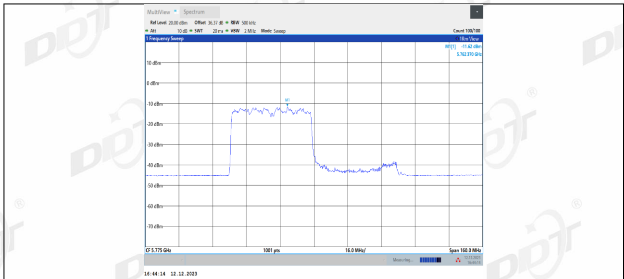
11AX80MIMO_Ant1_5775_484Tone_RU66
