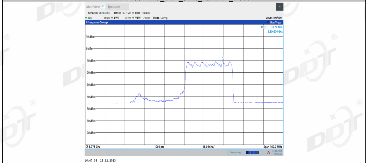
11AX80MIMO_Ant2_5775_484Tone_RU66
