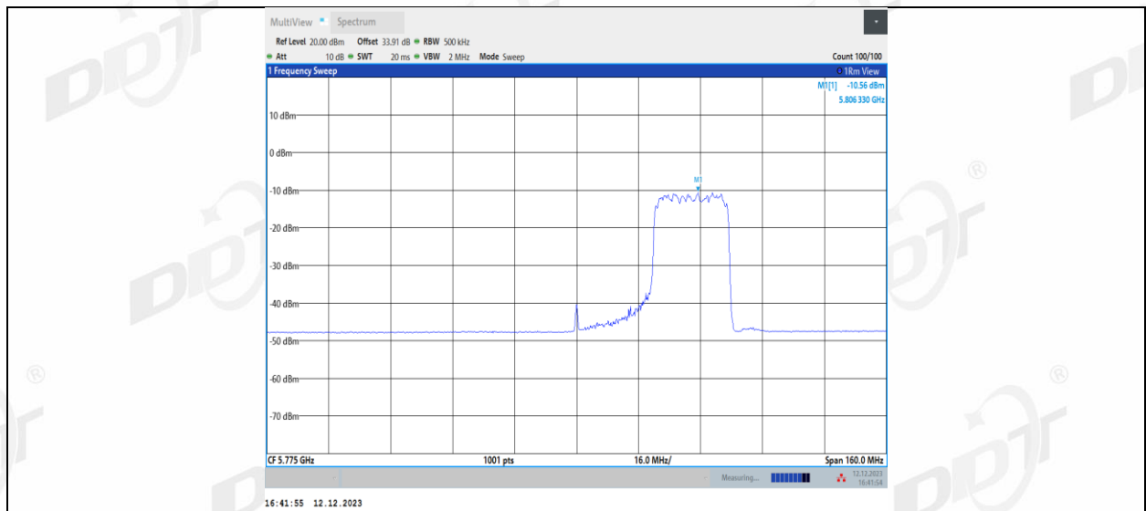
11AX80MIMO_Ant2_5775_484Tone_RU65
