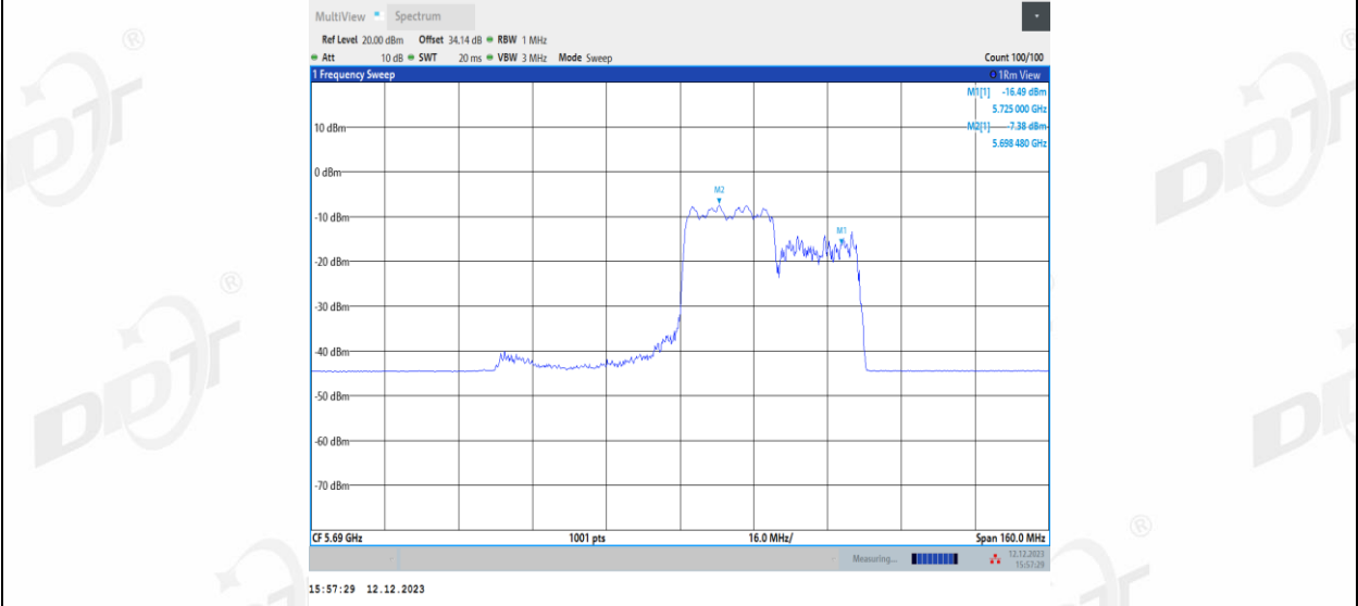
11AX80MIMO_Ant2_5690_UNII-2C_242Tone_RU64
