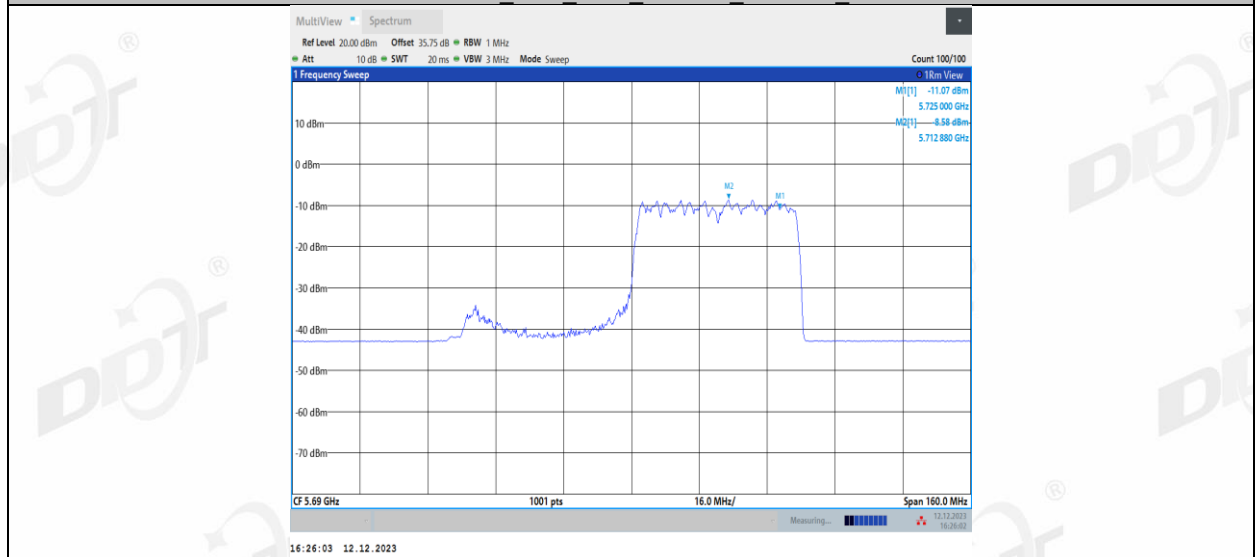
11AX80MIMO_Ant1_5690_UNII-3_242Tone_RU63
