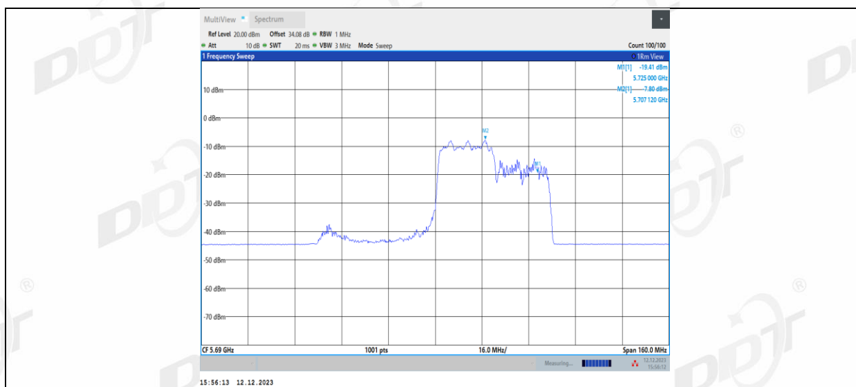
11AX80MIMO_Ant1_5690_UNII-2C_242Tone_RU64
