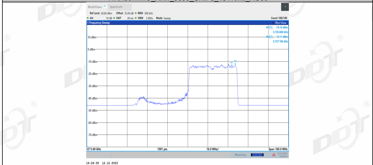
11AX80MIMO_Ant2_5690_UNII-3_242Tone_RU63
