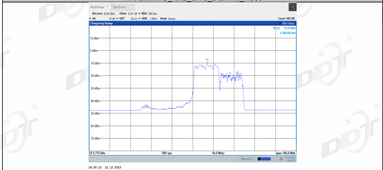
11AX80MIMO_Ant2_5775_242Tone_RU64
