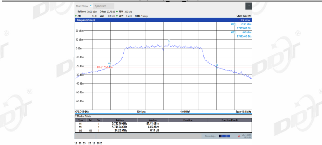
11AC20MIMO_Ant2_5745
