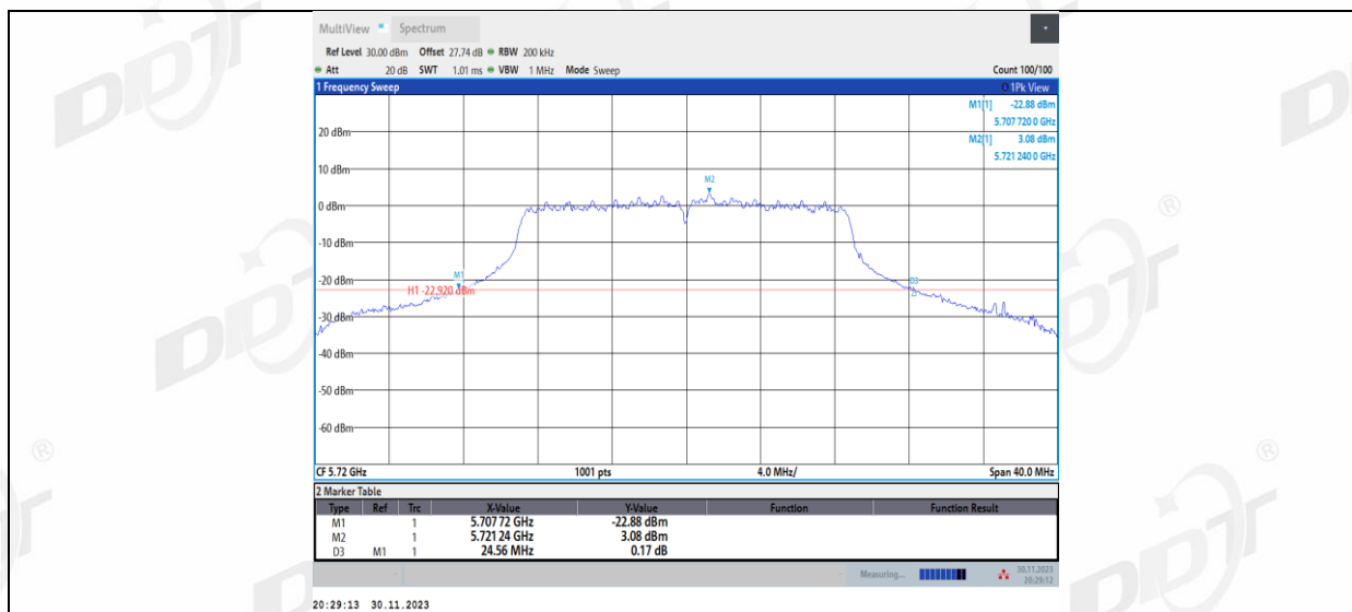
11AC20MIMO_Ant2_5720
