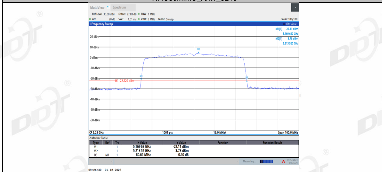
11AC80MIMO_Ant2_5210
