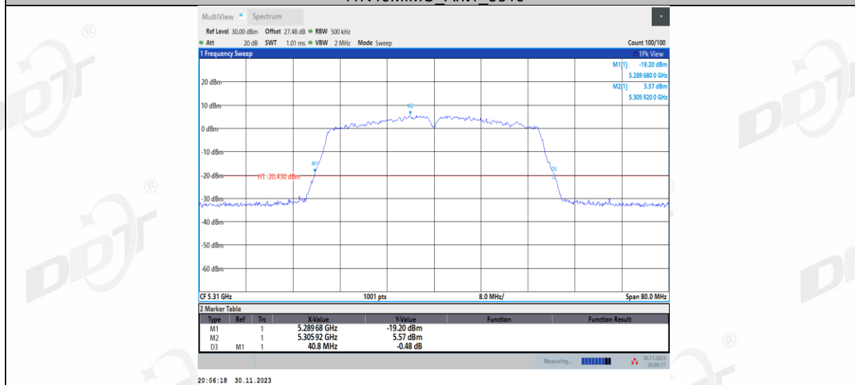
11N40MIMO_Ant2_5310
