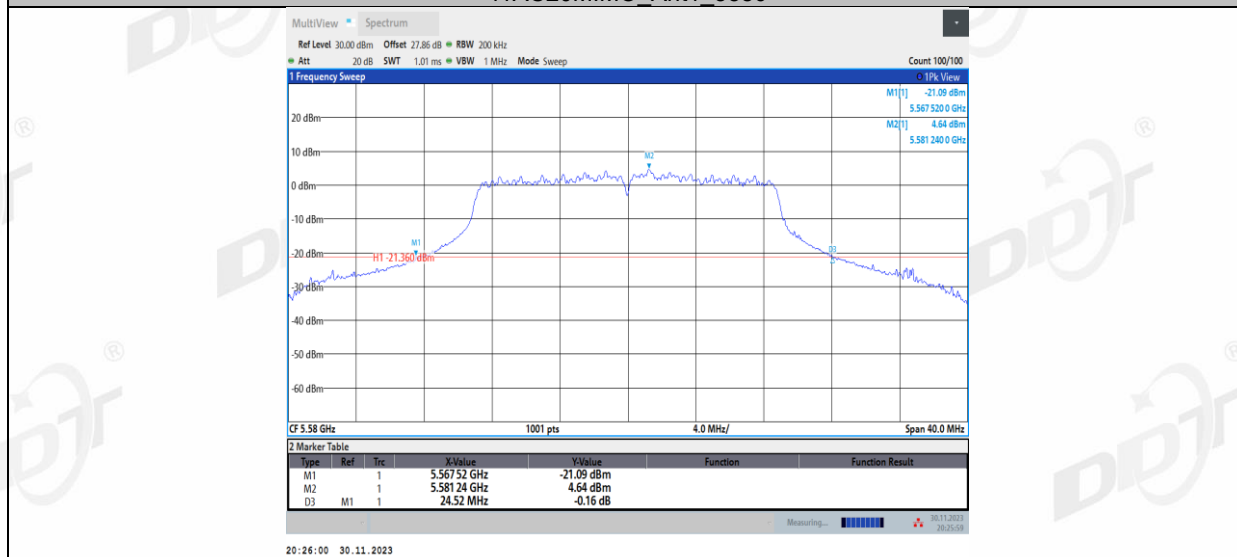
11AC20MIMO_Ant2_5580
