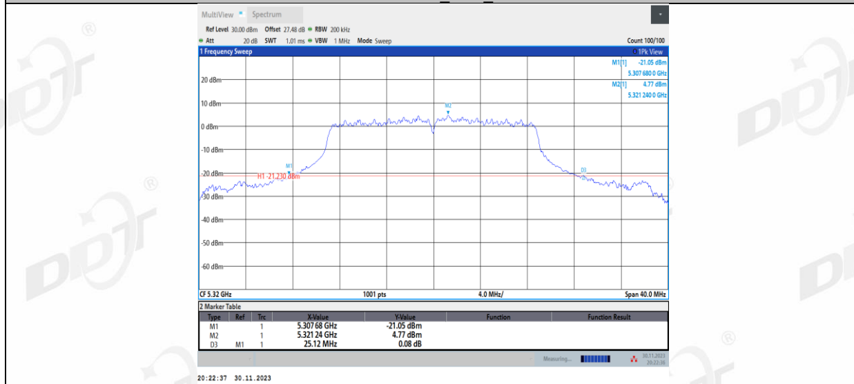
11AC20MIMO_Ant2_5320
