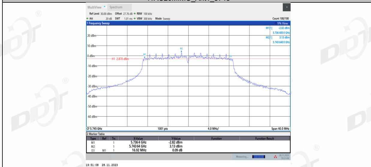
11AC20MIMO_Ant2_5745
