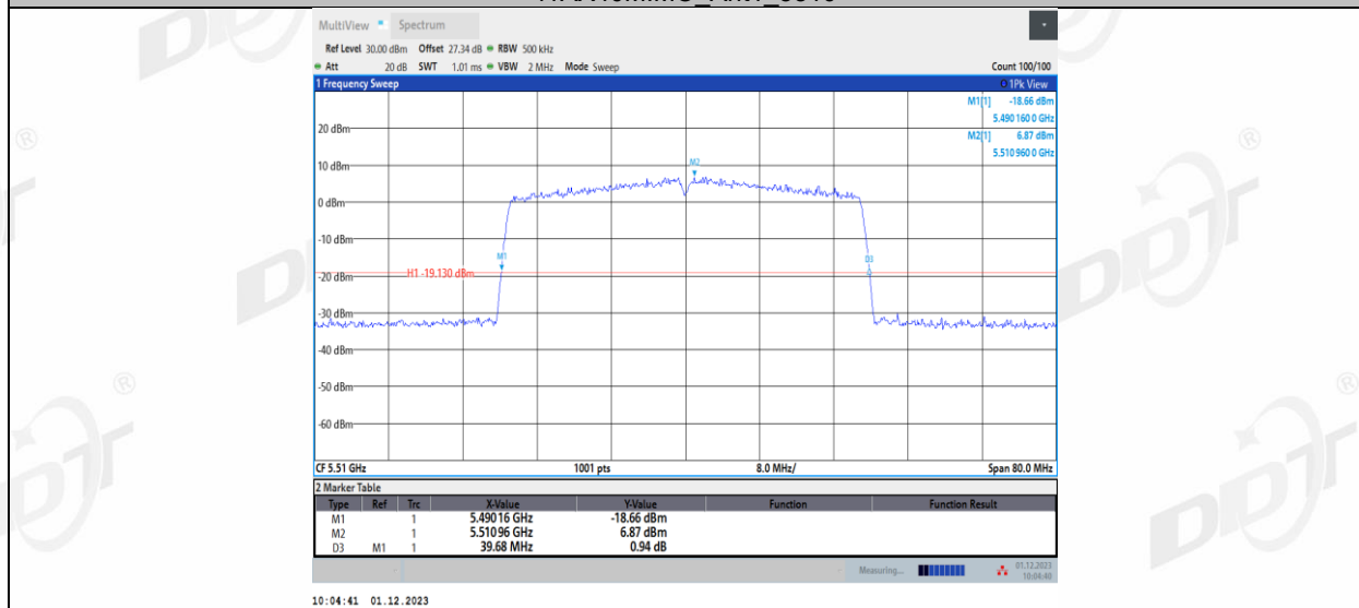
11AX40MIMO_Ant2_5510
