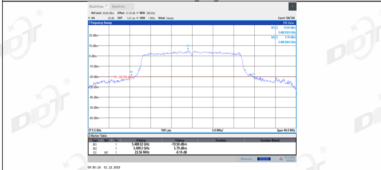
11AX20MIMO_Ant2_5500
