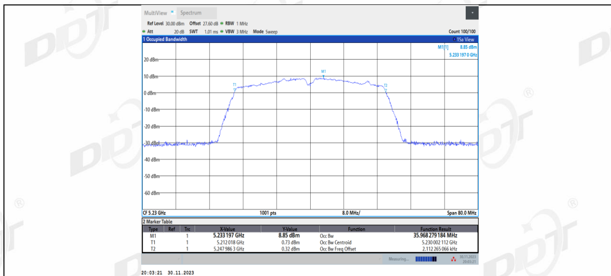
11N40MIMO_Ant2_5230
