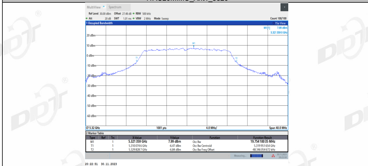
11AC20MIMO_Ant2_5320
