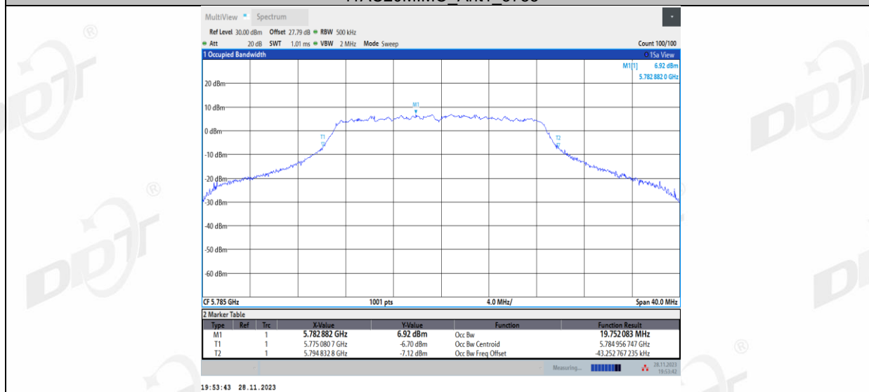
11AC20MIMO_Ant2_5785
