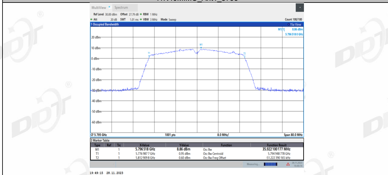
11N40MIMO_Ant2_5795
