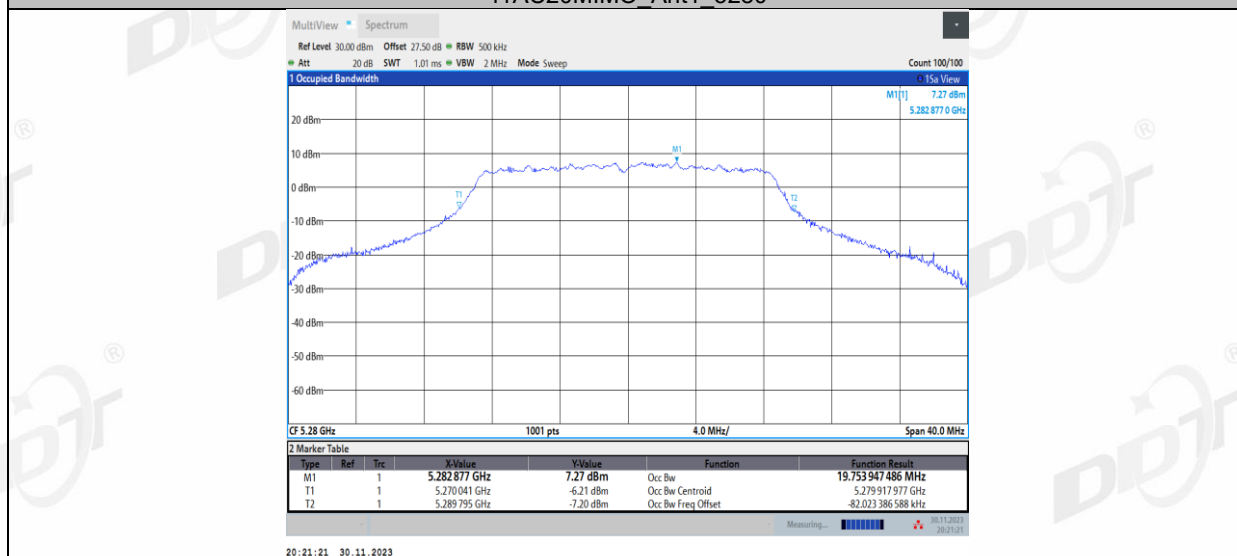
11AC20MIMO_Ant2_5280
