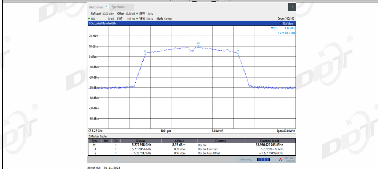
11N40MIMO_Ant2_5270
