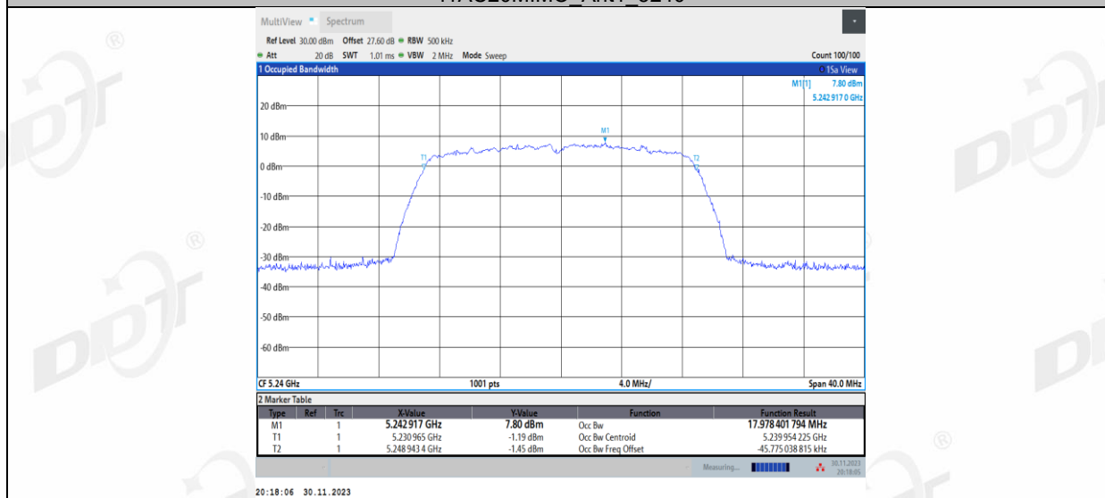
11AC20MIMO_Ant2_5240
