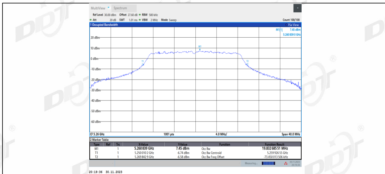
11AC20MIMO_Ant2_5260
