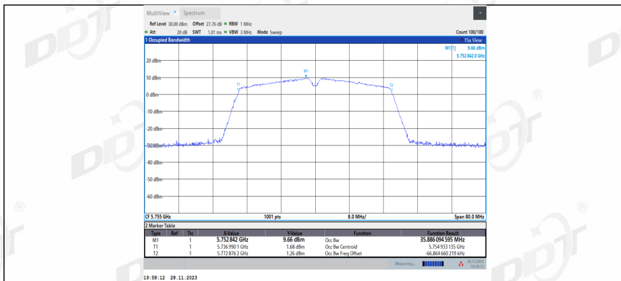
11AC40MIMO_Ant2_5755
