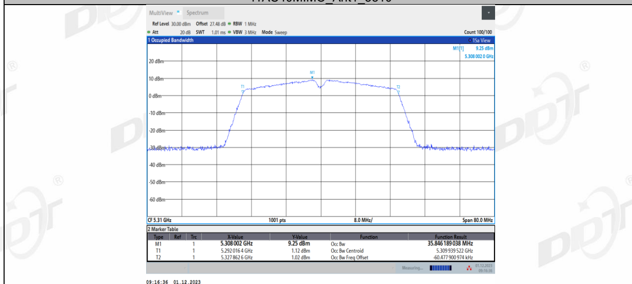
11AC40MIMO_Ant2_5310
