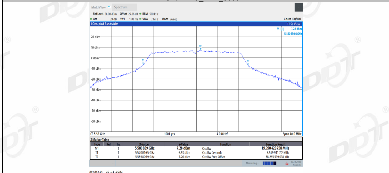
11AC20MIMO_Ant2_5580
