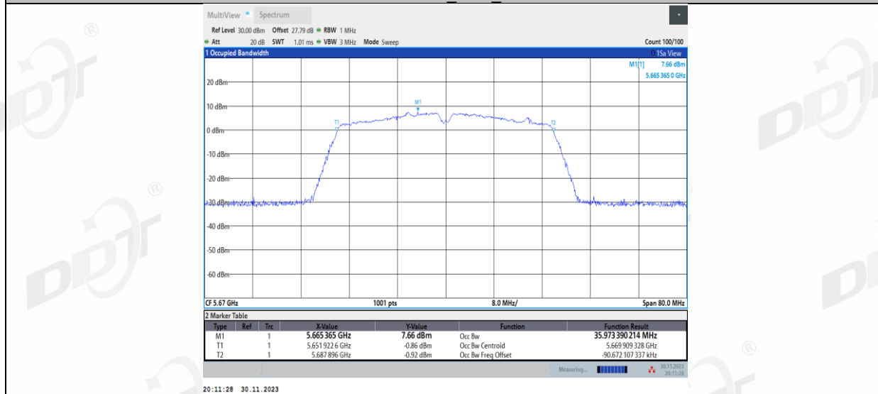
11N40MIMO_Ant2_5670
