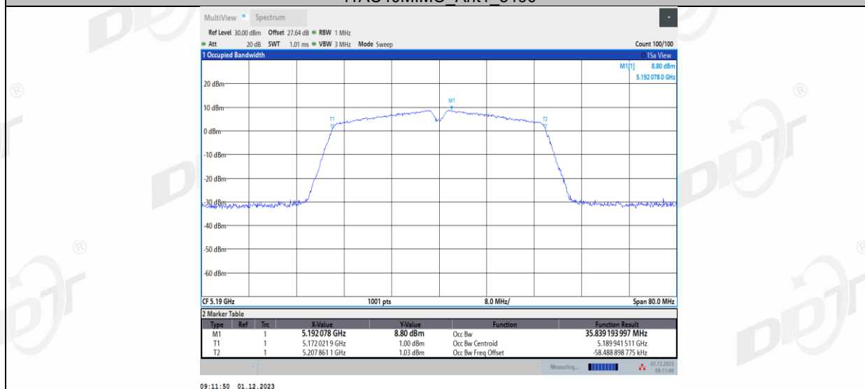
11AC40MIMO_Ant2_5190
