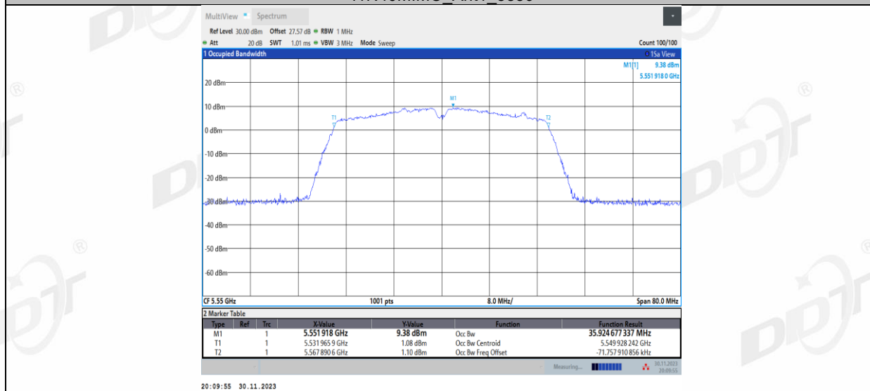
11N40MIMO_Ant2_5550
