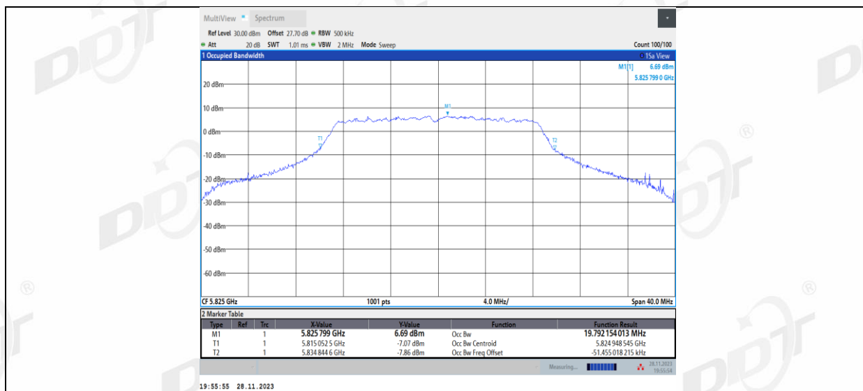
11AC20MIMO_Ant2_5825
