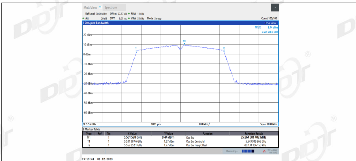
11AC40MIMO_Ant2_5550
