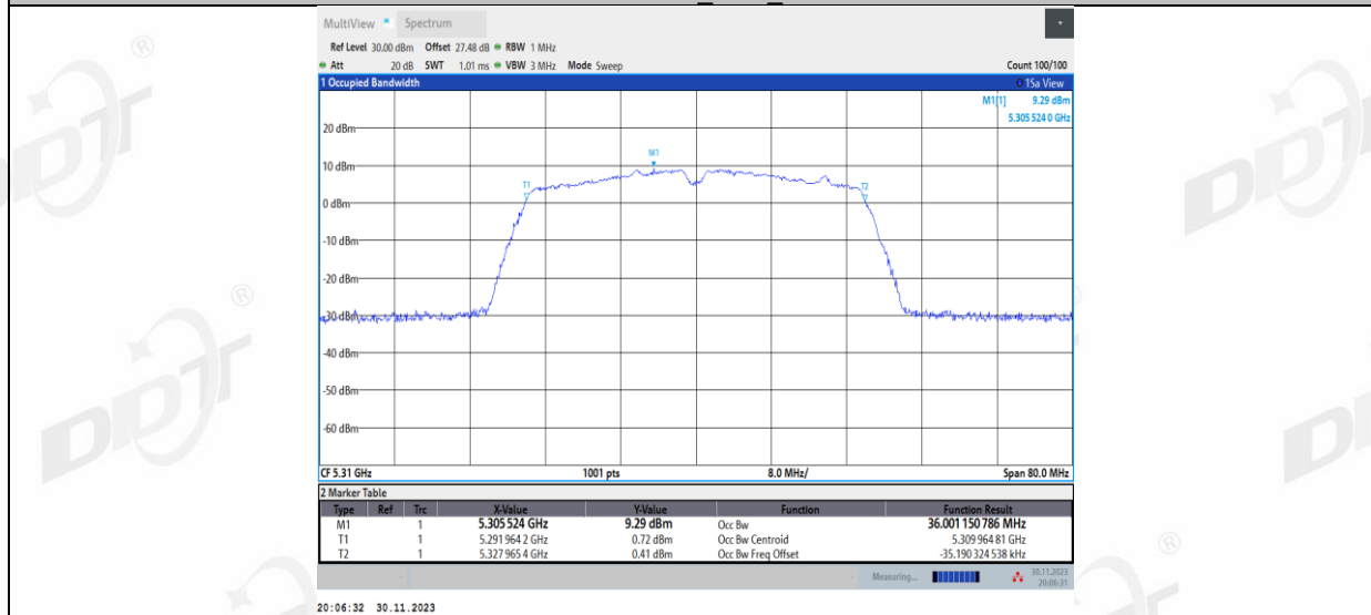
11N40MIMO_Ant2_5310
