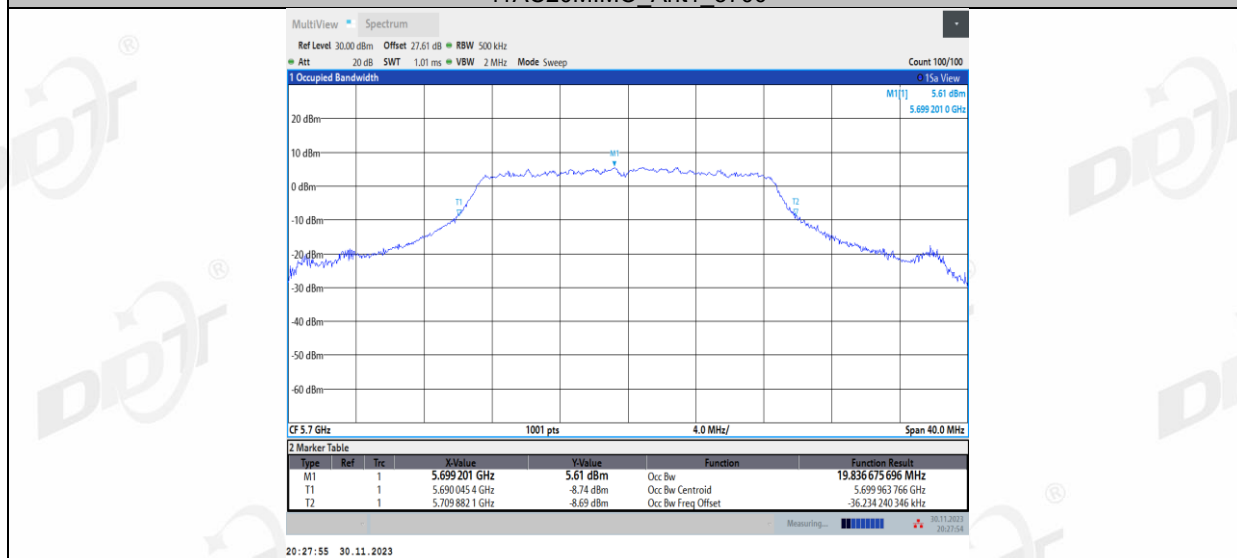
11AC20MIMO_Ant2_5700
