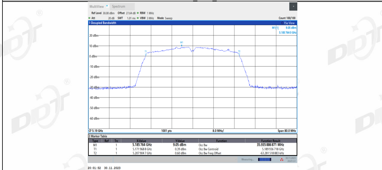
11N40MIMO_Ant2_5190
