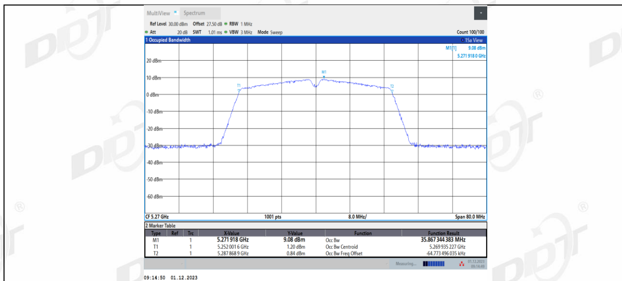
11AC40MIMO_Ant2_5270
