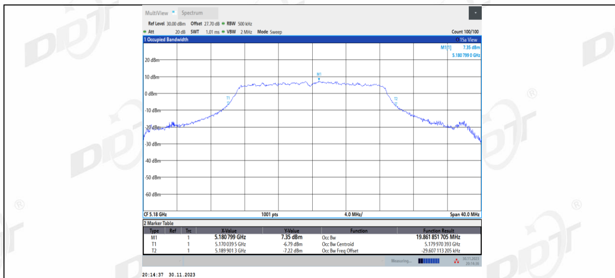
11AC20MIMO_Ant2_5180
