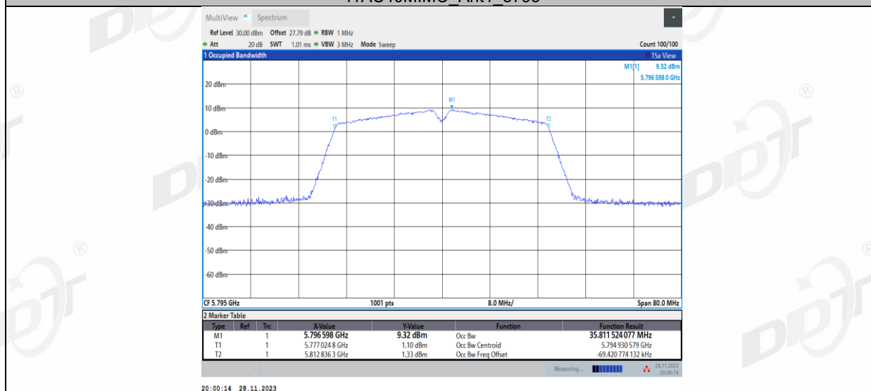
11AC40MIMO_Ant2_5795
