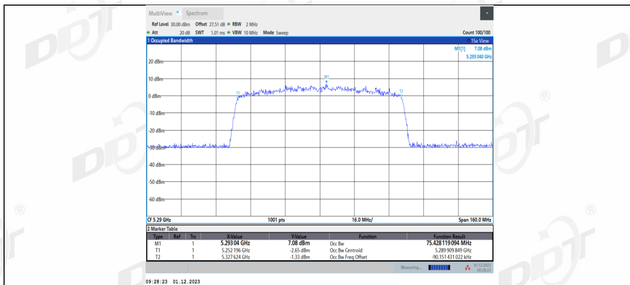
11AC80MIMO_Ant2_5290
