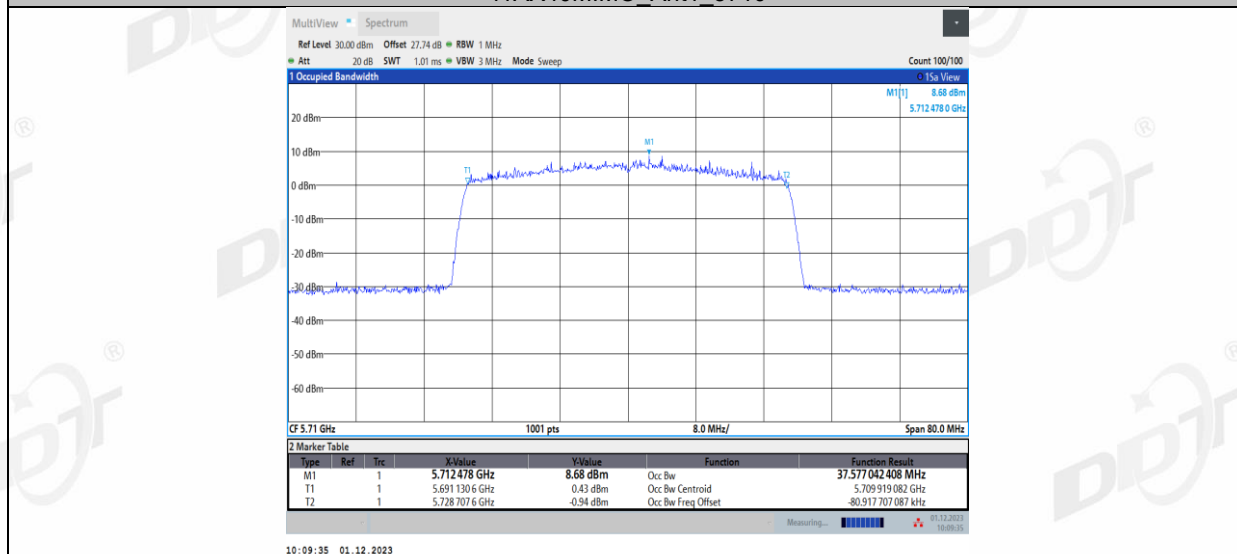
11AX40MIMO_Ant2_5710
