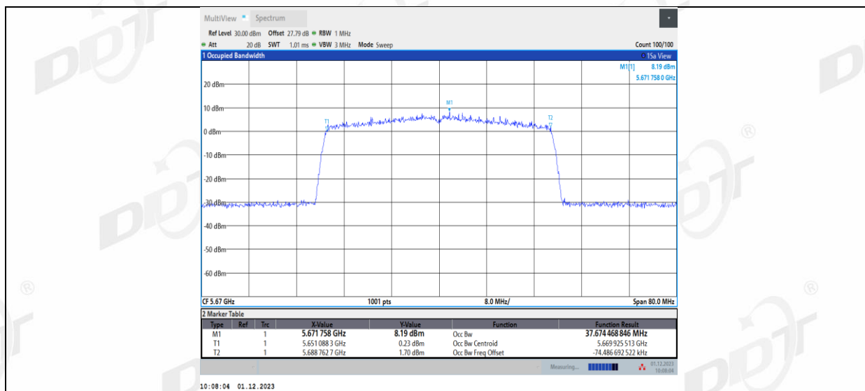
11AX40MIMO_Ant2_5670
