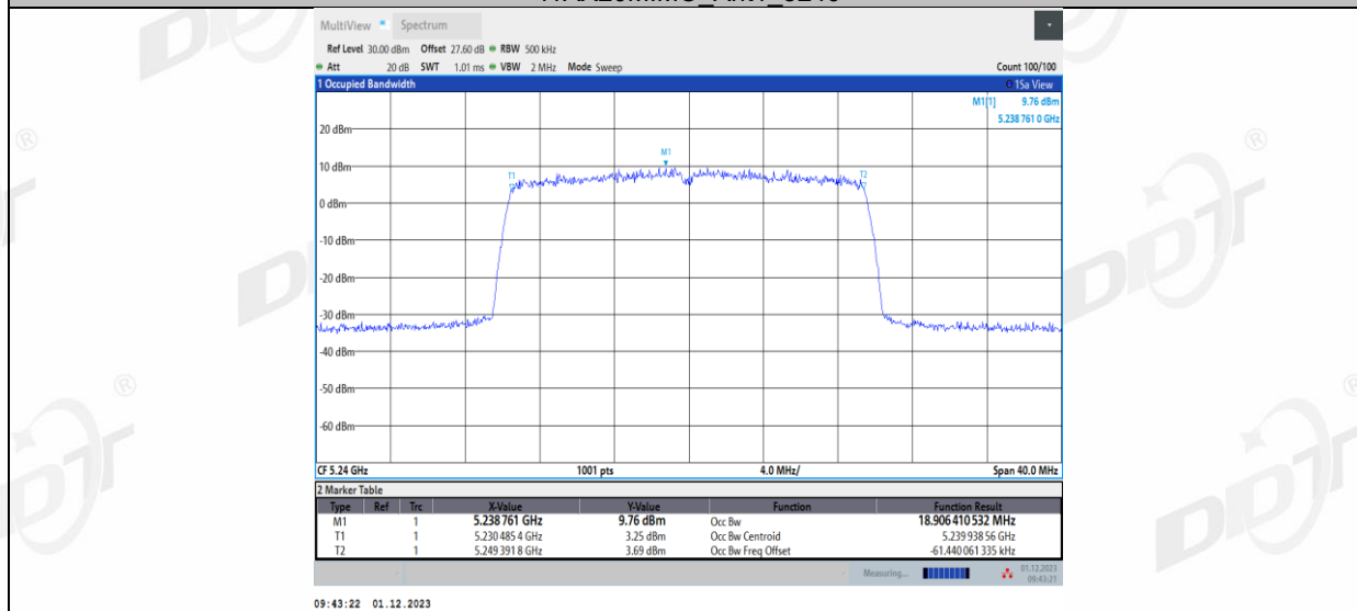
11AX20MIMO_Ant2_5240
