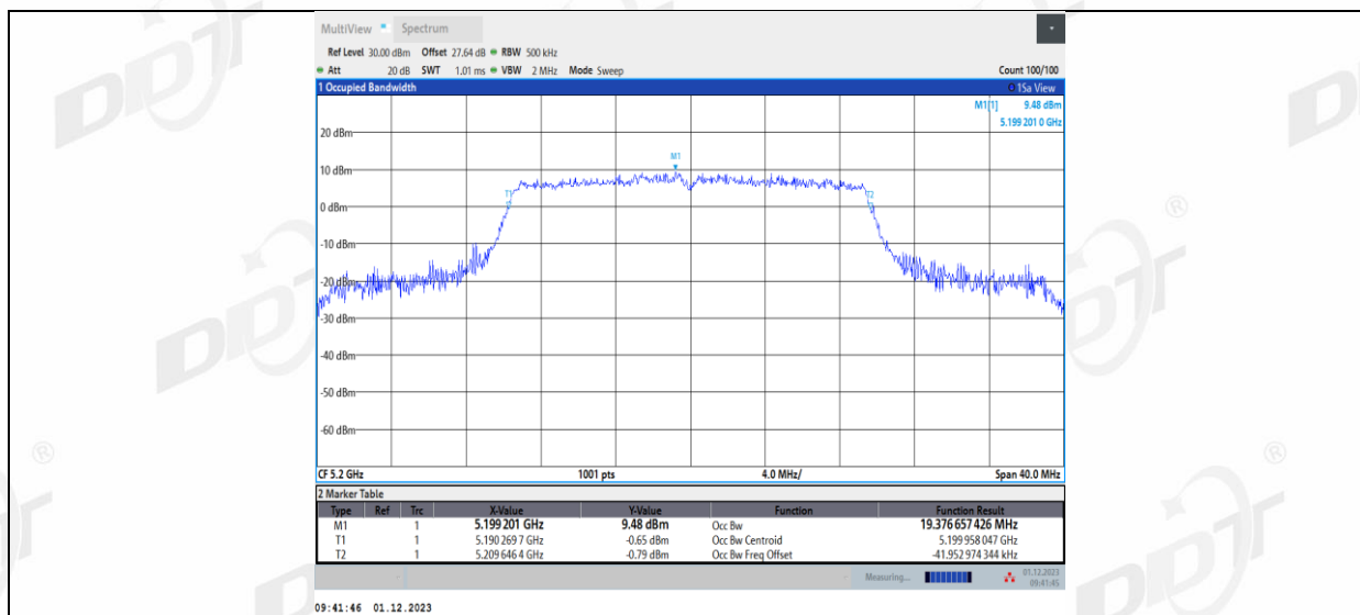
11AX20MIMO_Ant2_5200
