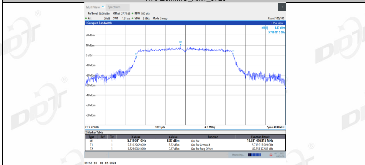
11AX20MIMO_Ant2_5720
