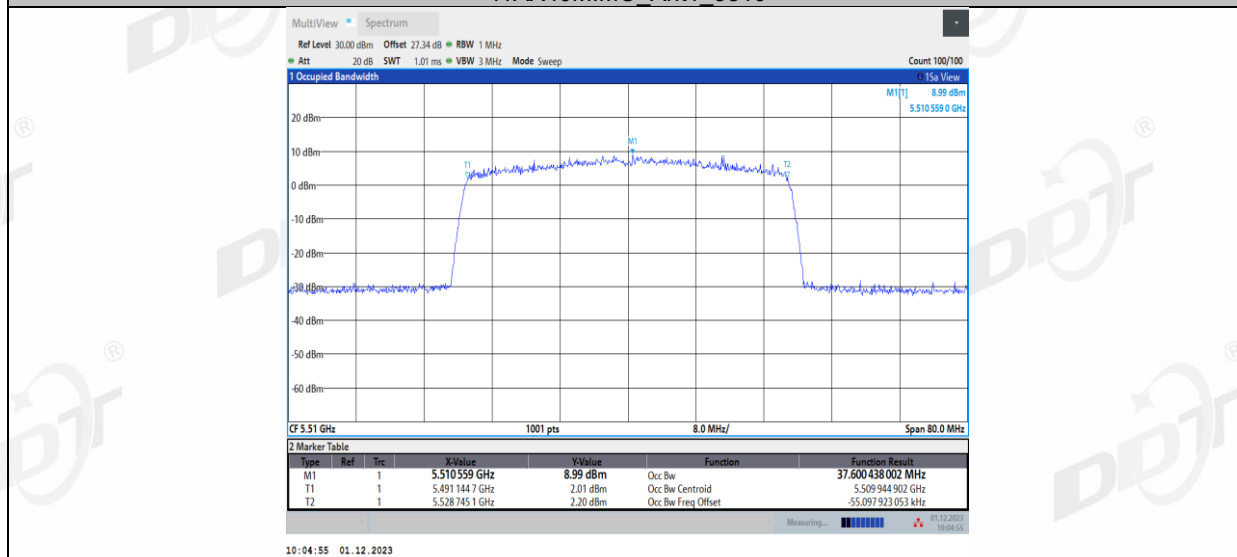
11AX40MIMO_Ant2_5510
