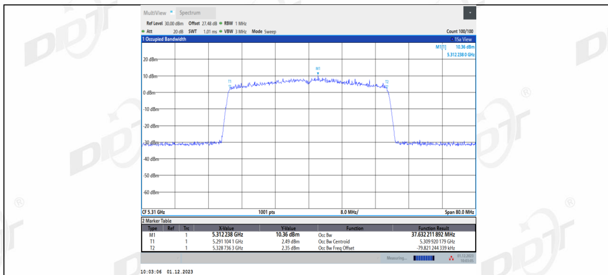
11AX40MIMO_Ant2_5310
