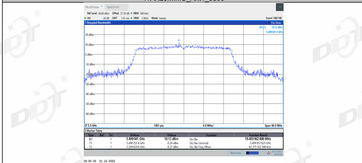
11AX20MIMO_Ant2_5500
