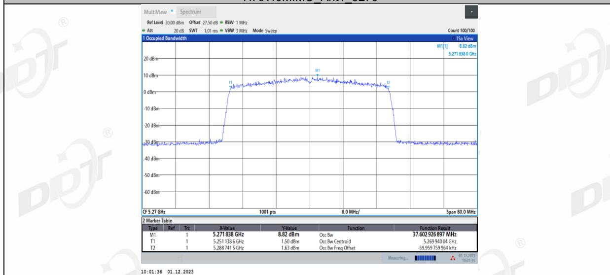
11AX40MIMO_Ant2_5270
