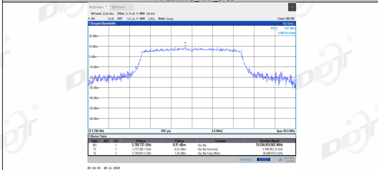
11AX20MIMO_Ant2_5785
