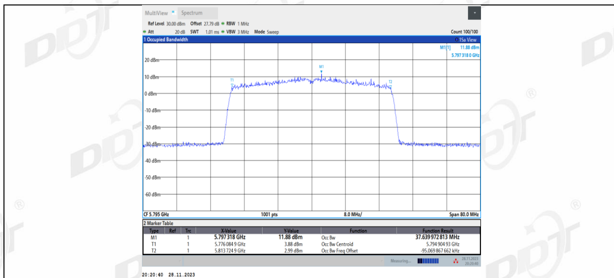
11AX40MIMO_Ant2_5795
