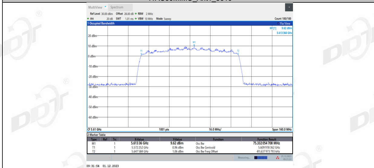
11AC80MIMO_Ant2_5610
