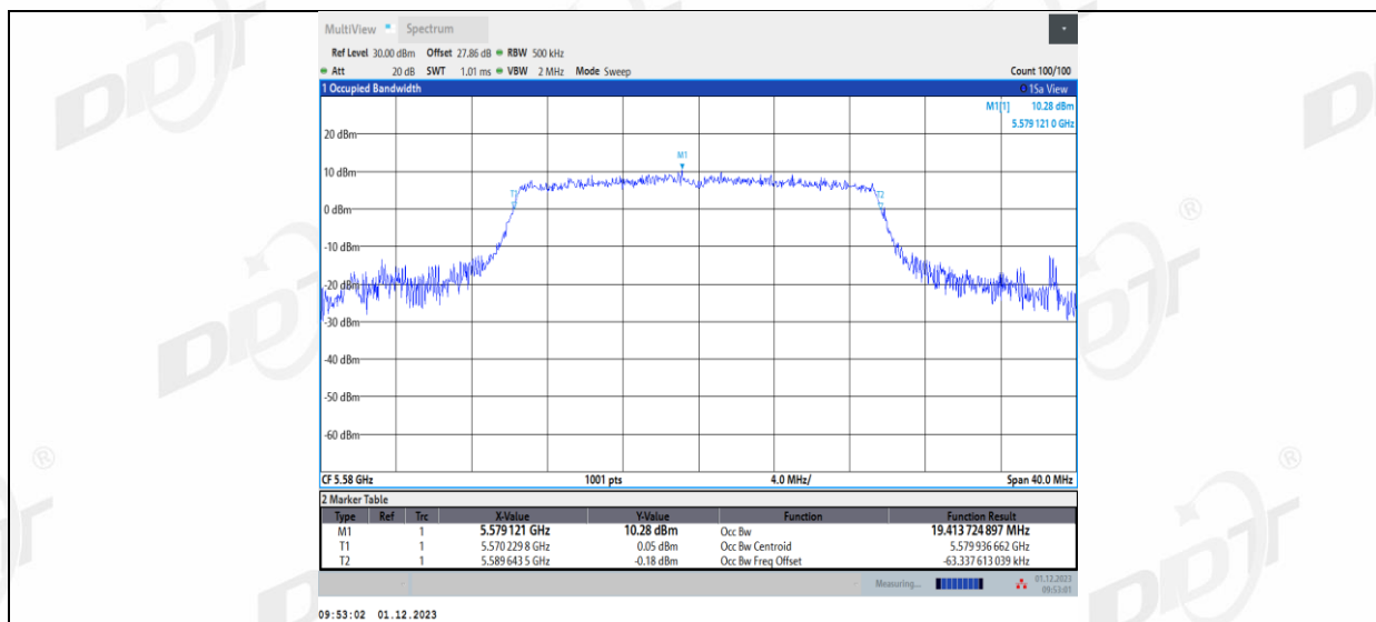
11AX20MIMO_Ant2_5580
