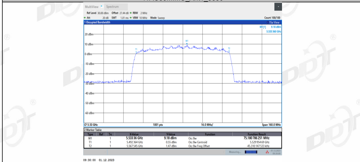
11AC80MIMO_Ant2_5530
