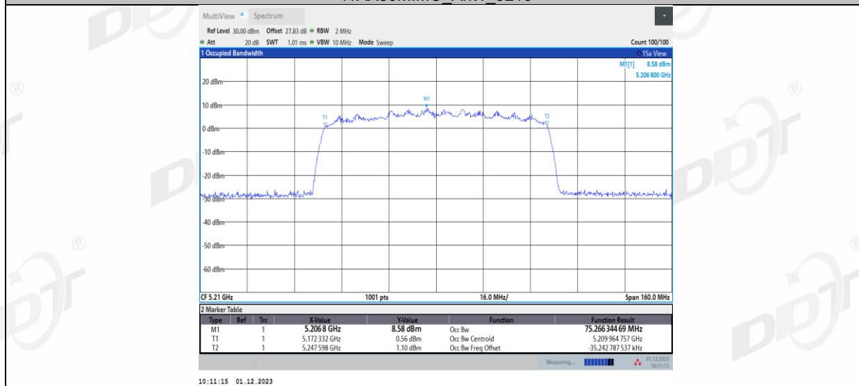
11AX80MIMO_Ant2_5210
