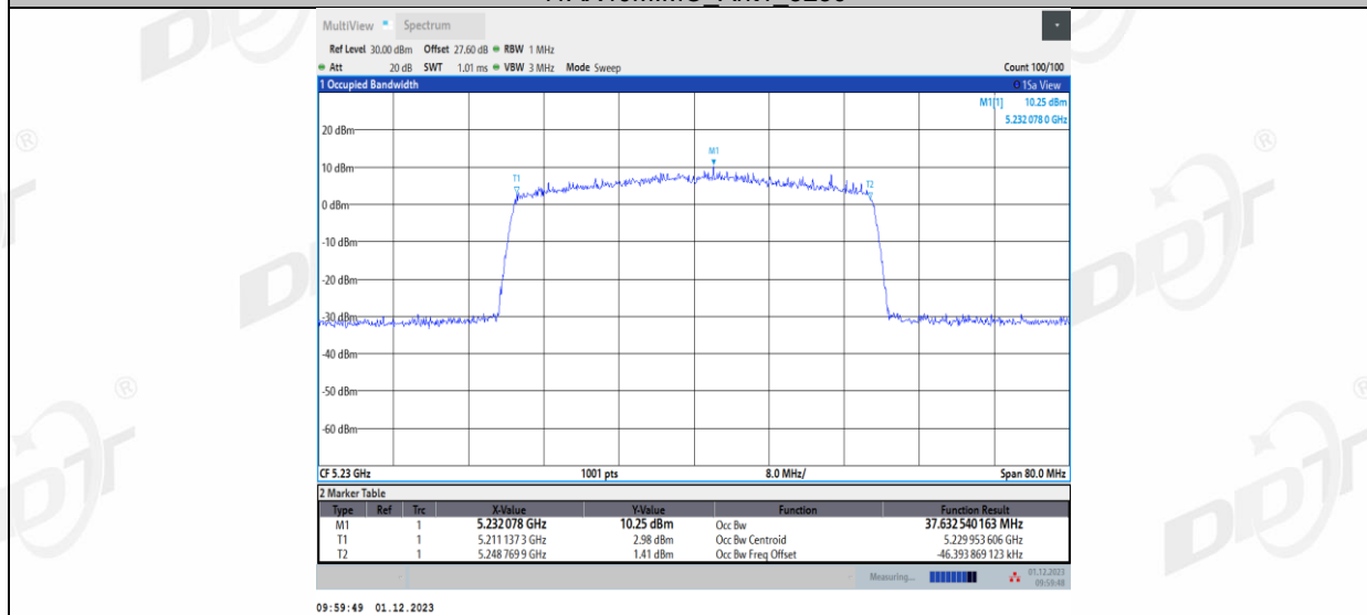
11AX40MIMO_Ant2_5230
