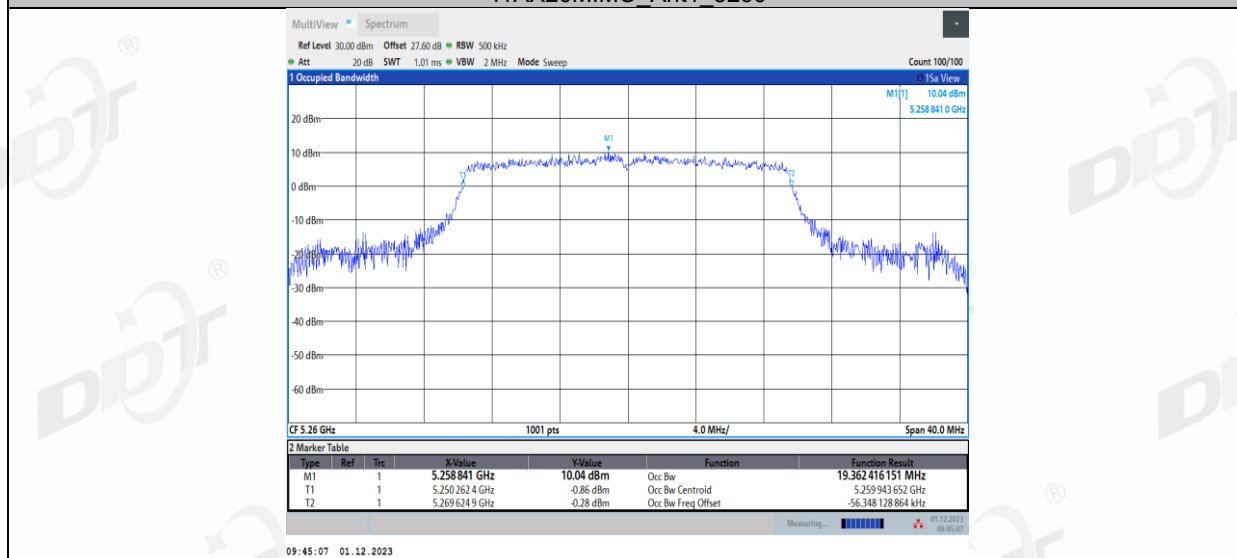
11AX20MIMO_Ant2_5260
