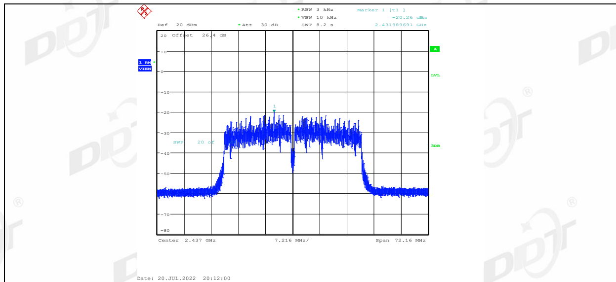
11N40MIMO_Ant2_2437
