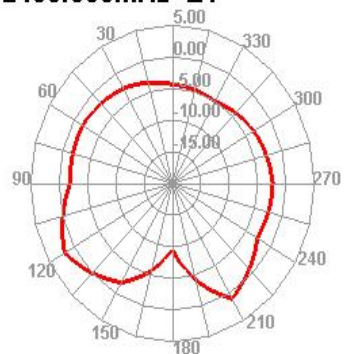
2450.000MHz E1
