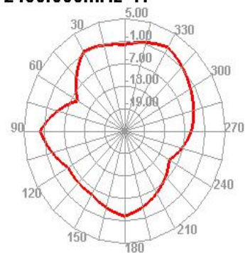
2450.000MHz H
