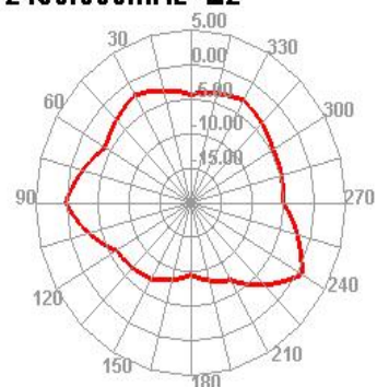
2450.000MHz E2
