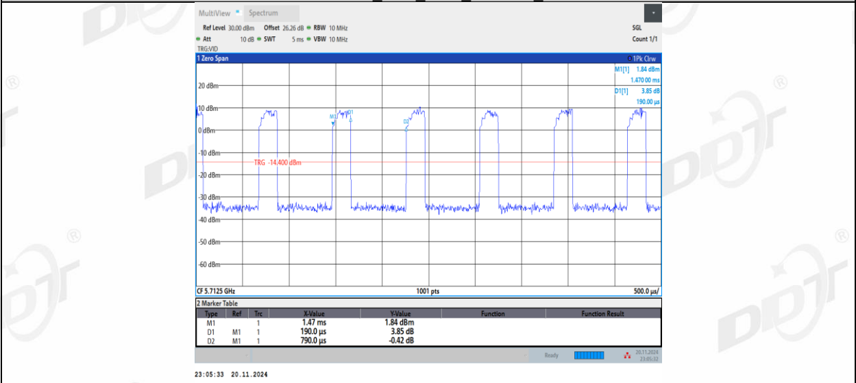
11AX40MIMO_Ant1_5710_106Tone_RU56
