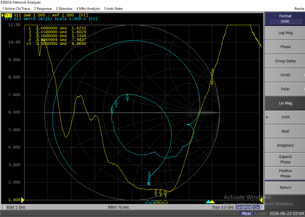
VSWR
