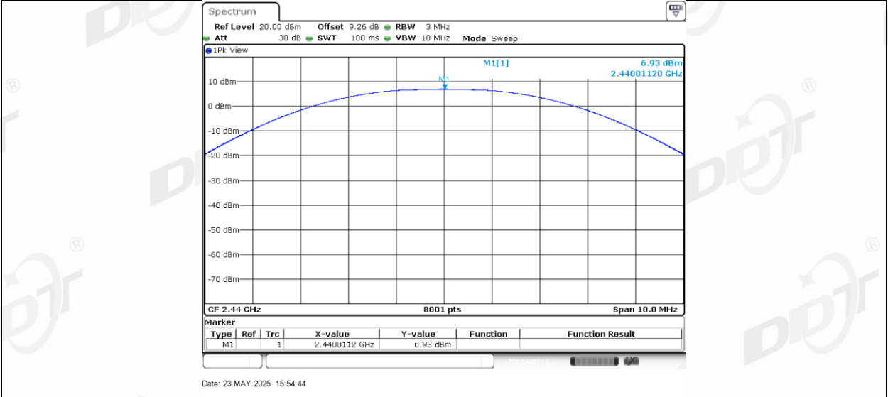
BLE_2M_Right side_2440
