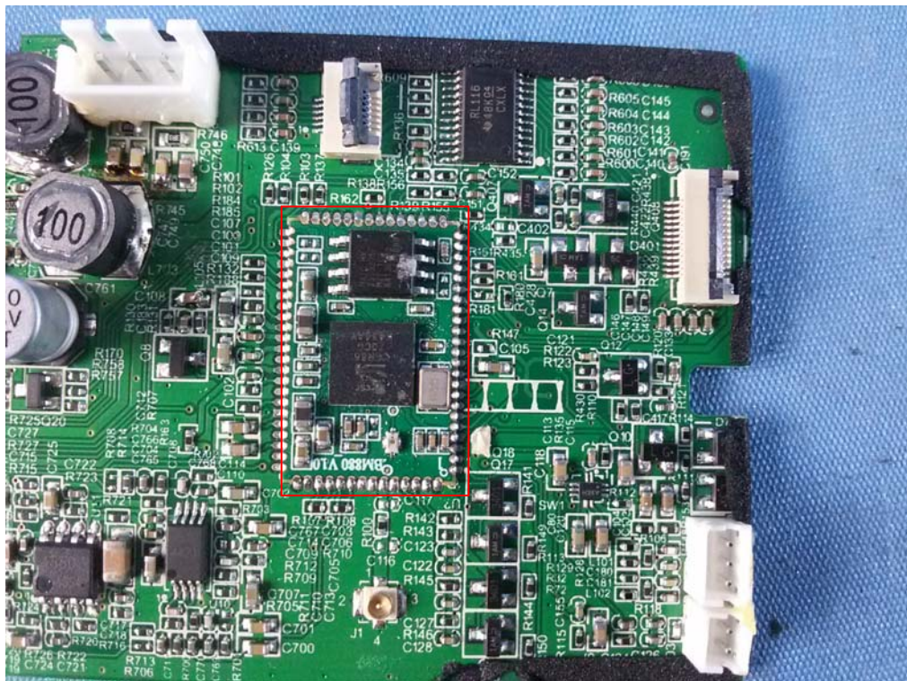
Photo 17 BT Module
