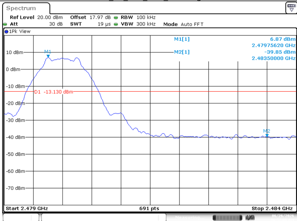
BLE_1M_Ant1_2480_band edge
