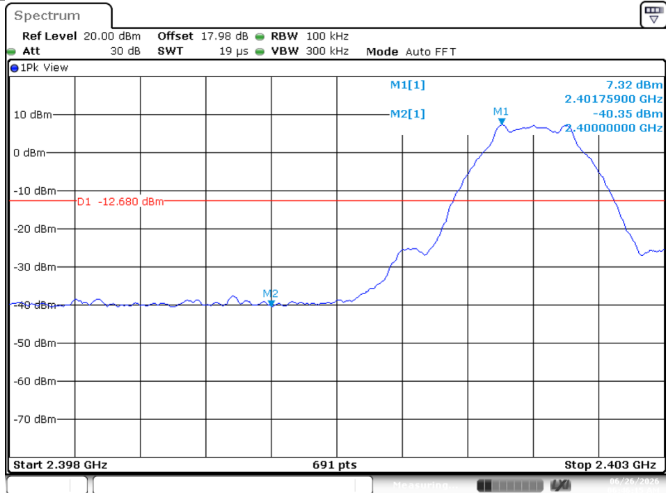
BLE_1M_Ant1_2402_band edge
