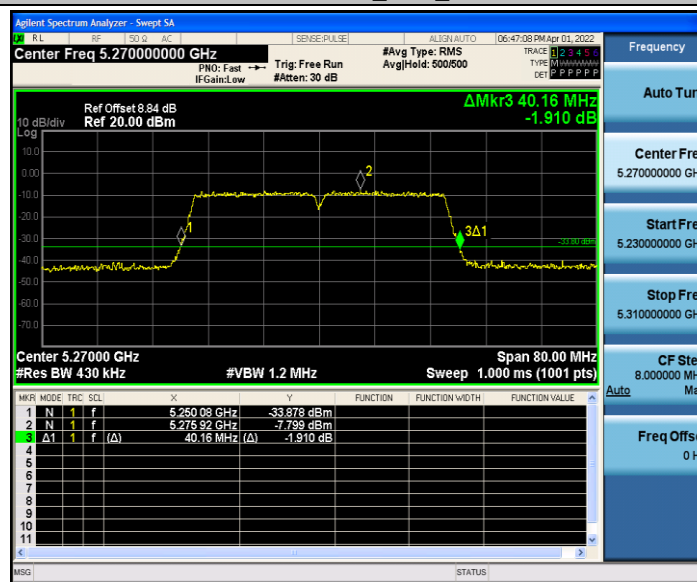
11AC40MIMO_Ant2_5270
