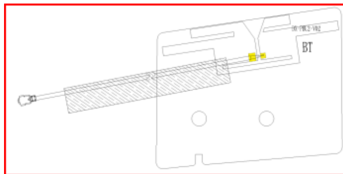
天线外观图
