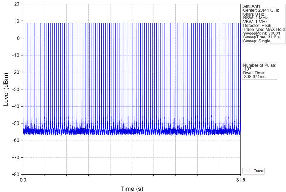
GFSK_DH5_HOPP_Ant1_NTNV
