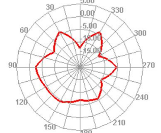
2430.000MHz E2
