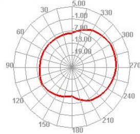
2450.000MHz H
