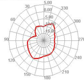
2500.000MHz E1
