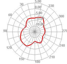
2450.000MHz E1
