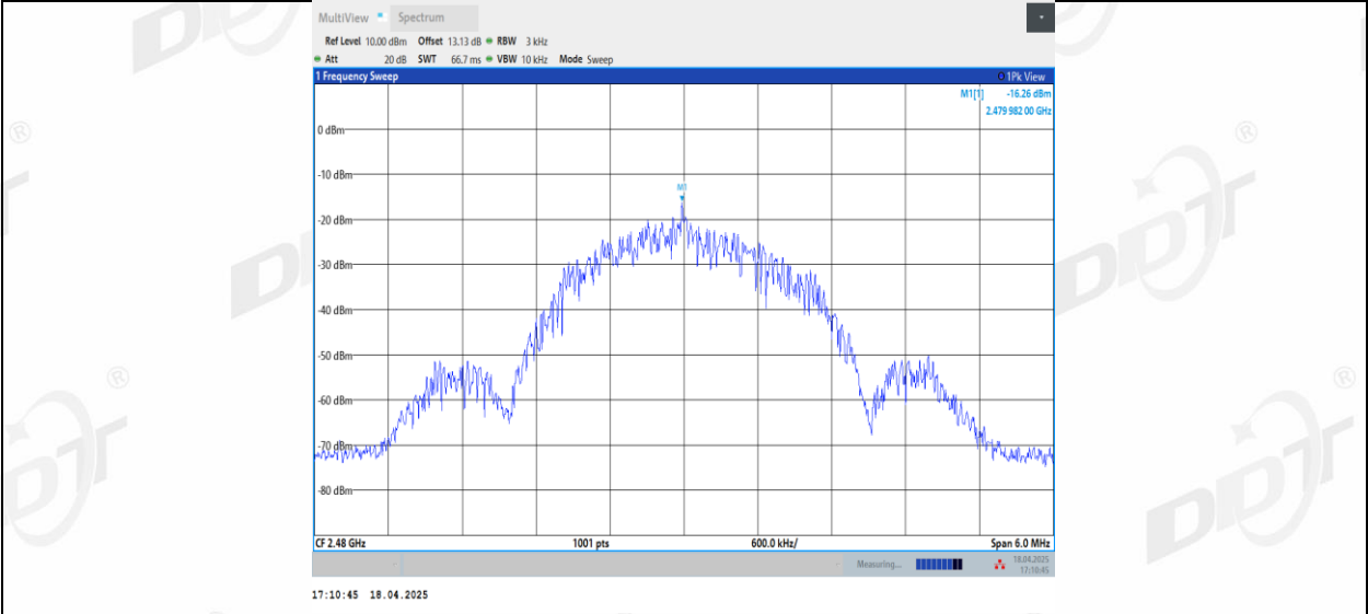
BLE_2M_Ant1_2480
