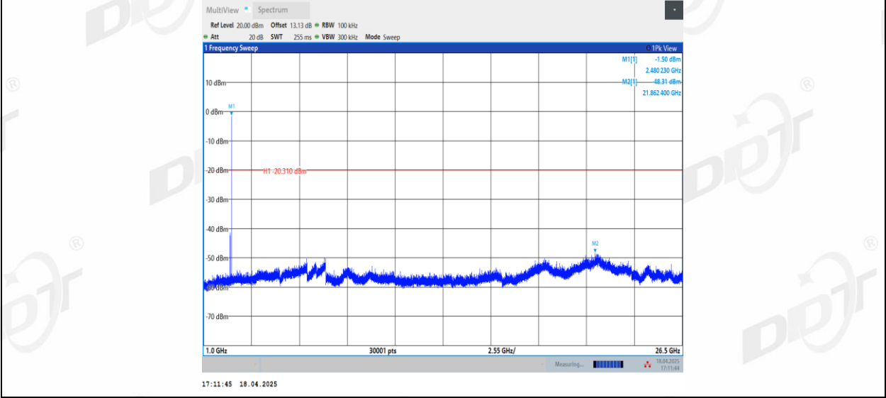
BLE_2M_Ant1_2480_1000~26500
