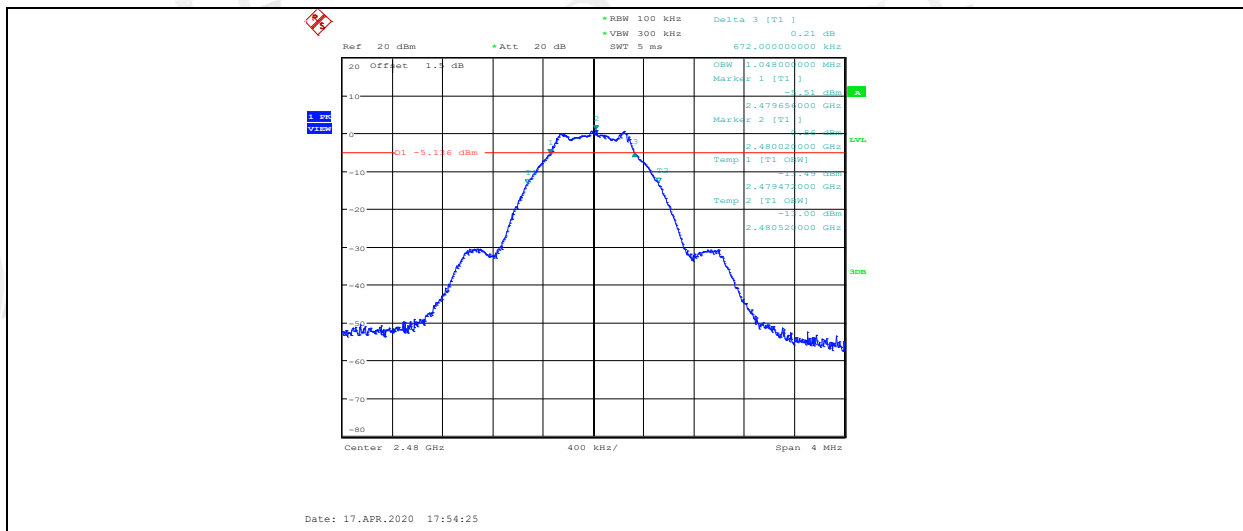
GFSK 2M
