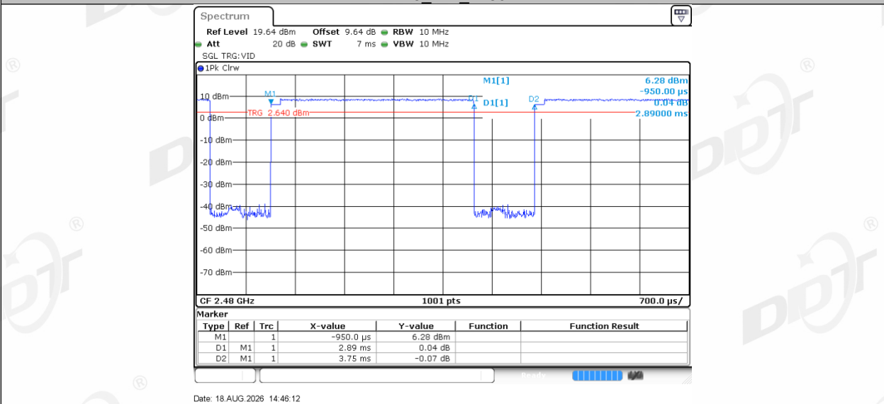
2DH5_Right_2480
