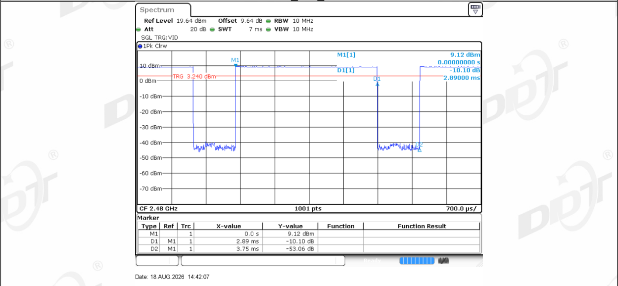
DH5 Right 2480
