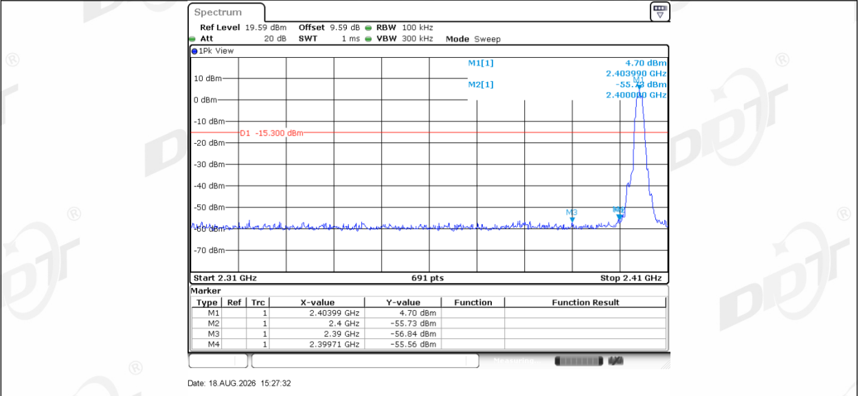
BLE 2M Right Low 2404
