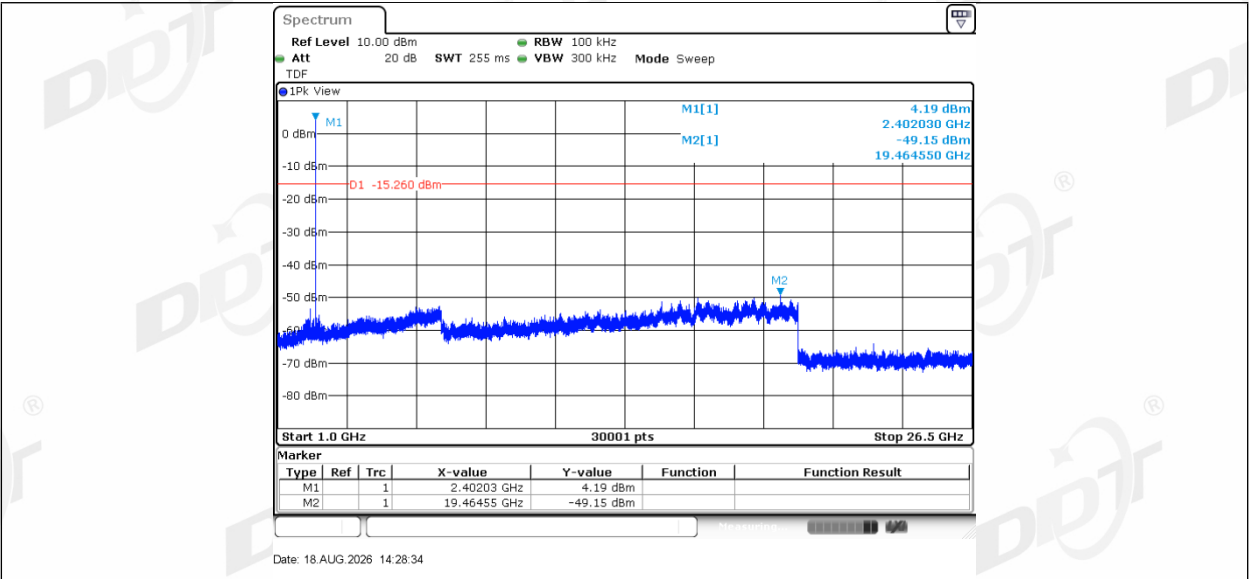
BLE 1M Right 2402 0~Reference
