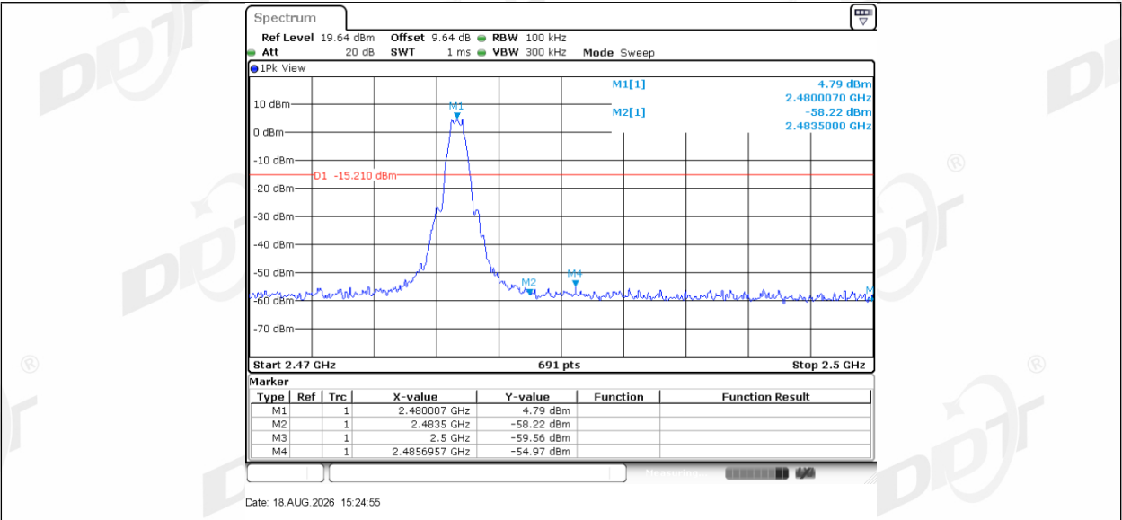
BLE 1M Right High 2480
