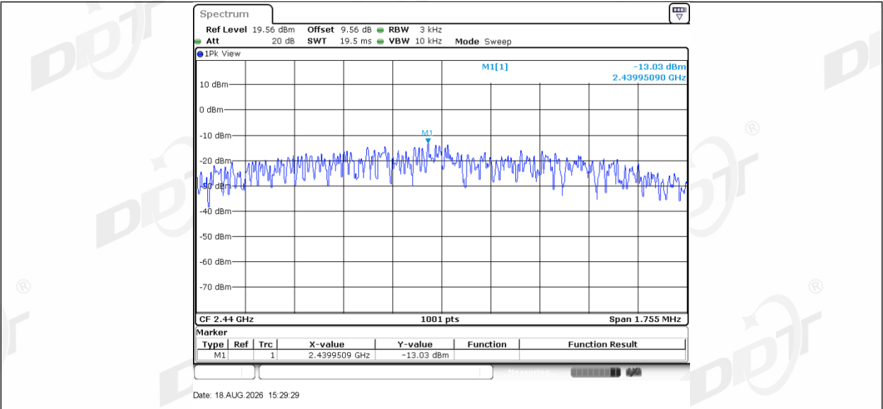
BLE 2M Right 2440
