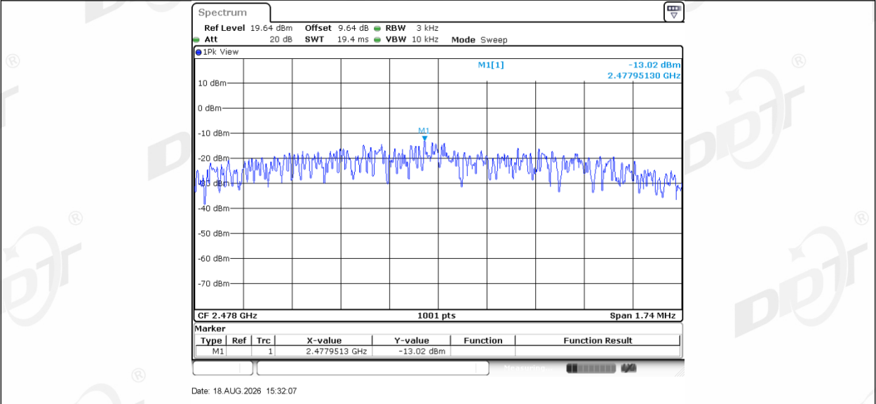
BLE 2M Right 2478
