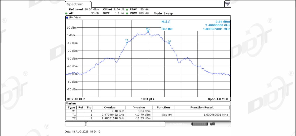
BLE 1M Right 2480
