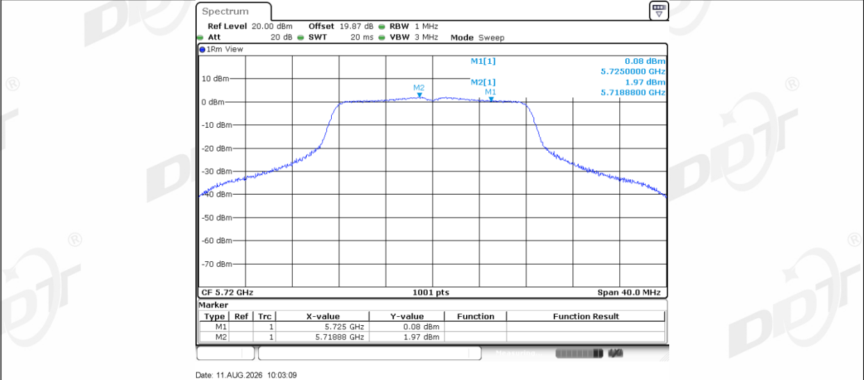
11A_Ant2_5720_UNII-2C
