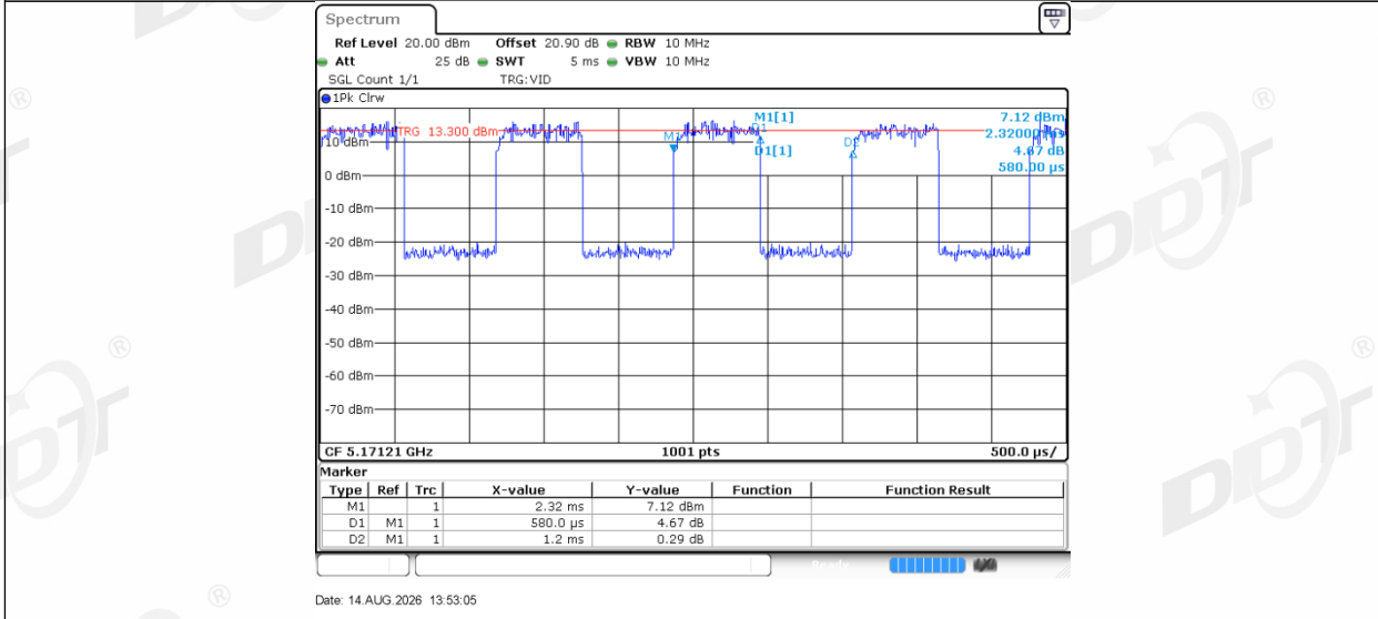
11AX20MIMO_Ant1_5180_52Tone_RU37
