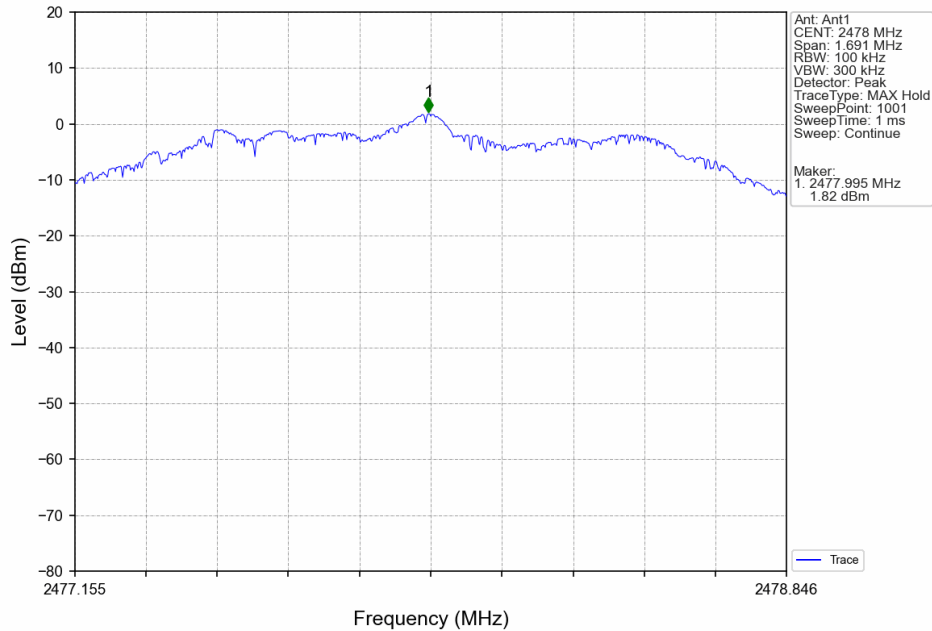
2.4G_HCH_2478MHz_Ant1_NTNV
