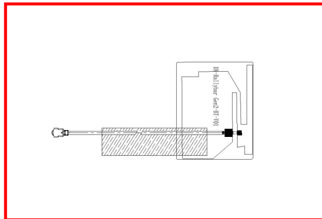
天线外观图
