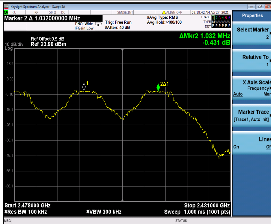
DH5_Ant1_Hop_2480
