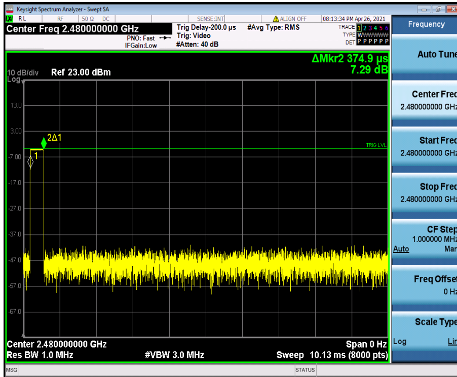
DH1_Ant1_Hop_2480
