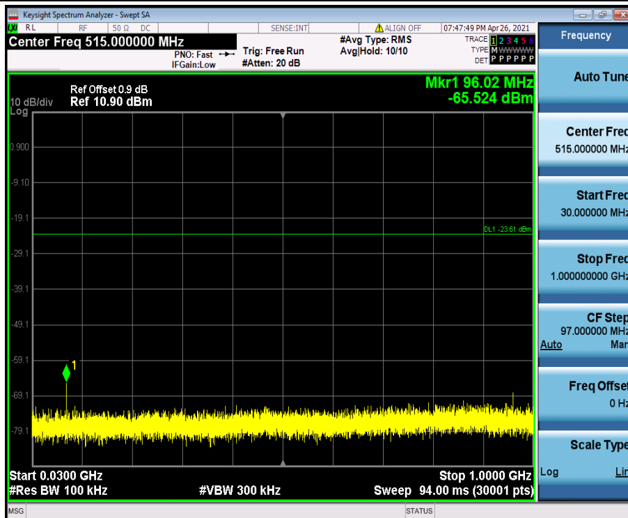
DH5_Ant1_2480_30~1000
