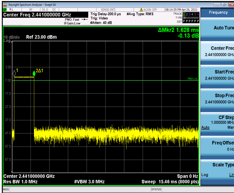
DH3_Ant1_Hop_2441
