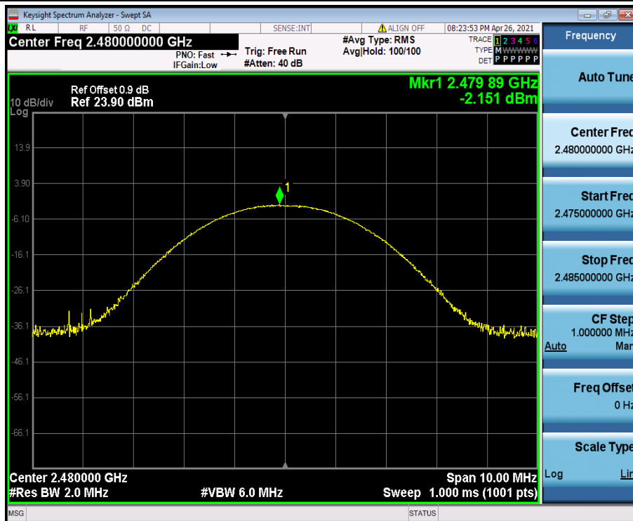
2DH5_Ant1_2480
