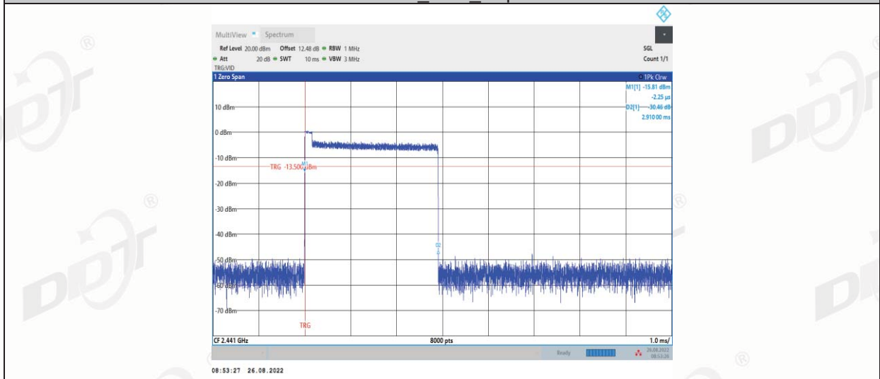
2DH5_Ant1_Hop
