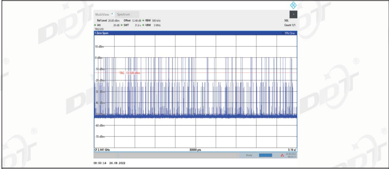
2DH1_Ant1_Hop
