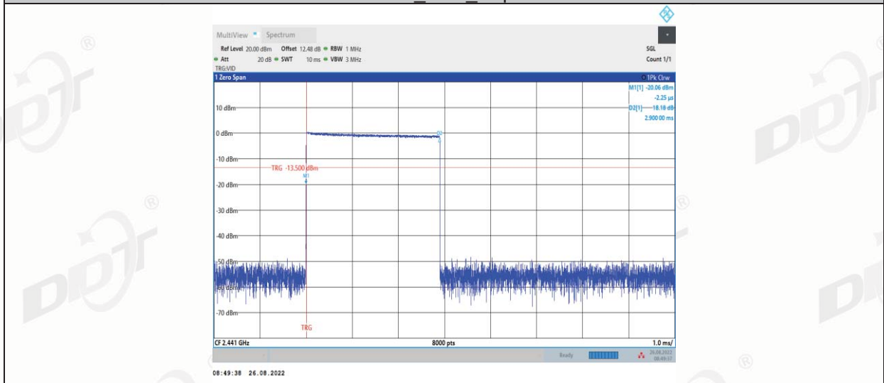
DH5_Ant1_Hop
