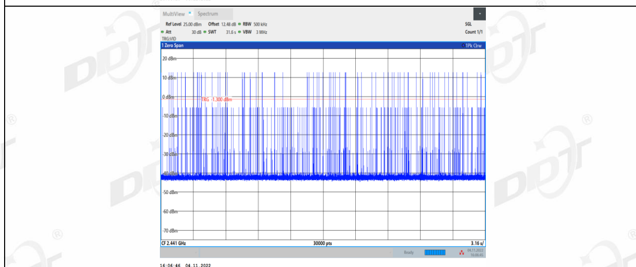
3DH1_Ant1_Hop
