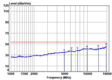
BLE_2M_TX_CH_38_Horizontal-Avg
