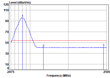
BLE_2M_TX_CH_38_Horizontal-Avg
