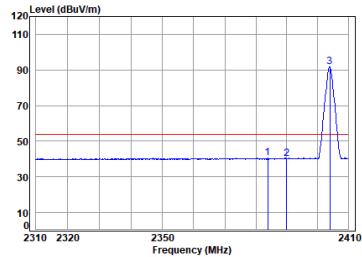
BLE_2M_TX_CH_01_Vertical-Avg
