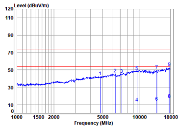
2.4G SRD_2M_TX_CH_01_Horizontal
