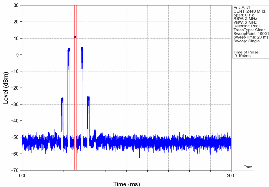
2M_HOPP_Ant1_NTNV
