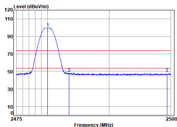
2.4G SRD_1M_TX_CH_39_Horizontal
