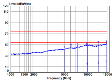
2.4G SRD_1M_TX_CH_39_Horizontal
