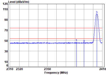
2.4G SRD_2M_TX_CH_01_Horizontal
