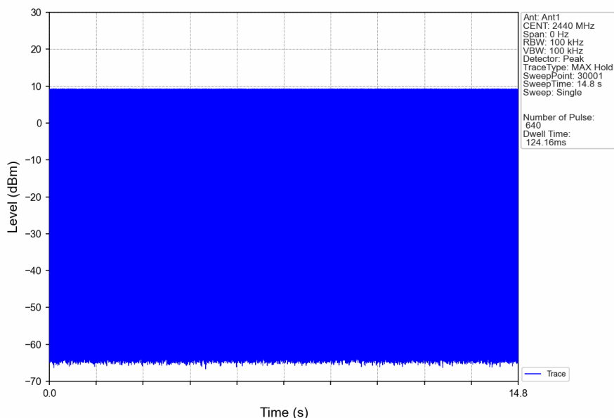
2M_HOPP_Ant1_NTNV
