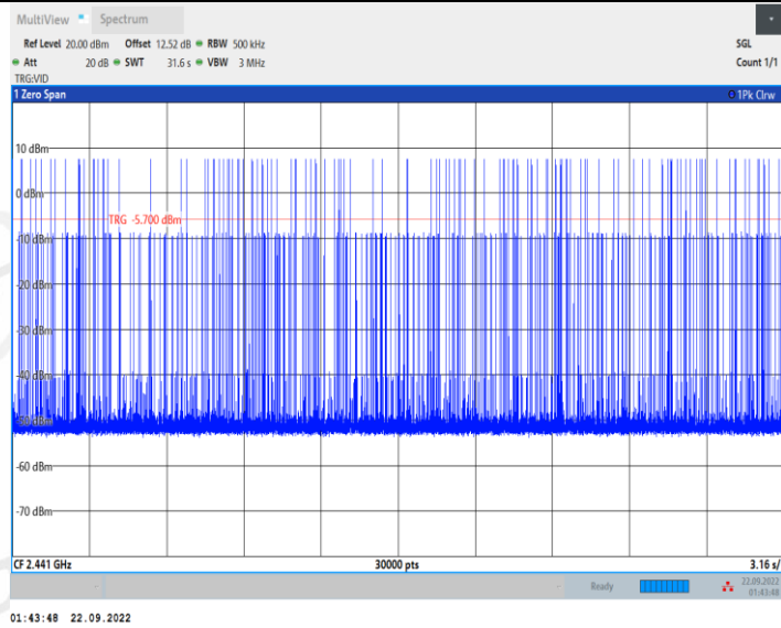
3DH1_Ant1_Hop
