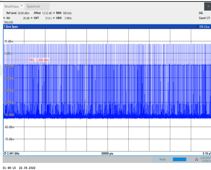
3DH3_Ant1_Hop
