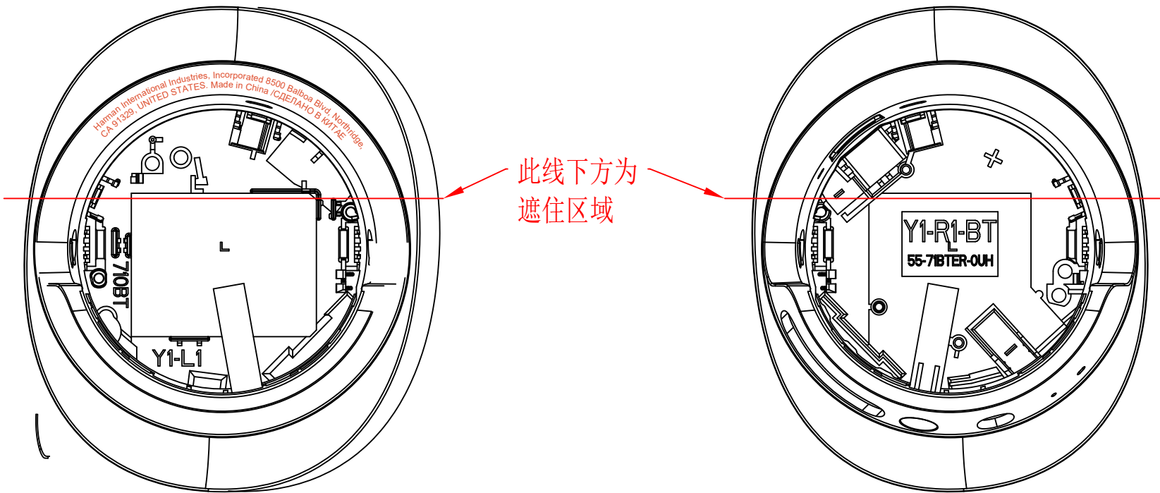
左耳壳
