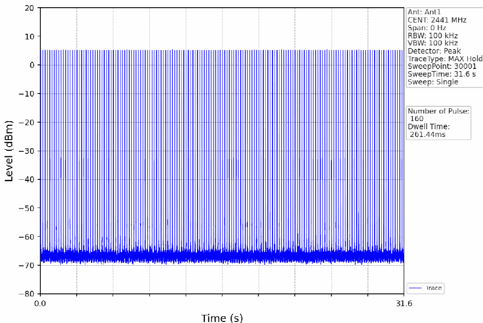
Pi/4DQPSK_2DH3_HOPP_Ant1_NTNV
