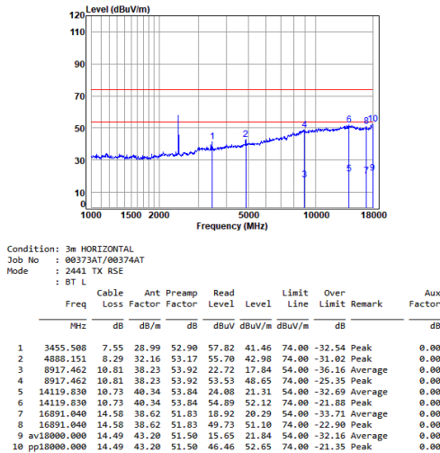
BT_DH5_TX_CH_39_Horizontal
