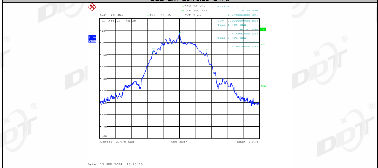
BLE_2M_Left side_2478
