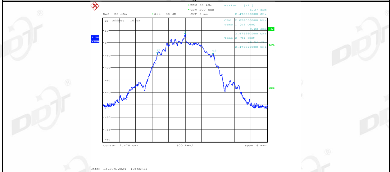
BLE_2M_Left side_2478
