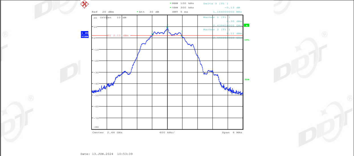
BLE 2M Left side 2440
