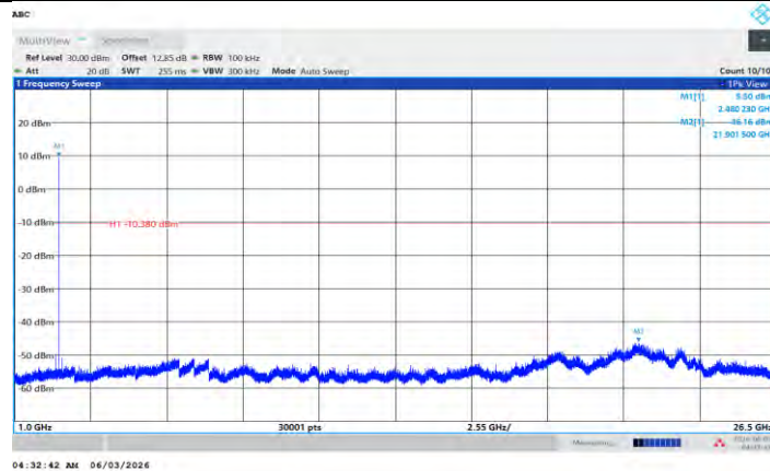
BLE_1M_Ant L_2480_1000-26500
