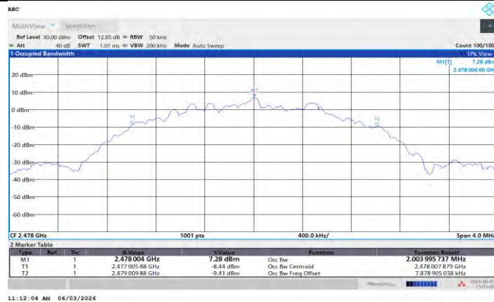
BLE_2M_Ant R_2478
