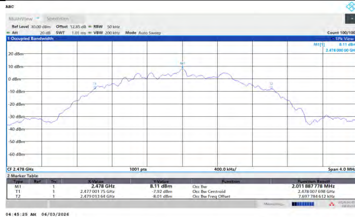
BLE_2M_Ant L_2478
