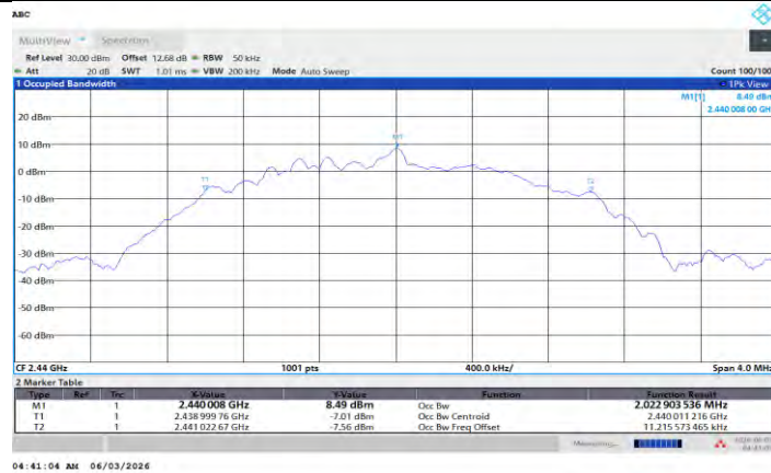
BLE_2M_Ant L_2440
