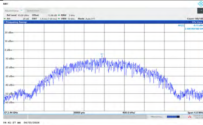
BLE_2M_Ant L_2440
