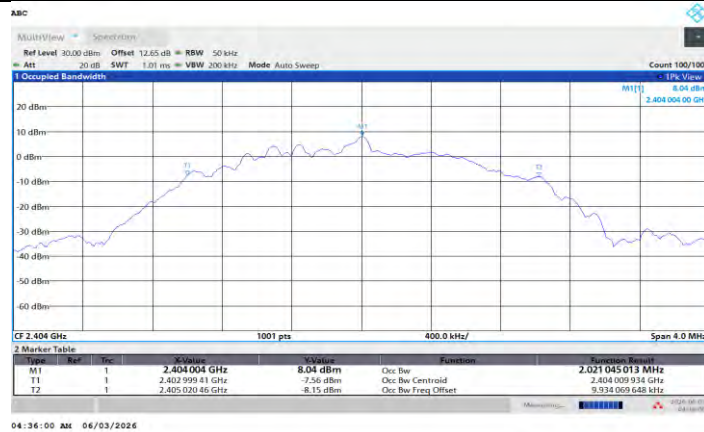
BLE_2M_Ant L_2404
