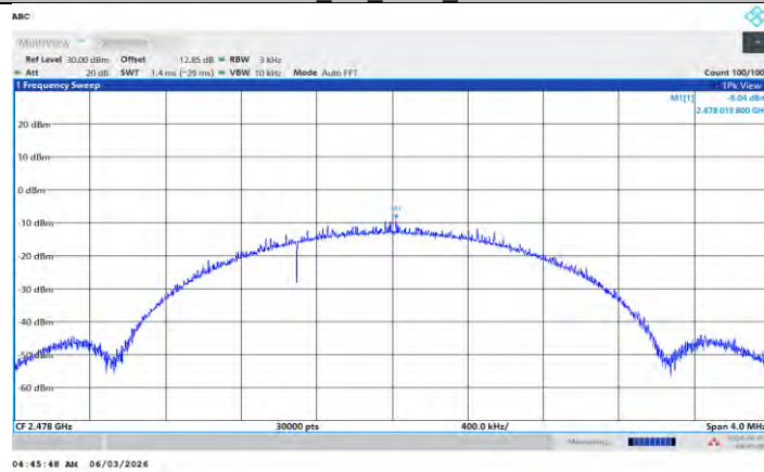
BLE_2M_Ant L_2478
