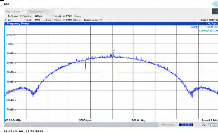
BLE_2M_Ant R_2404
