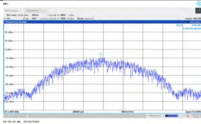
BLE_2M_Ant L_2404
