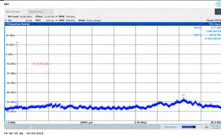
BLE_2M_Ant L_2440_1000-26500
