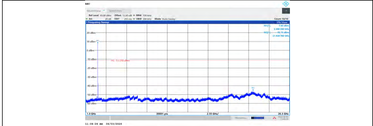
BLE_1M_Ant R_2480_1000-26500
