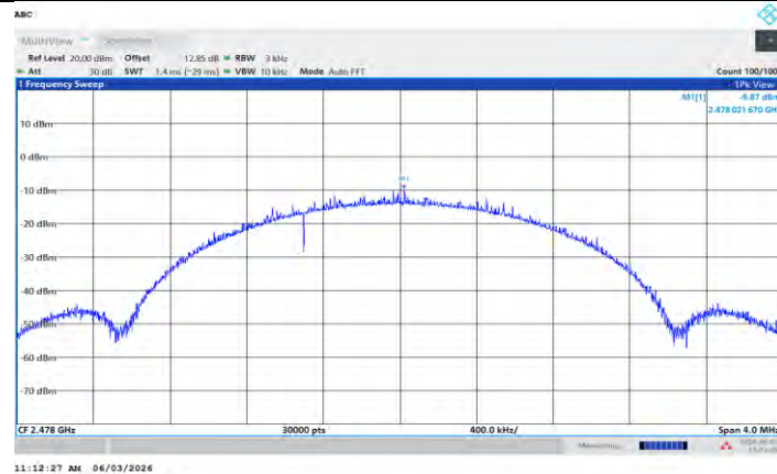
BLE_2M_Ant R_2478
