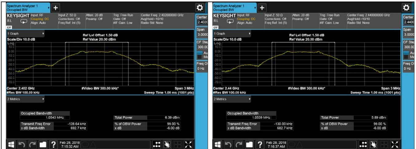
6dB BW –Bluetooth LE 2402MHz
