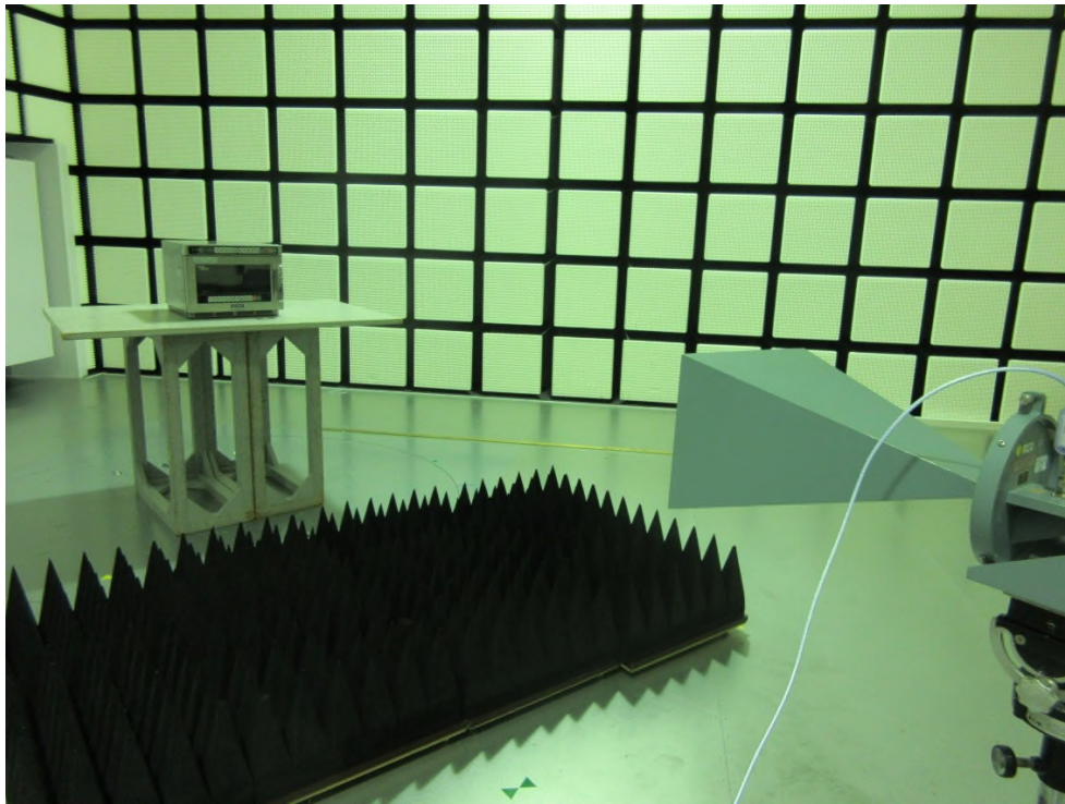
– View(1) –
