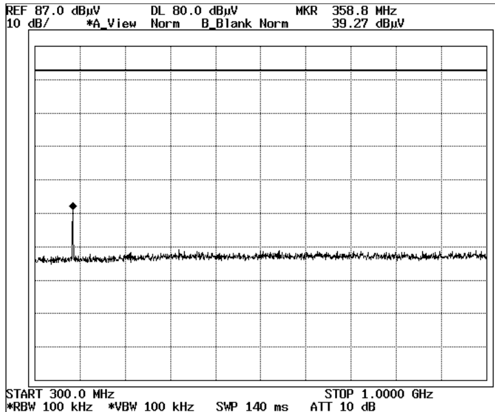
18. ch 40: 2.475GHz: External Attenuator 10dB
