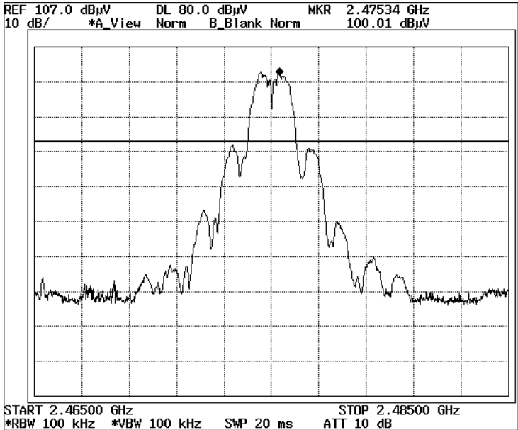
15. ch 40: 2.475GHz: External Attenuator 10dB
