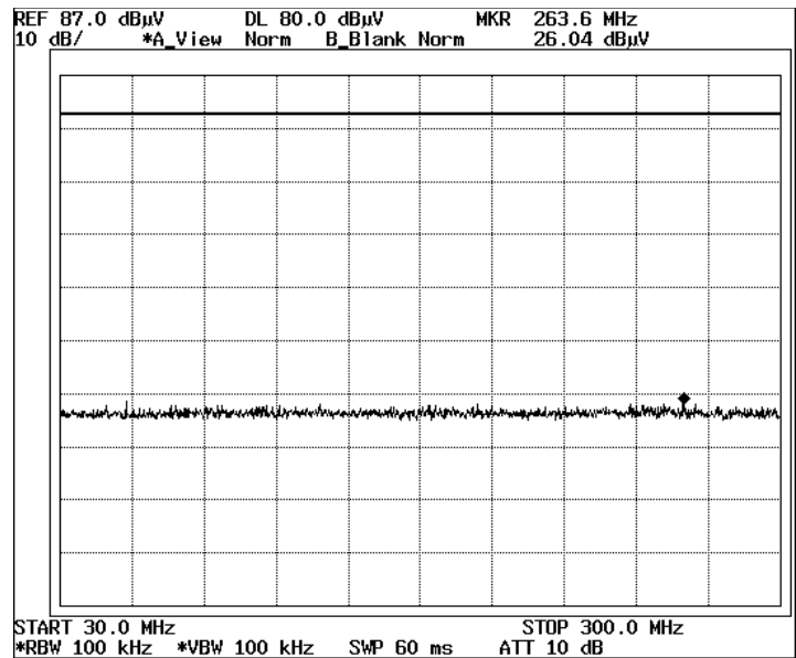
17. ch 40: 2.475GHz: External Attenuator 10dB
