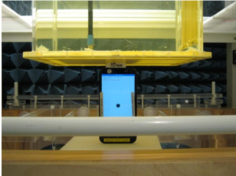
SAR - Top Edge
