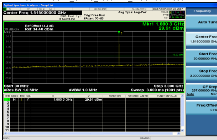
30MHz~3GHz GPRS 1900MHz MidCH661-1880
