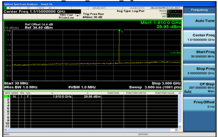
30MHz~3GHz GPRS 1900MHz HighCH810-1909.8
