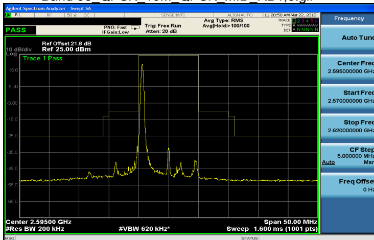
Band 38 QPSK 10M QPSK MID RB1,49.gif
