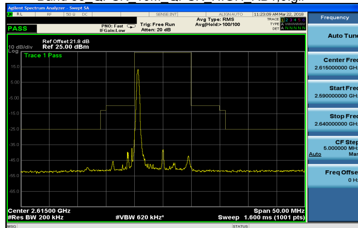
Band 38 QPSK 10M QPSK HIGH RB1,49.gif
