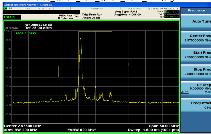
Band 38 QPSK 10M QPSK LOW RB1,49.gif
