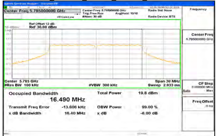
FCC 802.11a 20MHz Chain0 5785MHz
