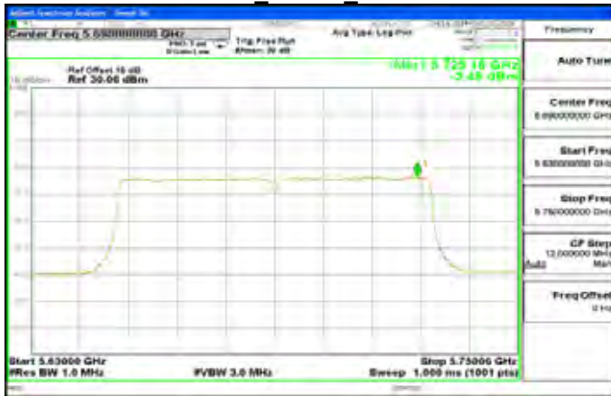
802.11ac 80MHz 5690MHz
