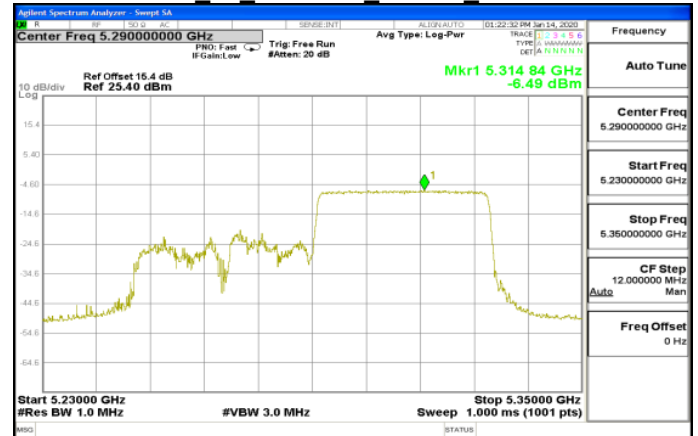
RU 484 66 802.11ax 80MHz 5290MHz
