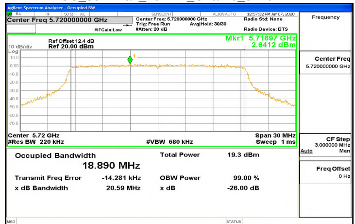
FCC 802.11ax 20MHz_Chain0_5720MHz
