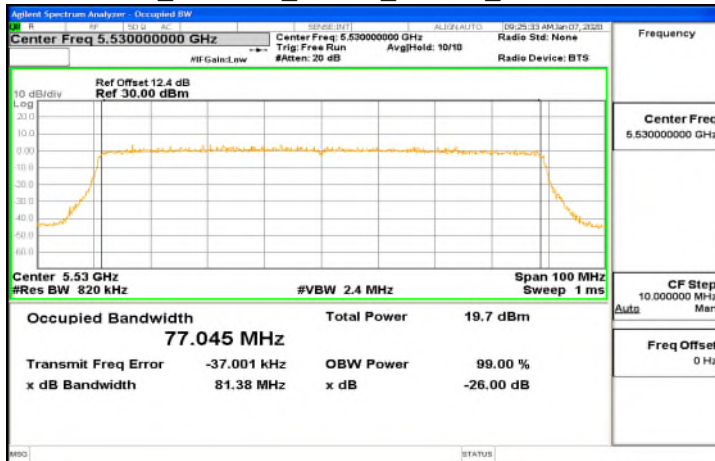
FCC 802.11ax 80MHz Chain1_5530MHz
