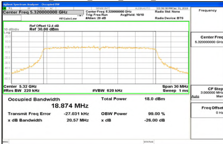
FCC 802.11ax 20MHz Chain1_5320MHz
