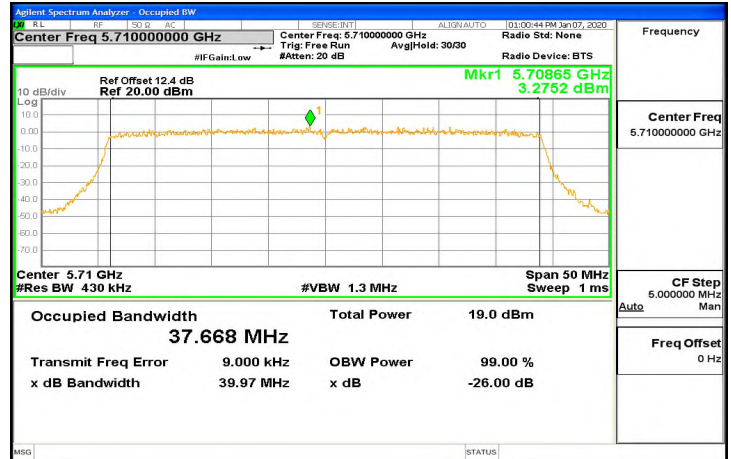
FCC 802.11ax 40MHz Chain0 5710MHz
