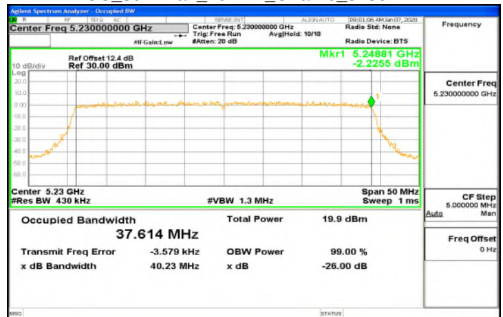
FCC 802.11ax 40MHz Chain0 5230MHz
