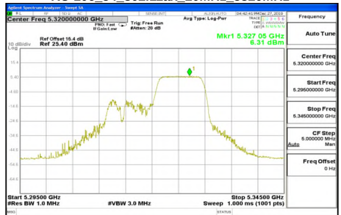
RU 106_54_802.11ax_20MHz_5320MHz
