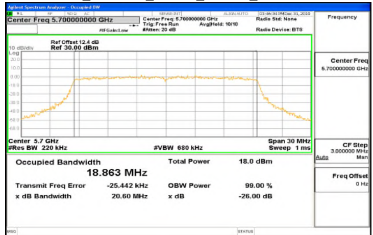
FCC 802.11ax 20MHz Chain1_5700MHz
