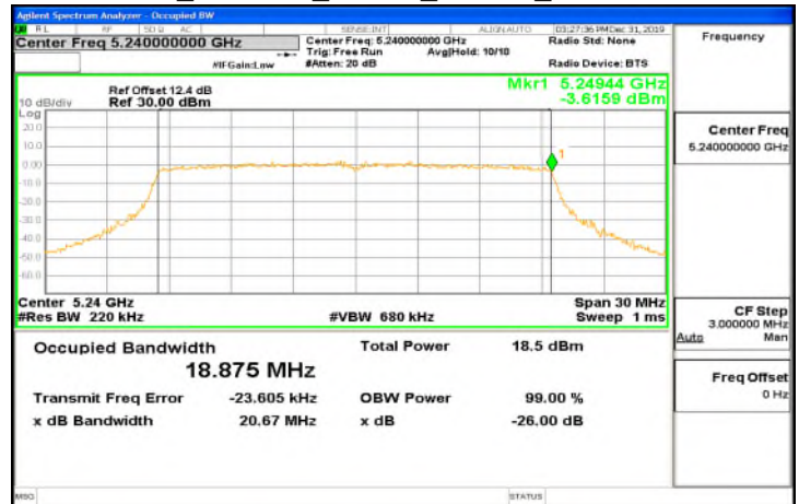
FCC 802.11ax 20MHz Chain1 5240MHz
