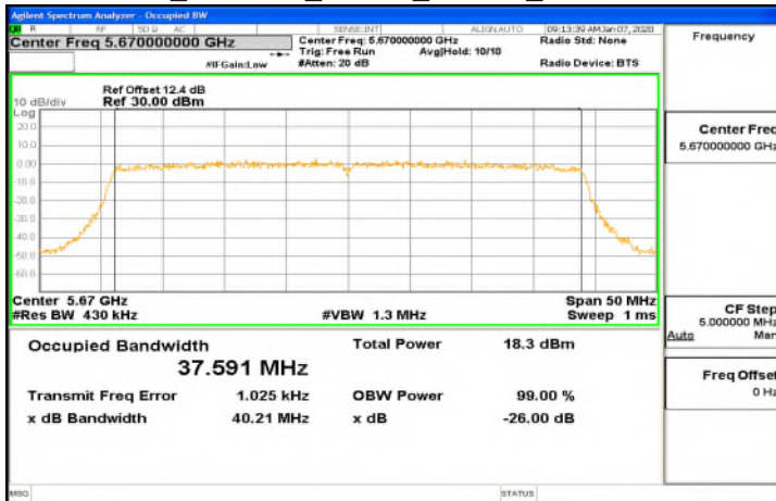
FCC 802.11ax 40MHz Chain1 5670MHz
