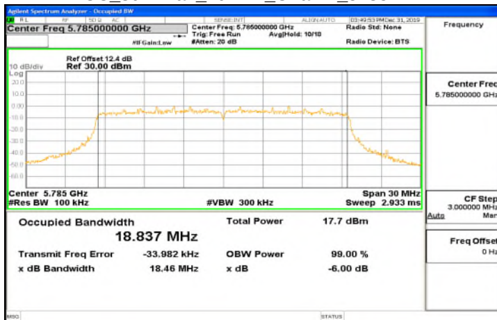
FCC 802.11ax 20MHz Chain1 5785MHz
