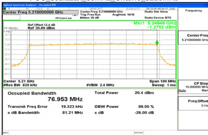
FCC 802.11ax 80MHz Chain0_5210MHz
